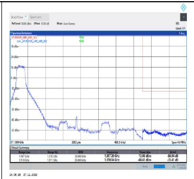
Band2_3MHz_QPSK_19185_1RB#0
