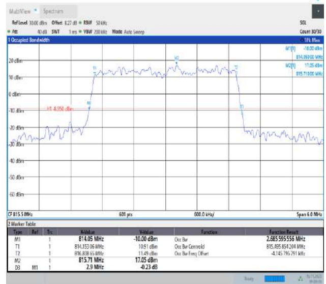
26(814-824)-3MHz-QPSK-26705-15RB#0-PASS
