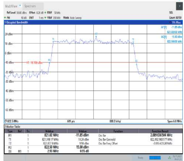
26(814-824)-3MHz-QPSK-26775-15RB#0-PASS
