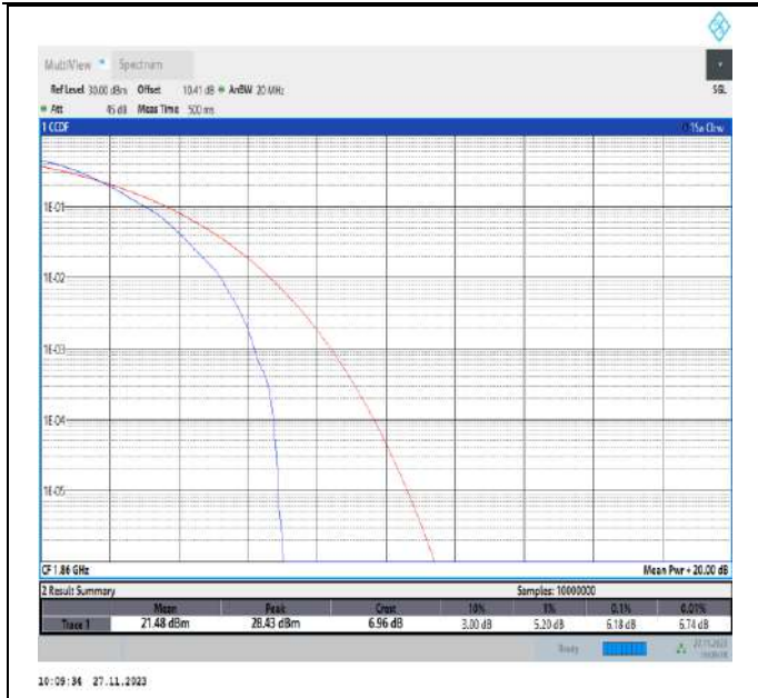
Band2-20MHz-64QAM-18700-1RB#0-PASS
