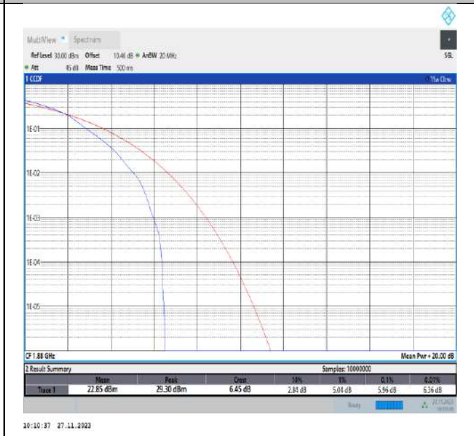
Band2-20MHz-16QAM-18900-1RB#0-PASS
