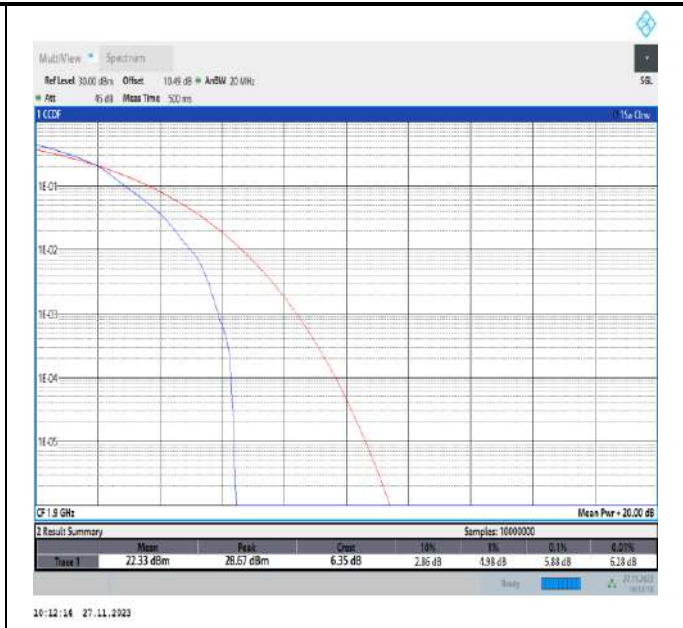
Band2-20MHz-16QAM-19100-1RB#0-PASS
