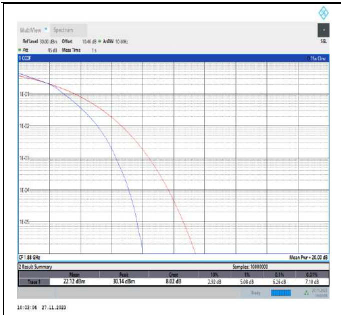
Band2-10MHz-16QAM-18900-50RB#0-PASS
