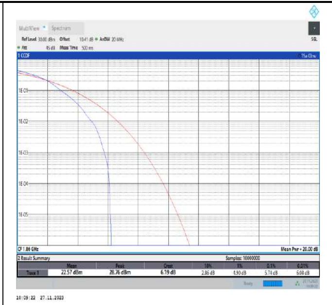
Band2-20MHz-16QAM-18700-1RB#0-PASS
