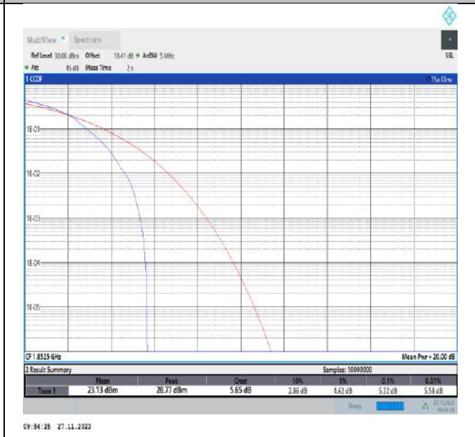
Band2-5MHz-16QAM-18625-1RB#0-PASS
