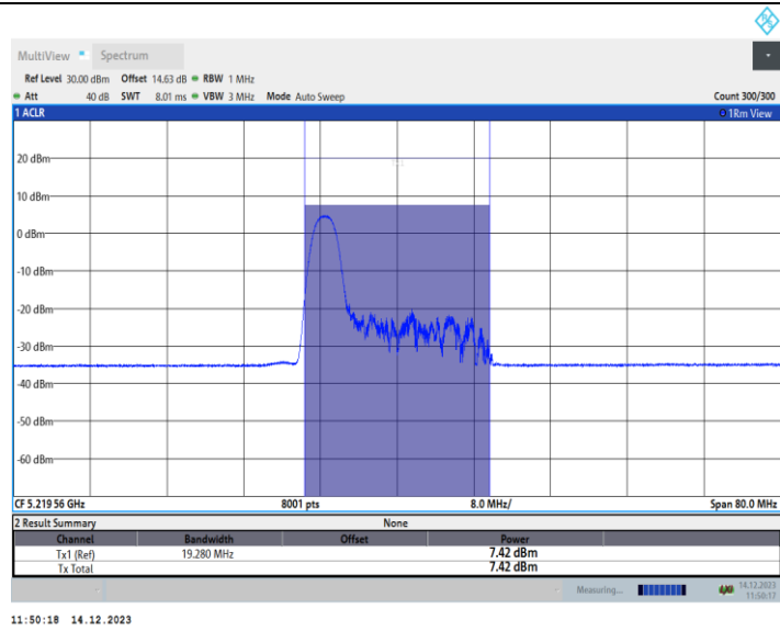
11AX40MIMO_Ant1_5230_52Tone_RU37
