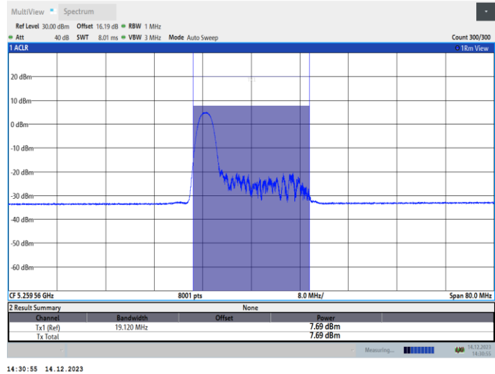
11AX40MIMO_Ant2_5270_52Tone_RU37
