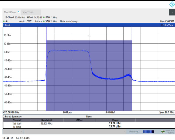
11AX40MIMO_Ant2_5590_26Tone_RU0
