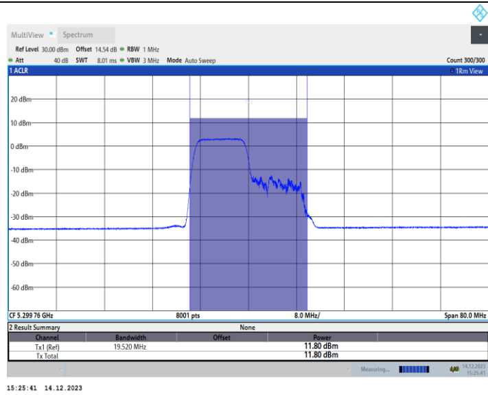
11AX40MIMO_Ant1_5310_242Tone_RU61
