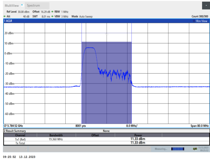
11AX40MIMO_Ant2_5795_106Tone_RU53
