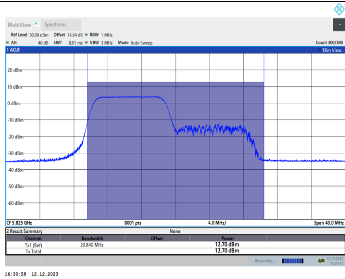
11AX20MIMO_Ant2_5825_26Tone_RU0
