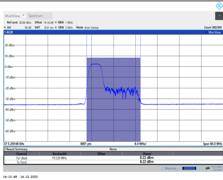
11AX40MIMO_Ant1_5270_106Tone_RU53
