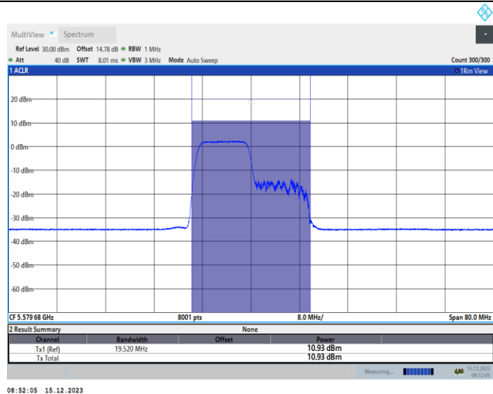
11AX40MIMO_Ant2_5590_242Tone_RU61
