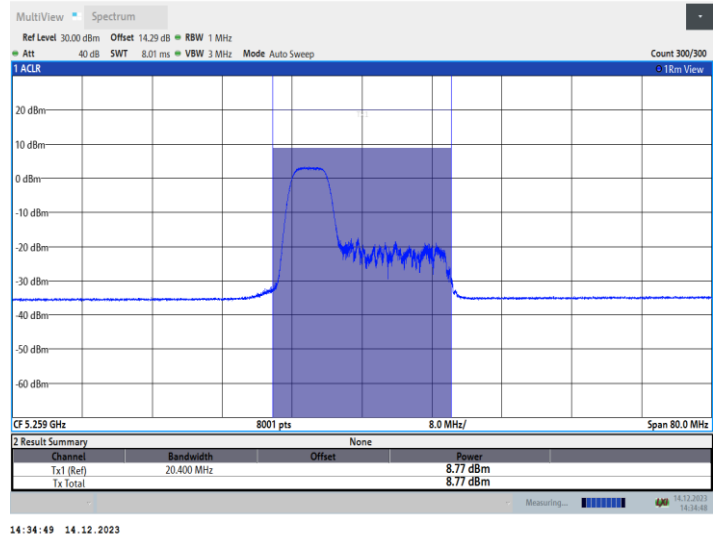
11AX40MIMO_Ant2_5270_106Tone_RU53
