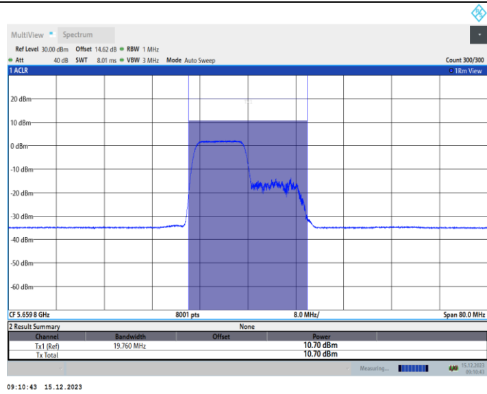
11AX40MIMO_Ant1_5670_242Tone_RU61
