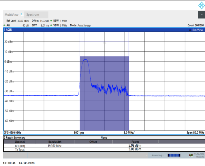
11AX40MIMO_Ant1_5510_52Tone_RU37
