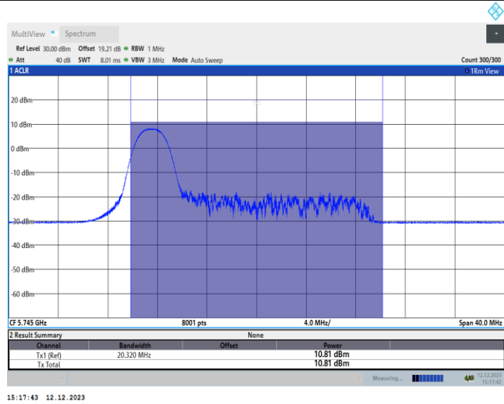
11AX20MIMO_Ant2_5745_52Tone_RU37
