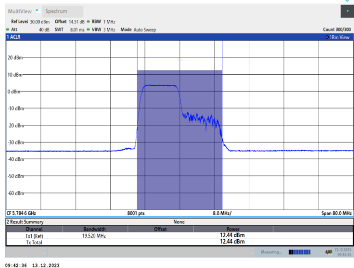
11AX40MIMO_Ant2_5795_242Tone_RU61
