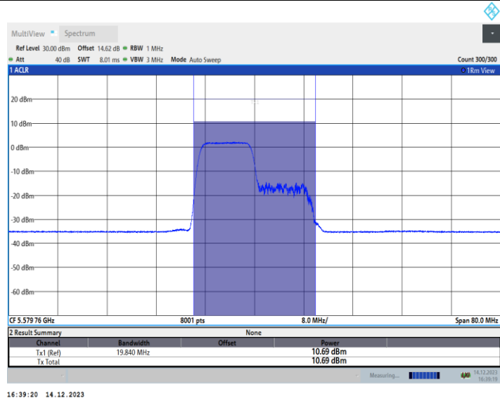
11AX40MIMO_Ant1_5590_242Tone_RU61
