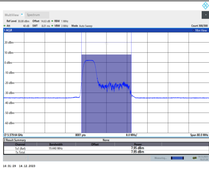
11AX40MIMO_Ant1_5590_106Tone_RU53
