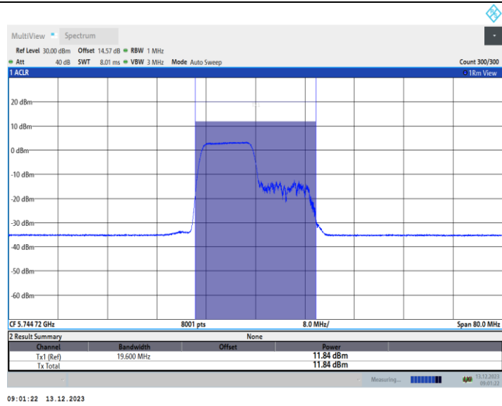
11AX40MIMO_Ant2_5755_242Tone_RU61
