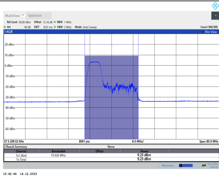
11AX40MIMO_Ant2_5310_106Tone_RU53
