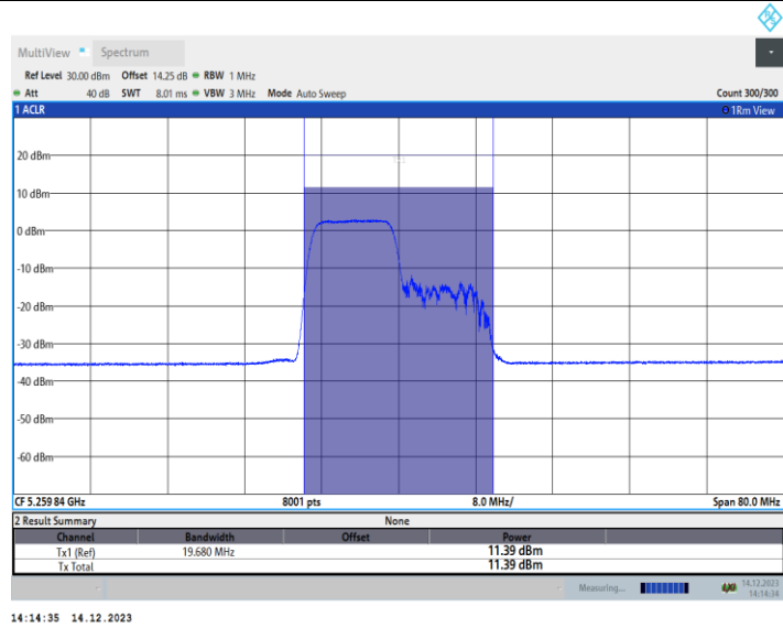
11AX40MIMO_Ant1_5270_242Tone_RU61
