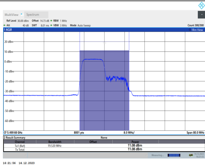
11AX40MIMO_Ant2_5510_242Tone_RU61
