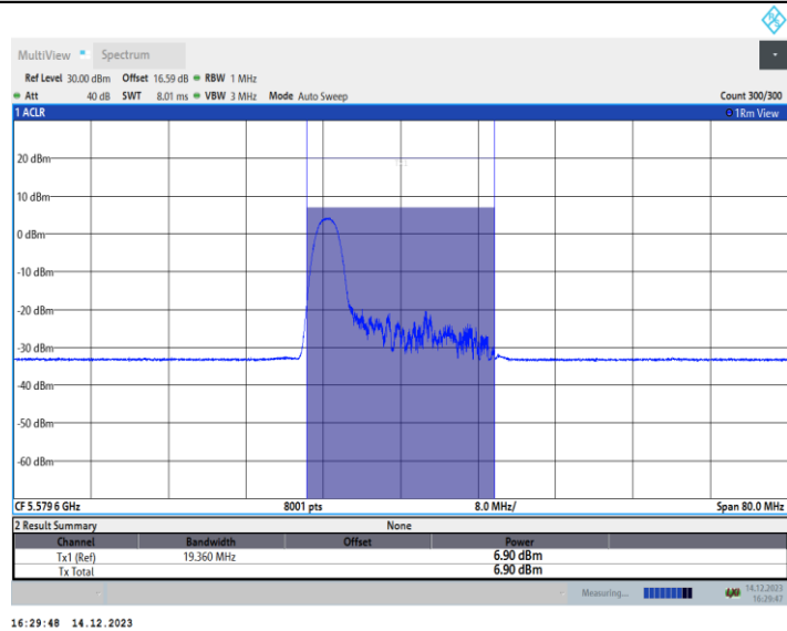
11AX40MIMO_Ant1_5590_52Tone_RU37
