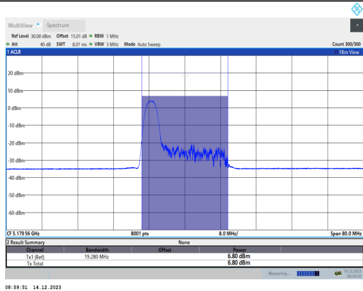
11AX40MIMO_Ant2_5190_52Tone_RU37
