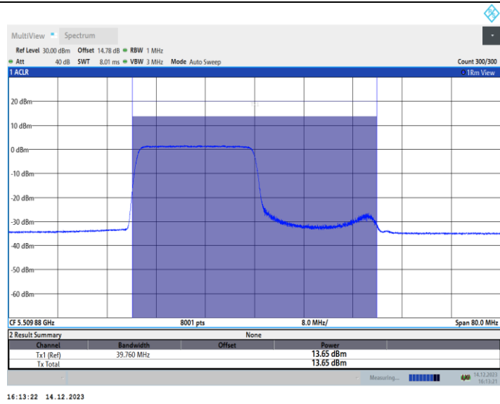
11AX40MIMO_Ant2_5510_26Tone_RU0
