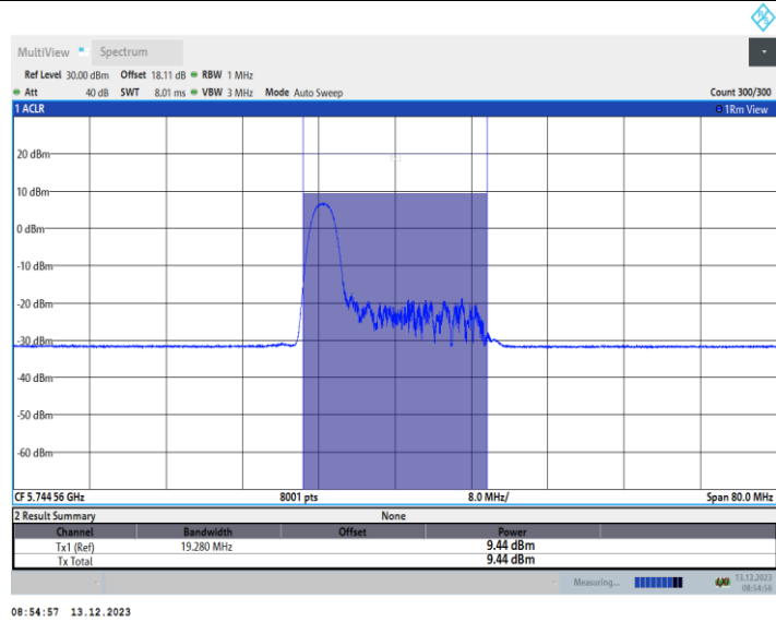
11AX40MIMO_Ant2_5755_52Tone_RU37
