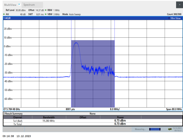
11AX40MIMO_Ant2_5795_52Tone_RU37
