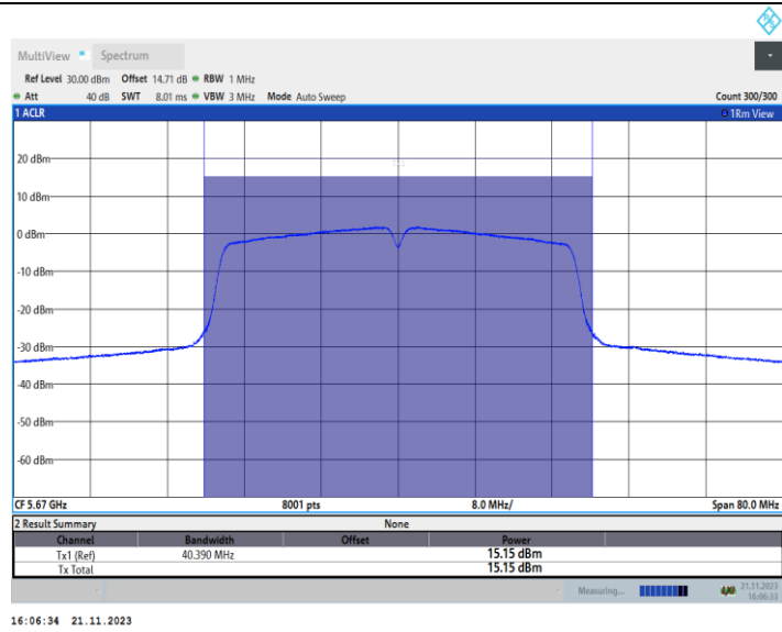
11AC40MIMO_Ant2_5670
