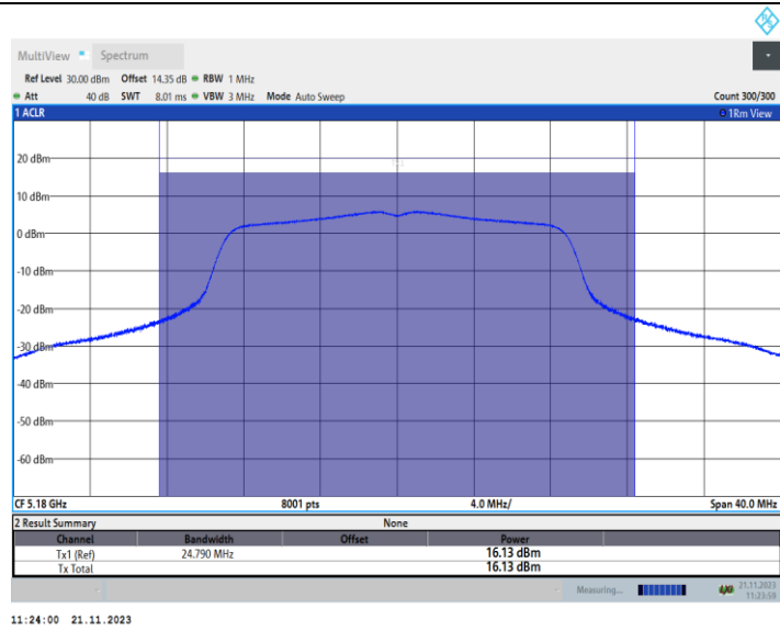
11AC20MIMO_Ant2_5180
