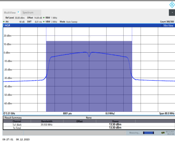
11AC40MIMO_Ant2_5310
