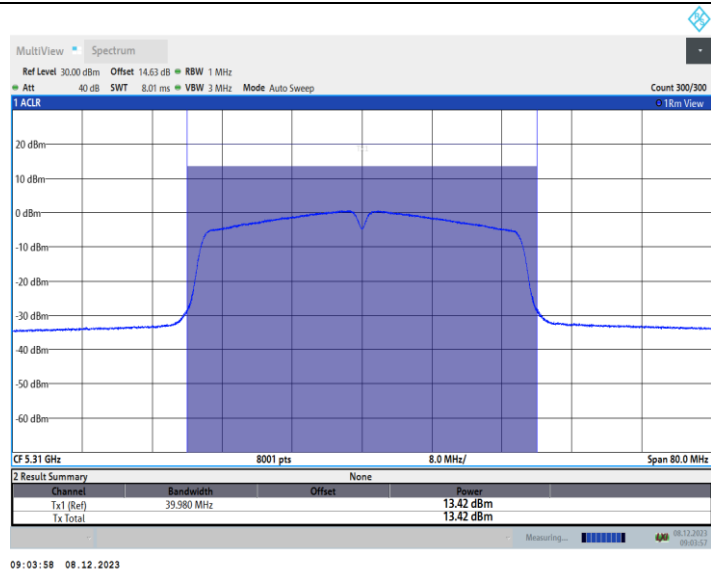
11N40MIMO_Ant2_5310
