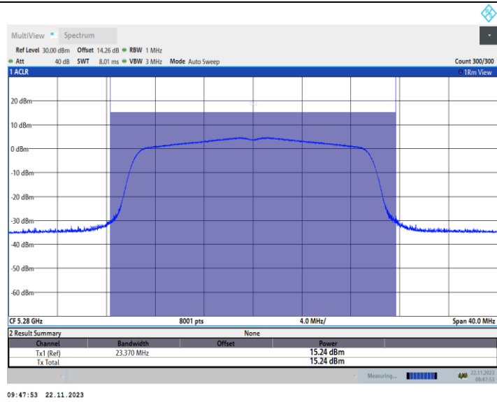
11AX20MIMO_Ant2_5280
