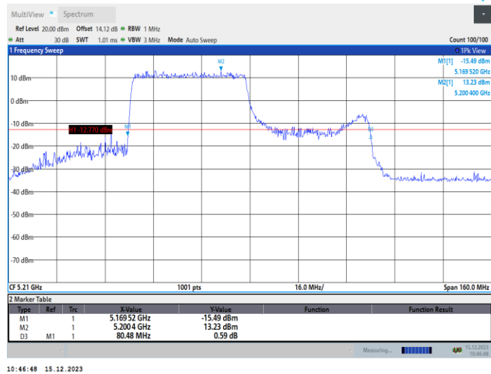
11AX80MIMO_Ant2_5210_26Tone_RU0
