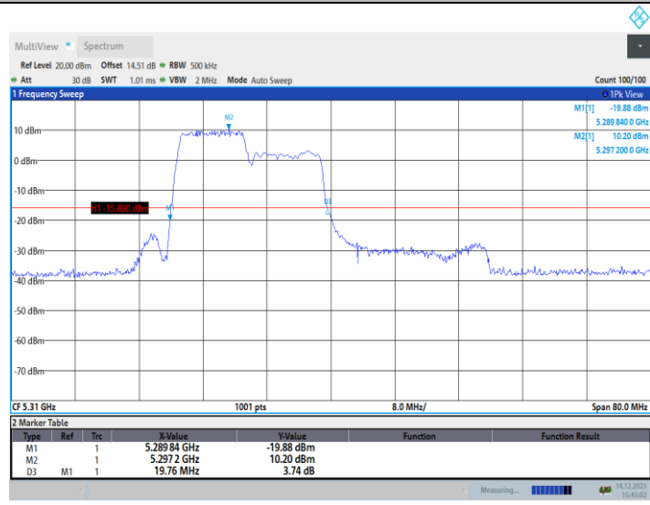
11AX40MIMO_Ant2_5310_242Tone_RU61
