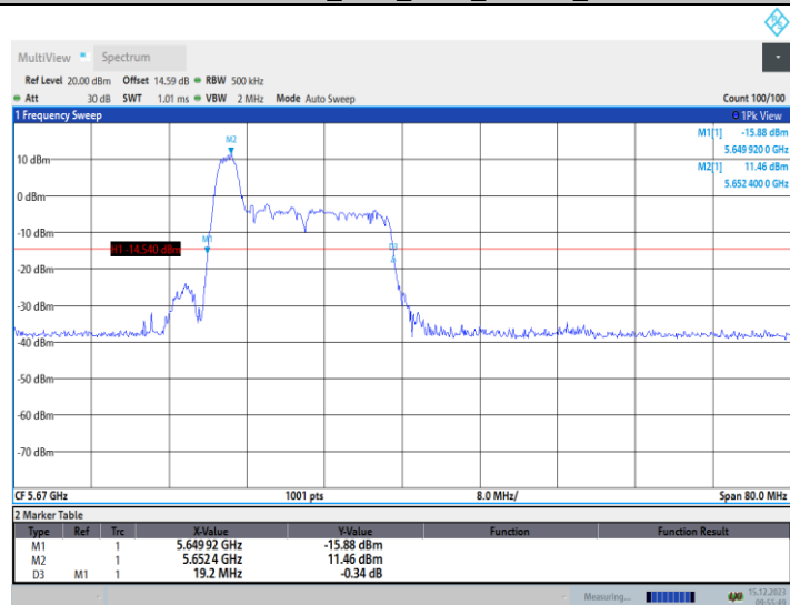
11AX40MIMO_Ant2_5670_26Tone_RU0
