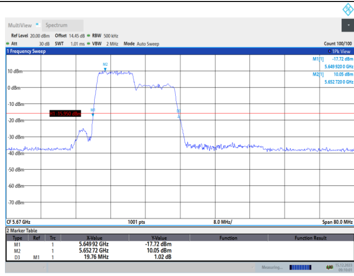
11AX40MIMO_Ant1_5670_242Tone_RU61
