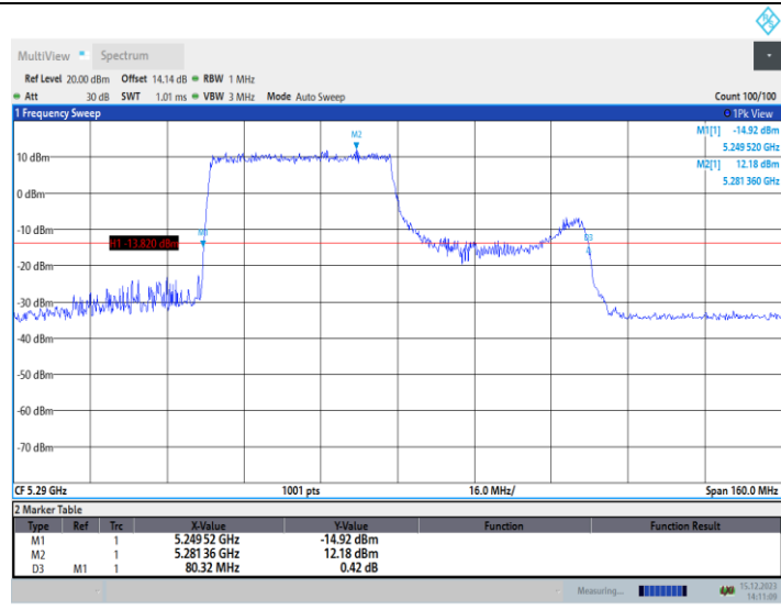
11AX80MIMO_Ant2_5290_26Tone_RU0
