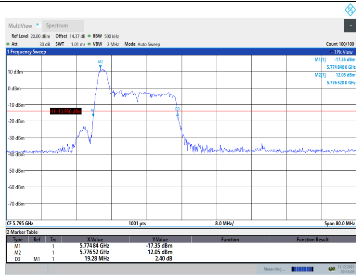
11AX40MIMO_Ant2_5795_52Tone_RU37
