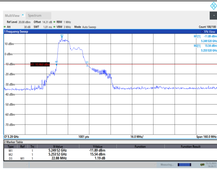
11AX80MIMO_Ant2_5290_242Tone_RU64
