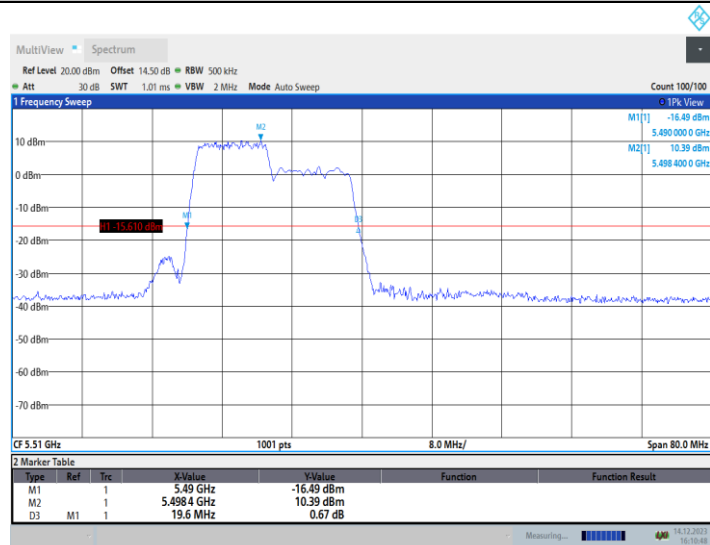
11AX40MIMO_Ant1_5510_106Tone_RU53
