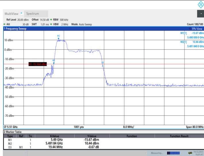
11AX40MIMO_Ant1_5510_52Tone_RU37
