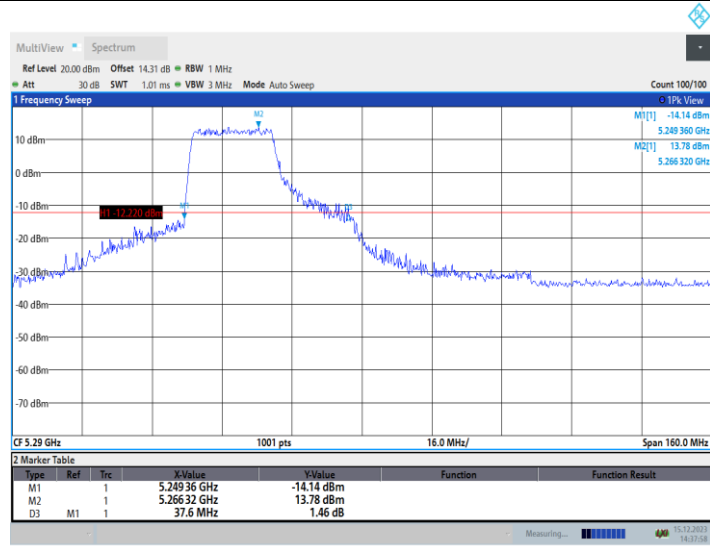
11AX80MIMO_Ant2_5290_484Tone_RU65
