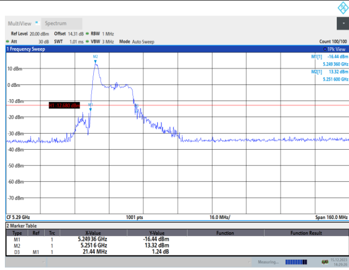
11AX80MIMO_Ant2_5290_52Tone_RU37
