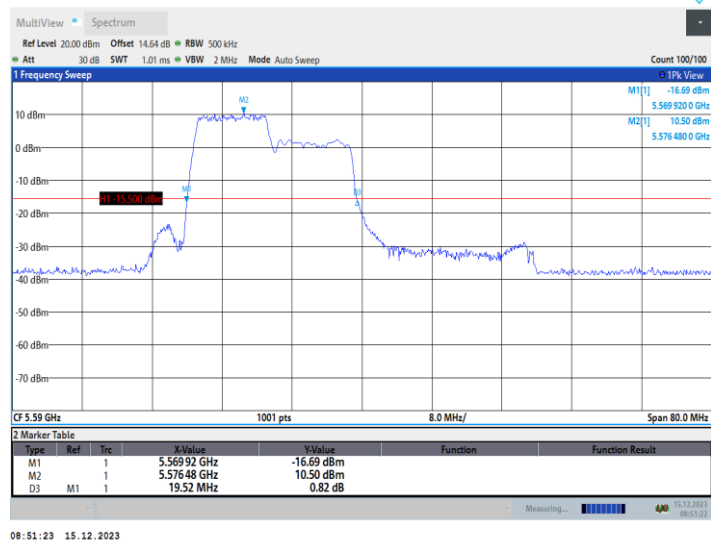
11AX40MIMO_Ant2_5590_242Tone_RU61
