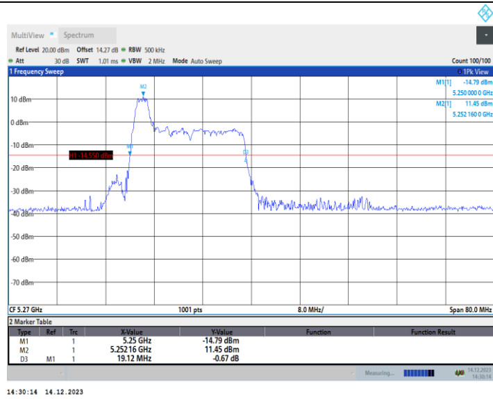
11AX40MIMO_Ant2_5270_52Tone_RU37
