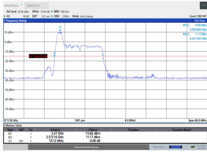
11AX40MIMO_Ant2_5590_52Tone_RU37
