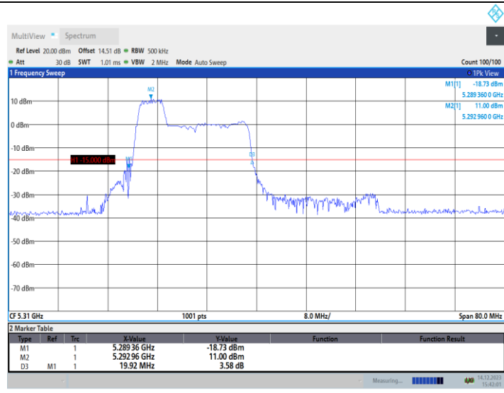
11AX40MIMO_Ant2_5310_106Tone_RU53
