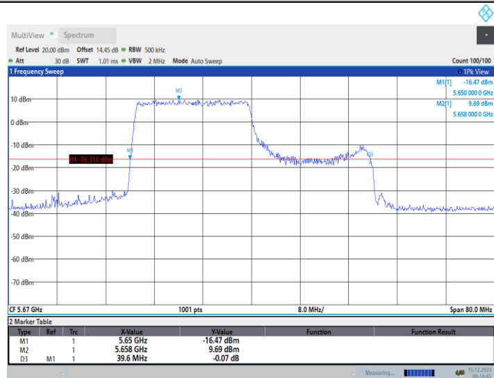
11AX40MIMO_Ant1_5670_242Tone_RU61
