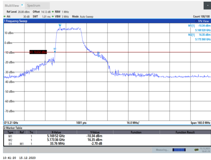
11AX80MIMO_Ant1_5210_484Tone_RU65
