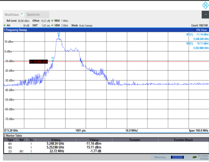
11AX80MIMO_Ant2_5290_106Tone_RU53
