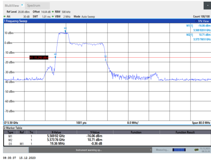
11AX40MIMO_Ant2_5590_106Tone_RU53
