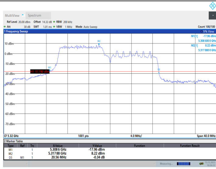
11AX20MIMO_Ant2_5320_26Tone_RU0
