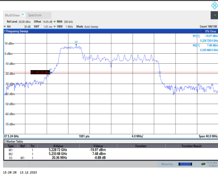
11AX20MIMO_Ant1_5240_106Tone_RU53
