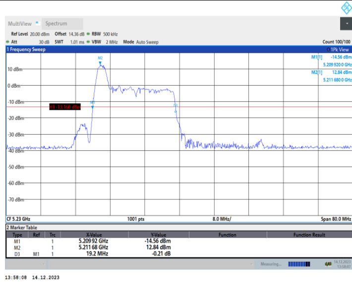
11AX40MIMO_Ant2_5230_52Tone_RU37
