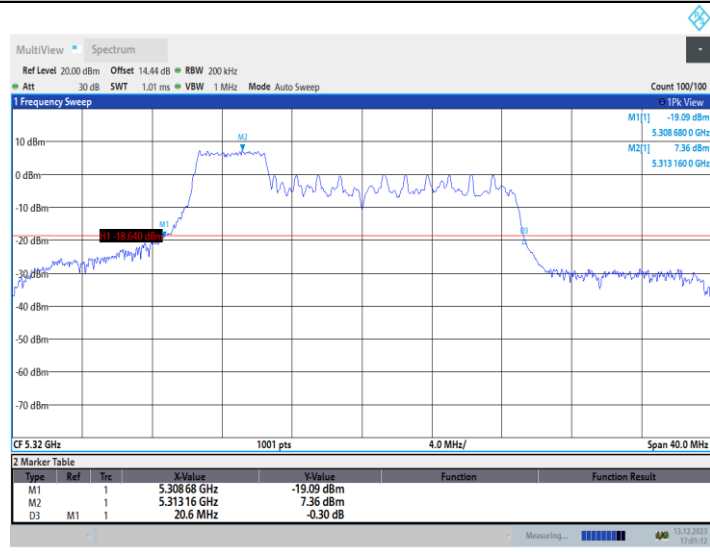
11AX20MIMO_Ant2_5320_106Tone_RU53
