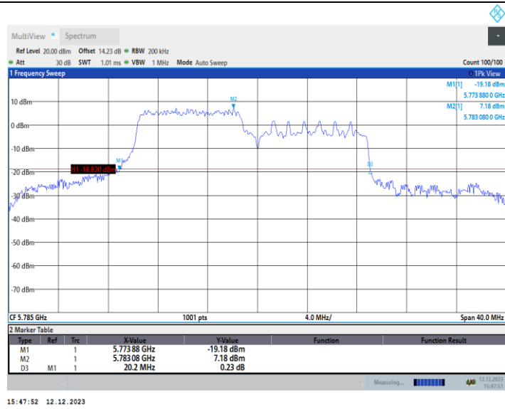
11AX20MIMO_Ant2_5785_26Tone_RU0
