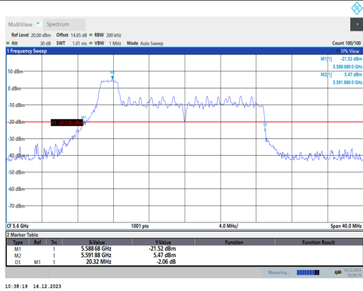
11AX20MIMO_Ant2_5600_52Tone_RU37
