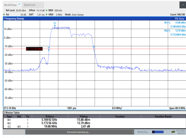
11AX40MIMO_Ant1_5190_242Tone_RU61
