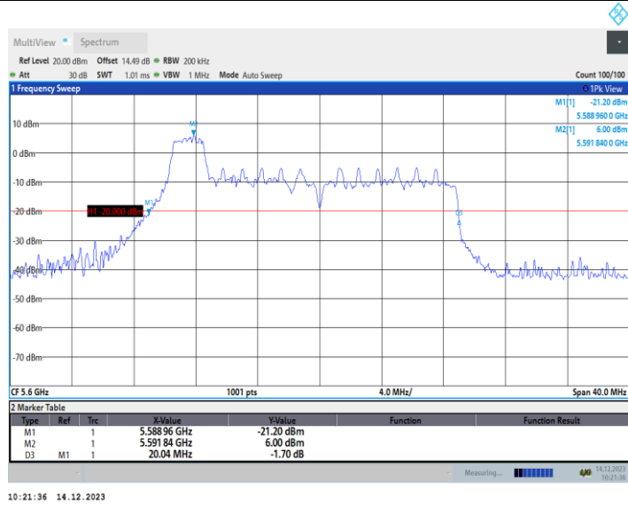
11AX20MIMO_Ant1_5600_52Tone_RU37
