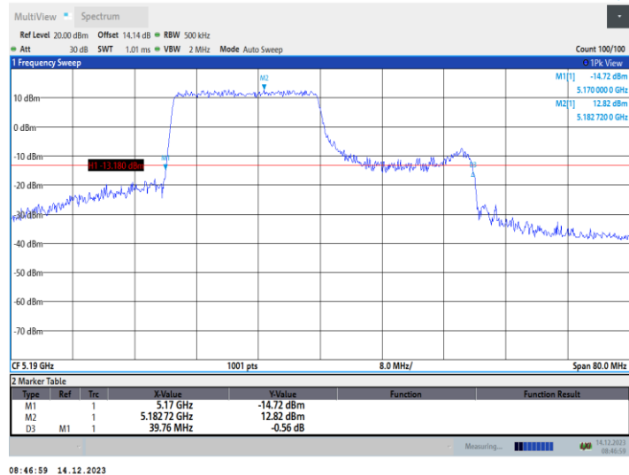
11AX40MIMO_Ant2_5190_26Tone_RU0
