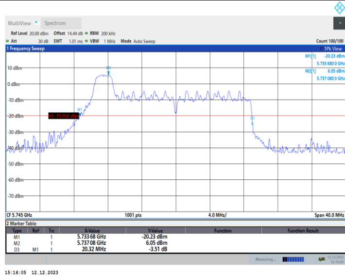
11AX20MIMO_Ant2_5745_52Tone_RU37
