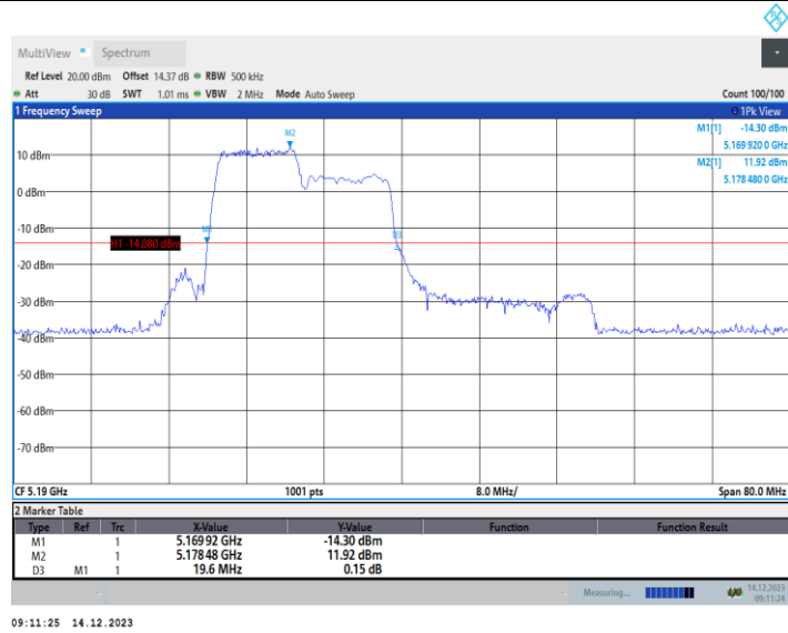
11AX40MIMO_Ant2_5190_242Tone_RU61
