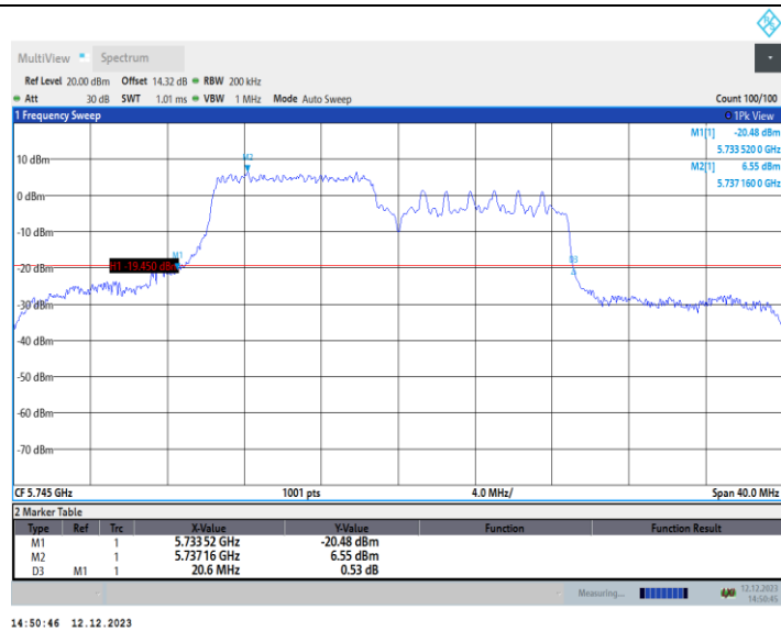
11AX20MIMO_Ant2_5745_26Tone_RU0
