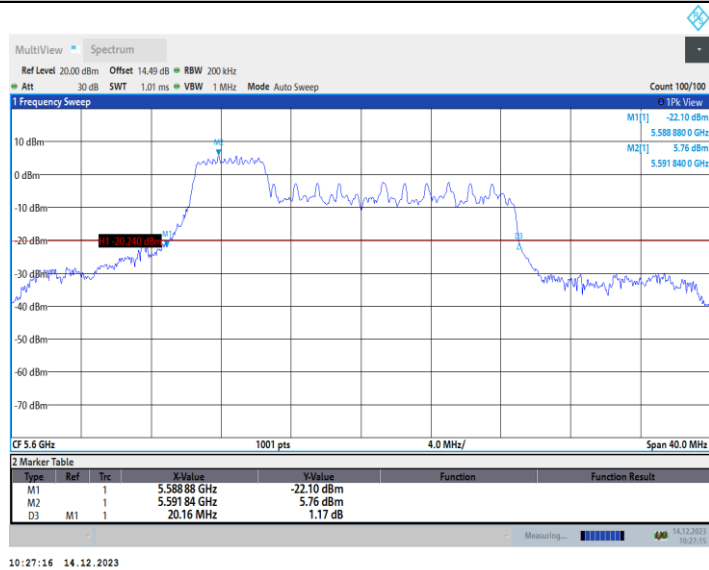
11AX20MIMO_Ant1_5600_106Tone_RU53
