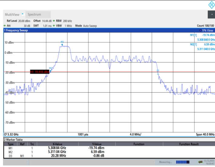
11AX20MIMO_Ant2_5320_52Tone_RU37
