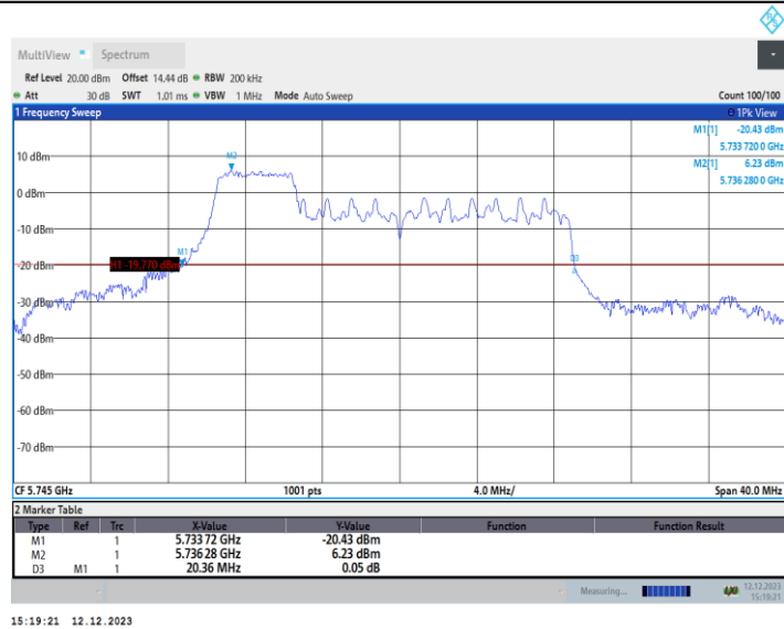
11AX20MIMO_Ant2_5745_106Tone_RU53
