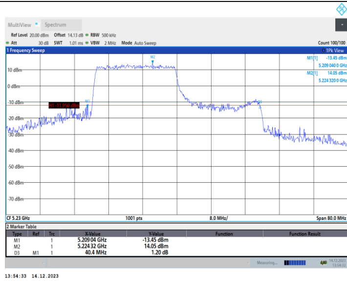
11AX40MIMO_Ant2_5230_26Tone_RU0
