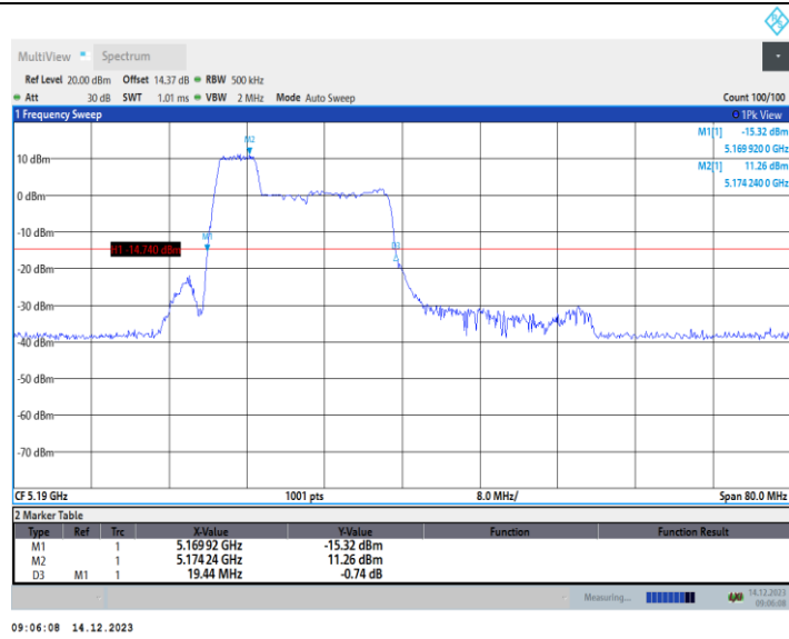
11AX40MIMO_Ant2_5190_106Tone_RU53
