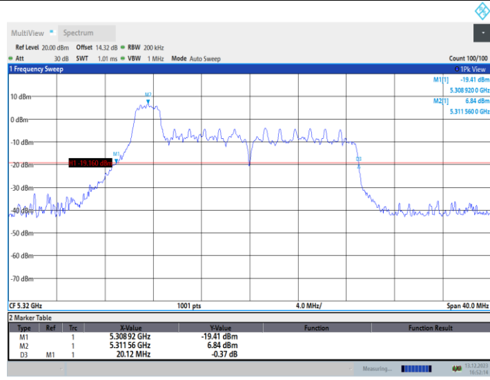
11AX20MIMO_Ant1_5320_52Tone_RU37
