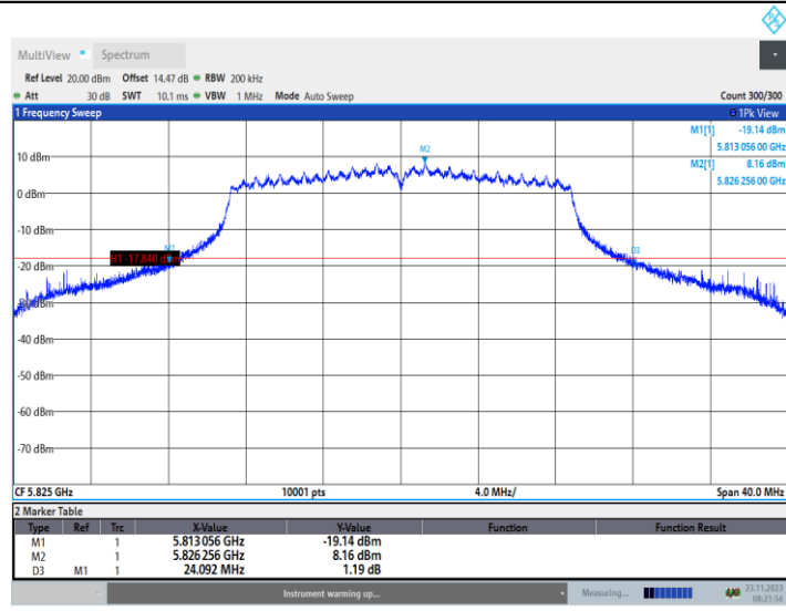
11N20MIMO_Ant2_5825
