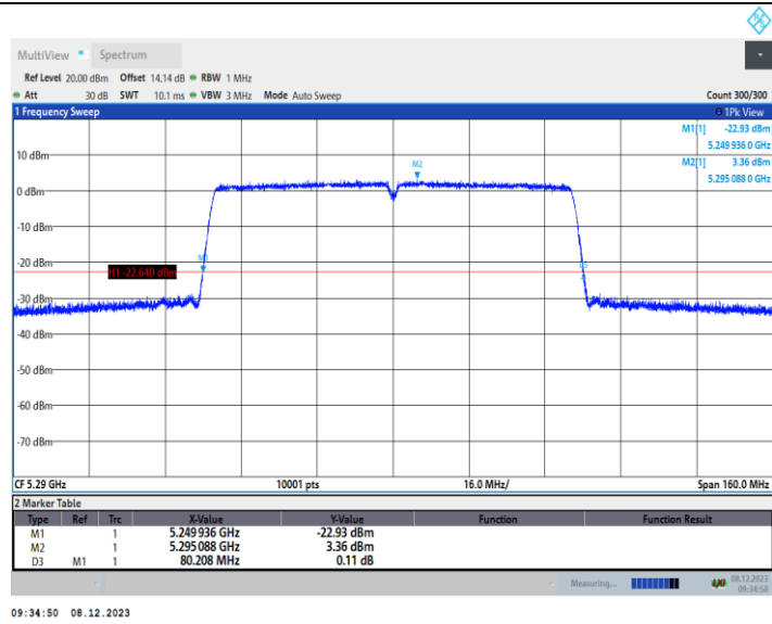
11AC80MIMO_Ant2_5290
