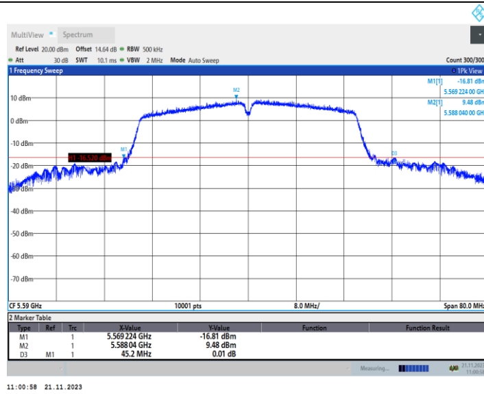
11N40MIMO_Ant1_5670
