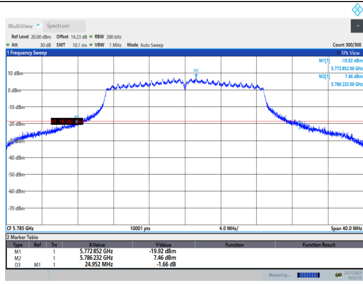
11N20MIMO_Ant2_5785
