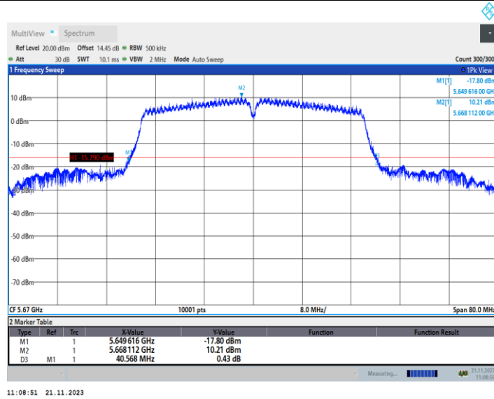
11N40MIMO_Ant2_5670
