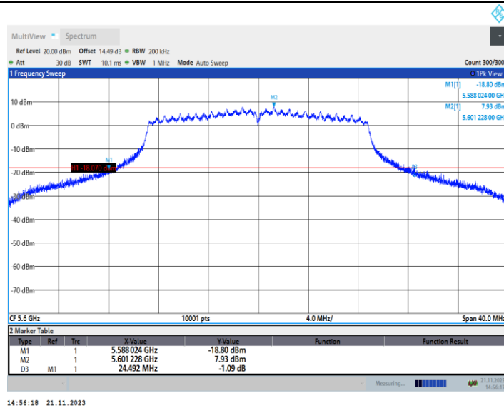
11AC20MIMO_Ant2_5600
