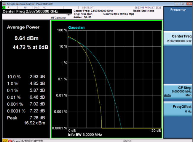
16QAM-21425
