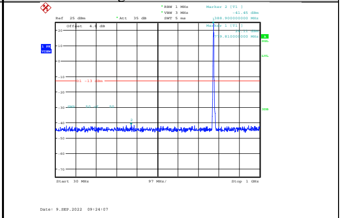
Band13-5MHz-QPSK-23230-1RB#0-Range1:30~1000MHz
