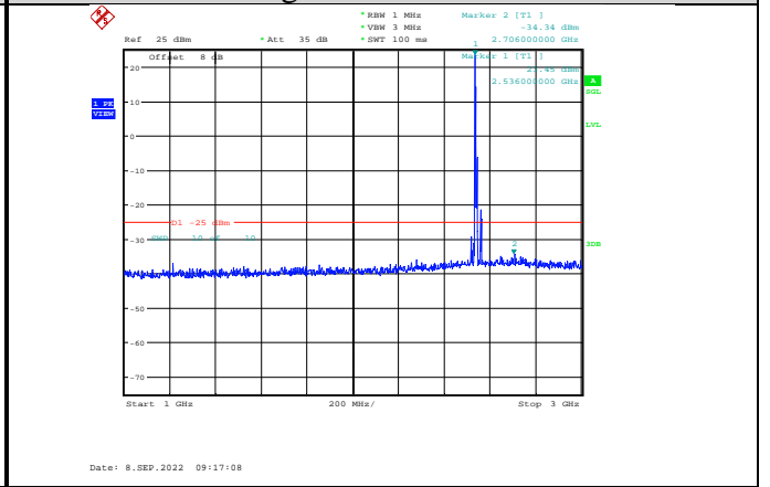
Band41-5MHz-16QAM-40065-1RB#0- Range2:1000~3000MHz
