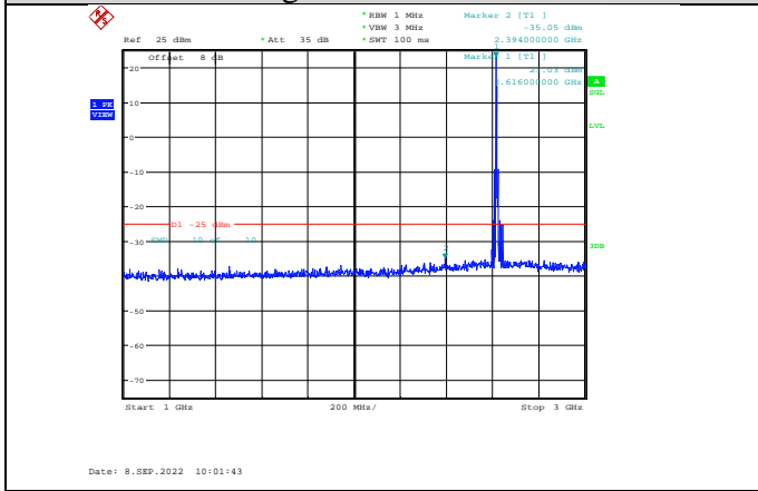
Band38-5MHz-QPSK-38225-1RB#0- Range2:1000~3000MHz
