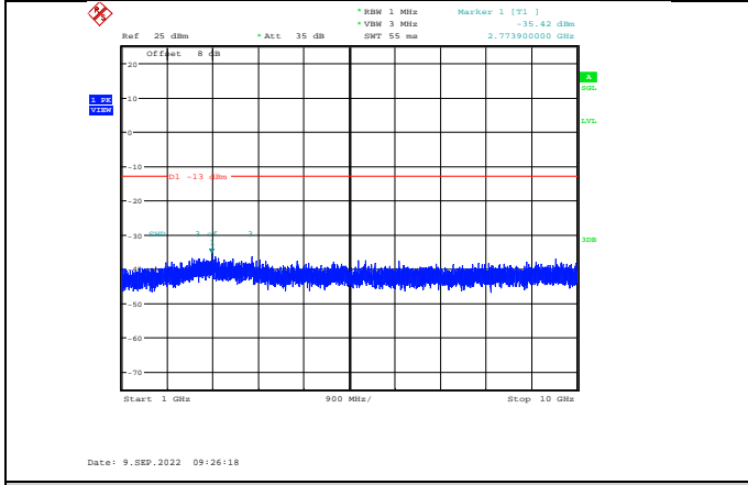
Band13-5MHz-QPSK-23255-1RB#0-Range2:1000~10000MHz
