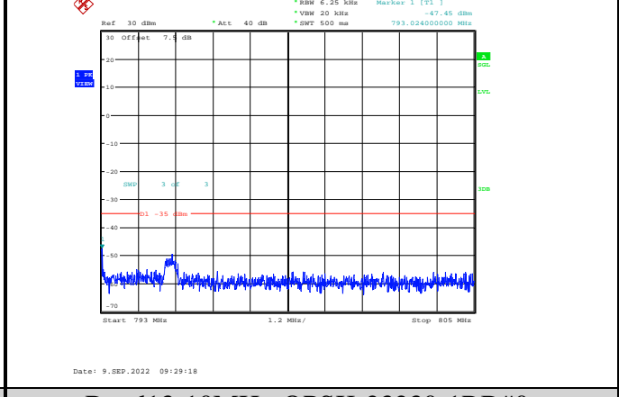
Band13-10MHz-QPSK-23230-1RB#0-Range4:793~805MHz
