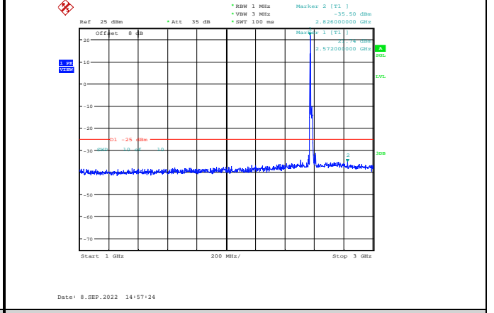
Band38-20MHz-64QAM-37850-1RB#0-Range2:1000~3000MHz
