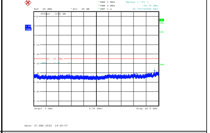
Band41-10MHz-QPSK-40090-1RB#0-Range3:3000~26500MHz
