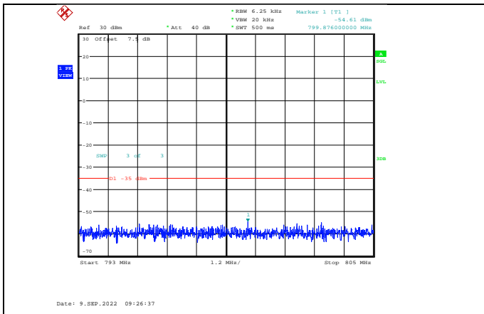
Band13-5MHz-QPSK-23255-1RB#0-Range4:793~805MHz
