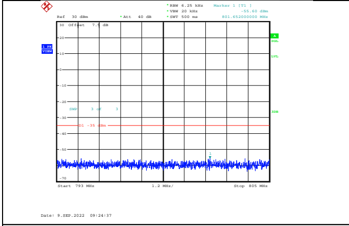
Band13-5MHz-QPSK-23230-1RB#0-Range4:793~805MHz
