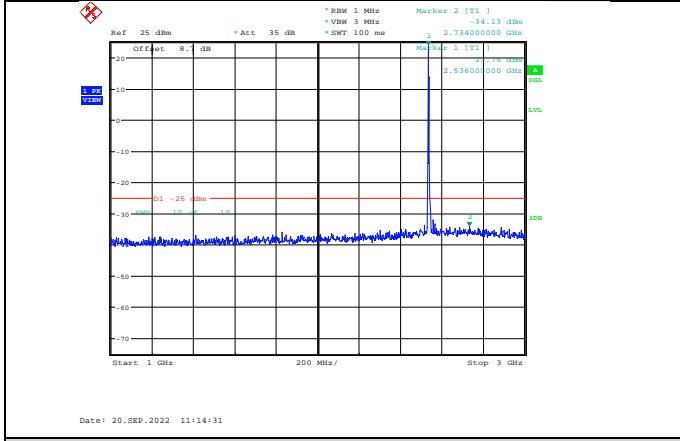
Band41-5MHz-64QAM-40065-1RB#0-Range2:1000~3000MHz
