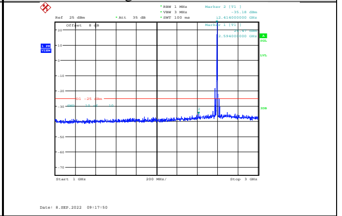
Band41-5MHz-QPSK-40640-1RB#0-Range2:1000~3000MHz
