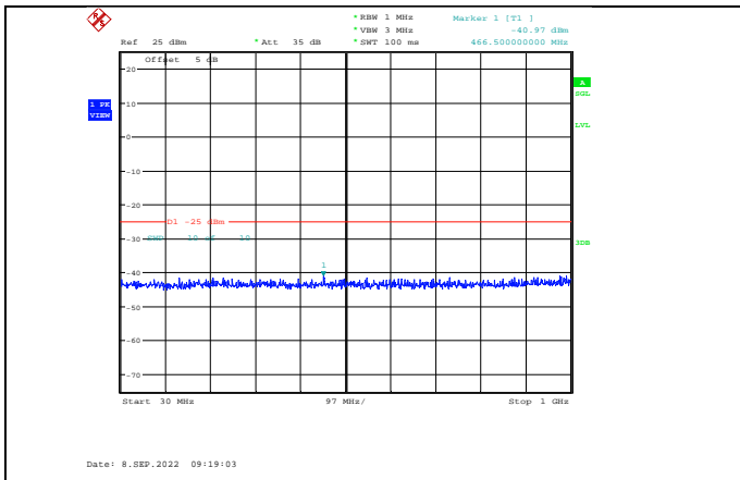
Band41-5MHz-QPSK-41215-1RB#0- Range1:30~1000MHz
