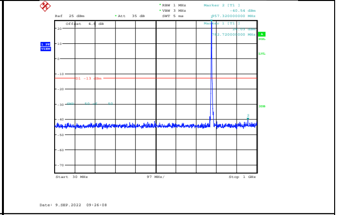
Band13-5MHz-QPSK-23255-1RB#0-Range1:30~1000MHz
