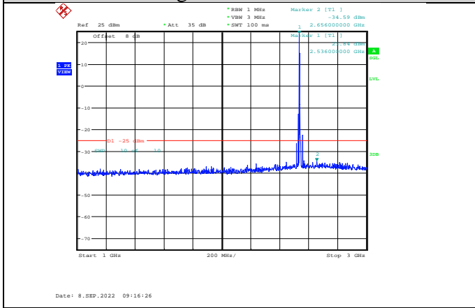
Band41-5MHz-QPSK-40065-1RB#0-Range2:1000~3000MHz
