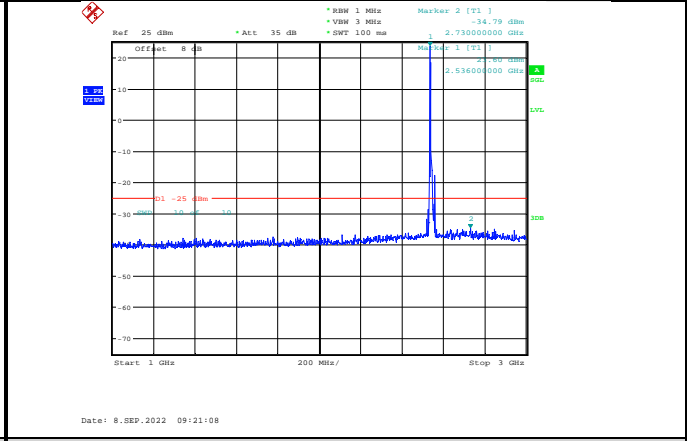
Band41-10MHz-QPSK-40090-1RB#0-Range2:1000~3000MHz
