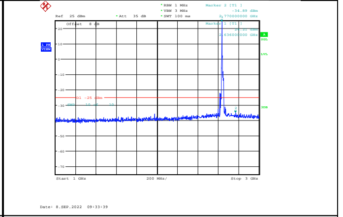
Band41-20MHz-QPSK-41140-1RB#0-Range2:1000~3000MHz
