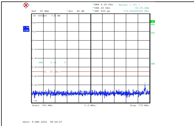
Band13-5MHz-QPSK-23230-1RB#0-Range3:763~775MHz
