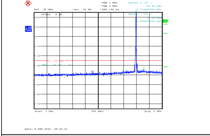
Band41-10MHz-QPSK-40640-1RB#0-Range2:1000~3000MHz
