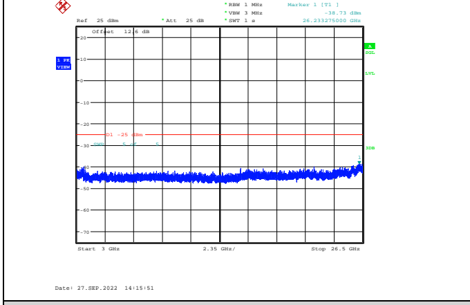
Band41-20MHz-QPSK-40640-1RB#0-Range3:3000~26500MHz
