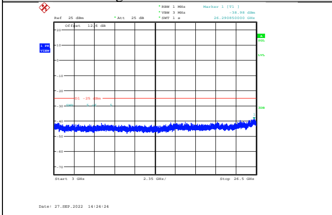
Band41-5MHz-QPSK-41215-1RB#0- Range3:3000~26500MHz
