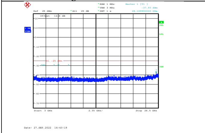
Band38-5MHz-QPSK-38225-1RB#0- Range3:3000~26500MHz
