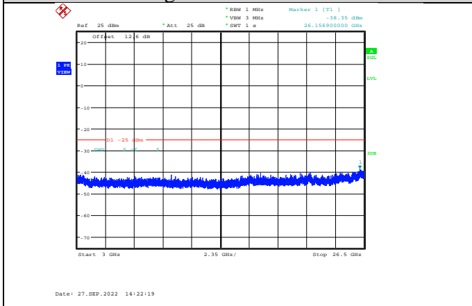
Band41-5MHz-QPSK-40065-1RB#0-Range3:3000~26500MHz
