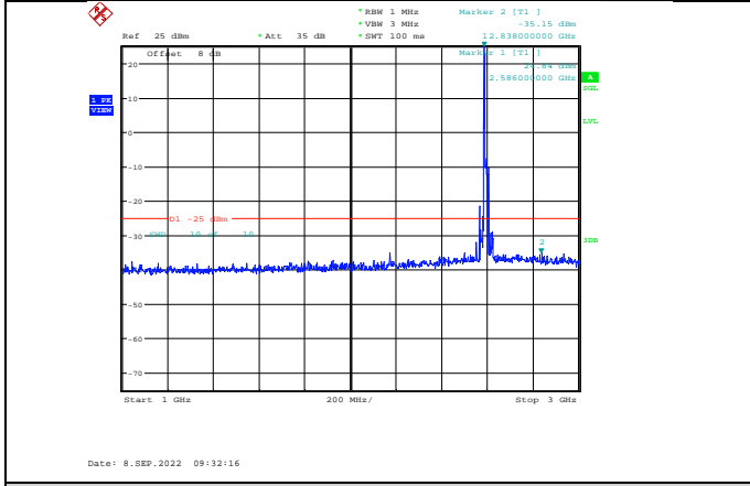
Band41-20MHz-QPSK-40640-1RB#0-Range2:1000~3000MHz
