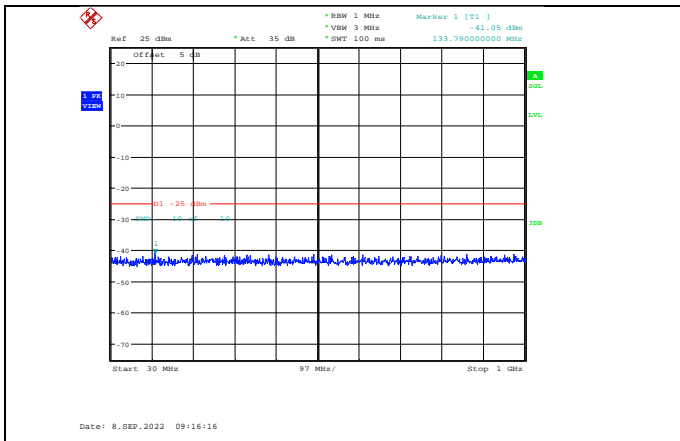
Band41-5MHz-QPSK-40065-1RB#0-Range1:30~1000MHz
