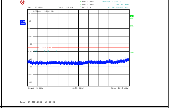
Band38-20MHz-QPSK-37850-1RB#0-Range3:3000~26500MHz
