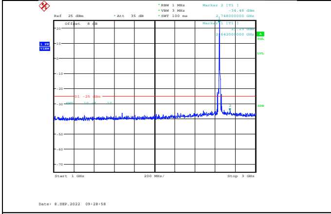
Band41-15MHz-QPSK-41165-1RB#0-Range2:1000~3000MHz
