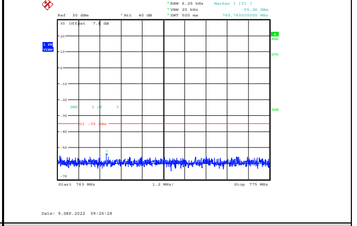
Band13-5MHz-QPSK-23255-1RB#0-Range3:763~775MHz
