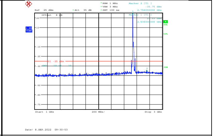
Band41-20MHz-QPSK-40140-1RB#0-Range2:1000~3000MHz
