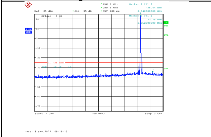
Band41-5MHz-QPSK-41215-1RB#0- Range2:1000~3000MHz
