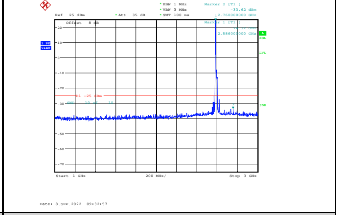
Band41-20MHz-16QAM-40640-1RB#0-Range2:1000~3000MHz
