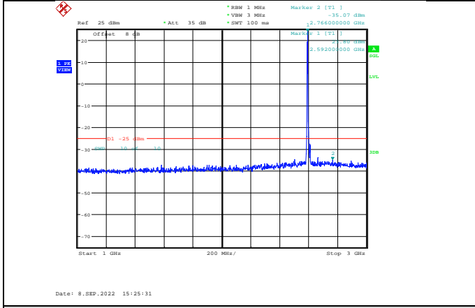
Band41-10MHz-64QAM-40640-1RB#0- Range2:1000~3000MHz
