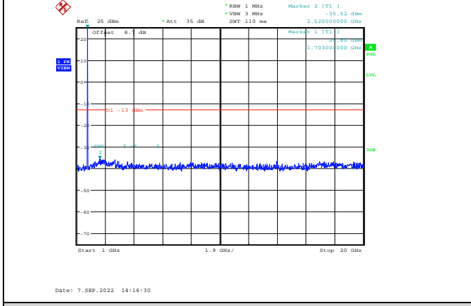
Band4-1.4MHz-QPSK-19957-1RB#0-Range2:1000~20000MHz
