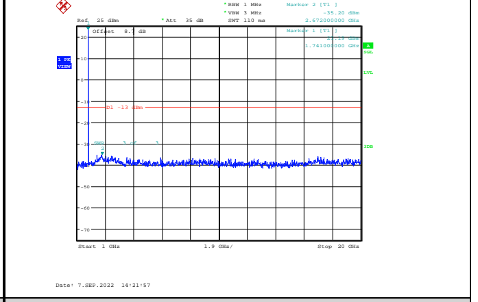
Band4-3MHz-QPSK-20385-1RB#0-Range2:1000~20000MHz
