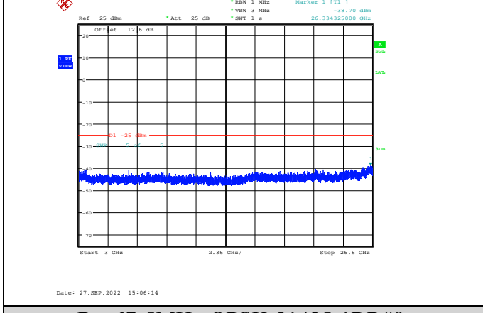
Band7-5MHz-QPSK-21425-1RB#0-Range3:3000~26500MHz
