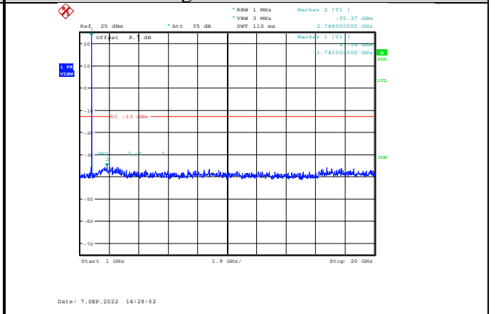
Band4-10MHz-QPSK-20350-1RB#0-Range2:1000~20000MHz
