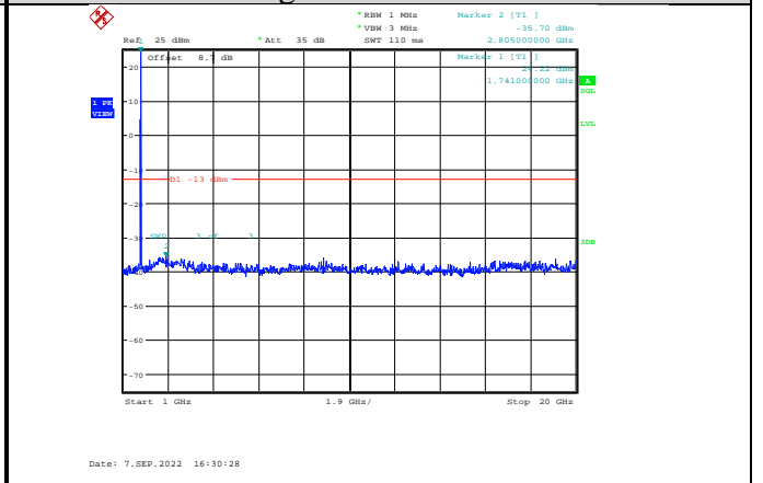
Band4-15MHz-QPSK-20325-1RB#0- Range2:1000~20000MHz
