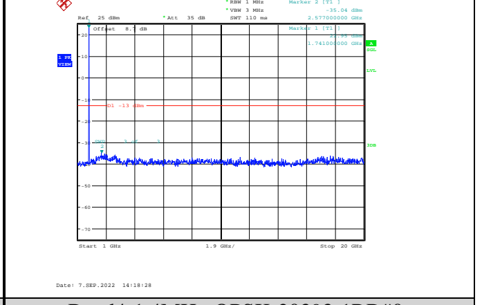
Band4-1.4MHz-QPSK-20393-1RB#0-Range2:1000~20000MHz
