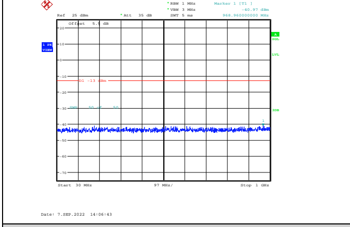
Band2-20MHz-QPSK-18900-1RB#0-Range1:30~1000MHz
