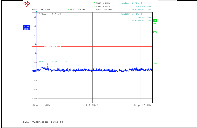
Band4-3MHz-QPSK-19965-1RB#0-Range2:1000~20000MHz
