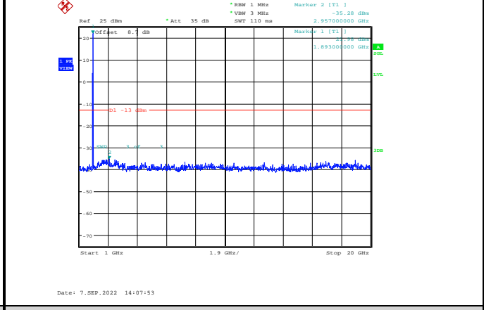
Band2-20MHz-QPSK-19100-1RB#0-Range2:1000~20000MHz
