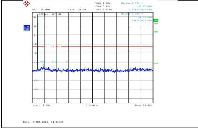
Band2-20MHz-16QAM-18700-1RB#0-Range2:1000~20000MHz
