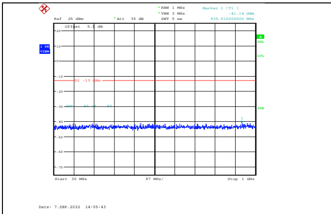
Band2-20MHz-QPSK-18700-1RB#0-Range1:30~1000MHz
