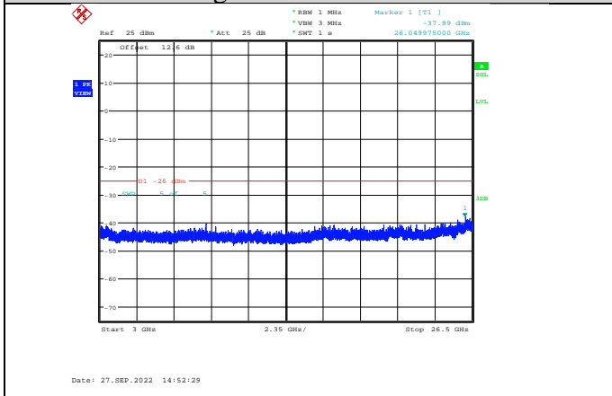
Band7-20MHz-QPSK-21100-1RB#0-Range3:3000~26500MHz
