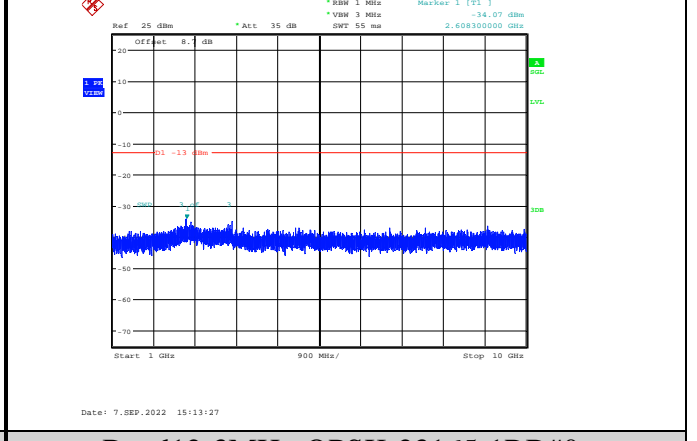
Band12-3MHz-QPSK-23165-1RB#0-Range2:1000~10000MHz
