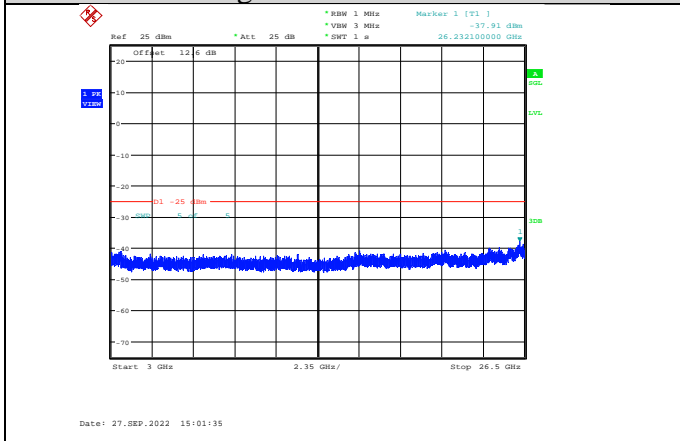
Band7-10MHz-QPSK-21100-1RB#0-Range3:3000~26500MHz
