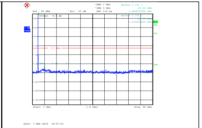
Band2-20MHz-16QAM-18900-1RB#0-Range2:1000~20000MHz
