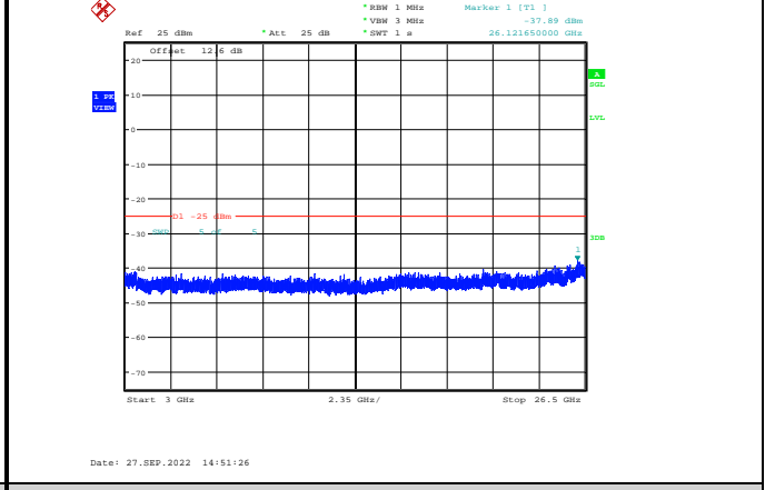
Band7-20MHz-QPSK-20850-1RB#0-Range3:3000~26500MHz
