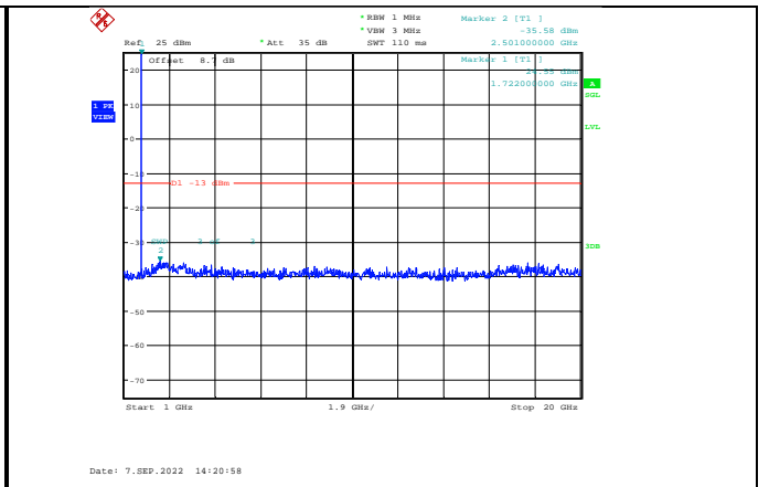
Band4-3MHz-QPSK-20175-1RB#0-Range2:1000~20000MHz
