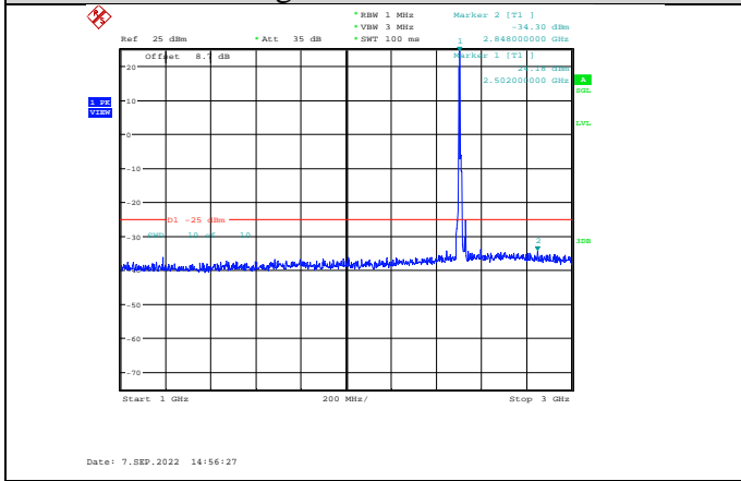
Band7-15MHz-QPSK-20825-1RB#0-Range2:1000~3000MHz
