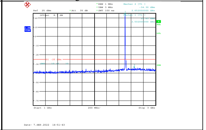
Band7-10MHz-QPSK-20800-1RB#0-Range2:1000~3000MHz
