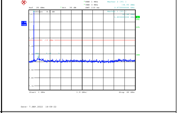
Band2-20MHz-16QAM-19100-1RB#0-Range2:1000~20000MHz
