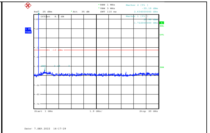
Band4-1.4MHz-QPSK-20175-1RB#0-Range2:1000~20000MHz
