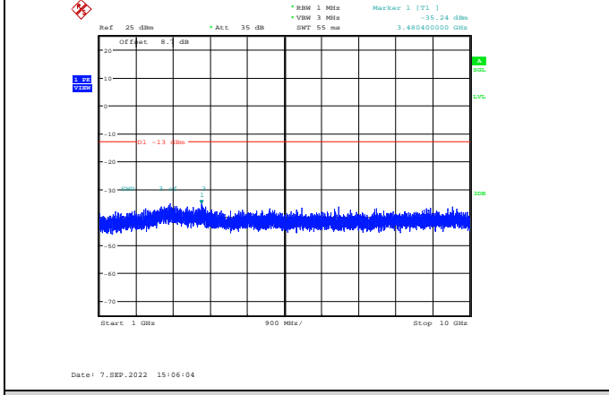
Band12-1.4MHz-QPSK-23017-1RB#0-Range2:1000~10000MHz
