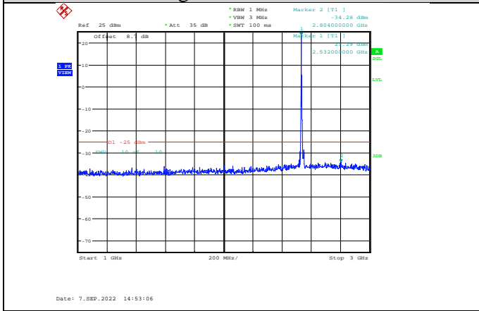
Band7-10MHz-QPSK-21100-1RB#0-Range2:1000~3000MHz
