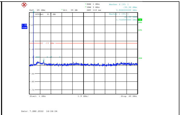
Band4-5MHz-QPSK-20175-1RB#0-Range2:1000~20000MHz
