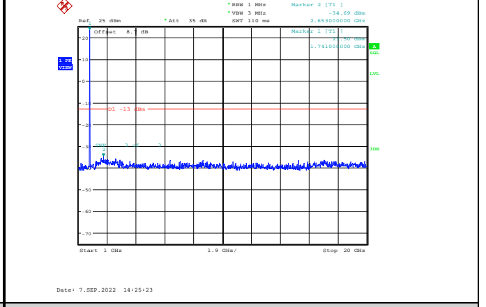
Band4-5MHz-QPSK-20375-1RB#0-Range2:1000~20000MHz
