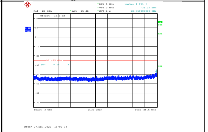
Band7-10MHz-QPSK-20800-1RB#0-Range3:3000~26500MHz
