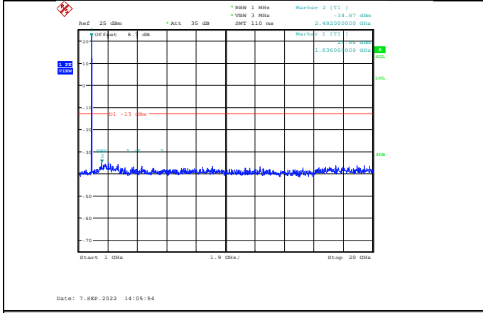
Band2-20MHz-QPSK-18700-1RB#0-Range2:1000~20000MHz
