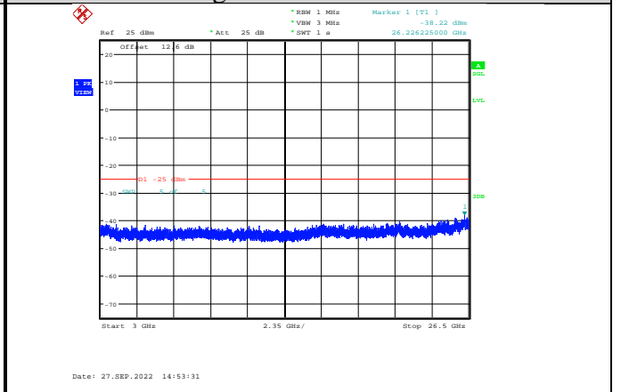
Band7-20MHz-QPSK-21350-1RB#0-Range3:3000~26500MHz
