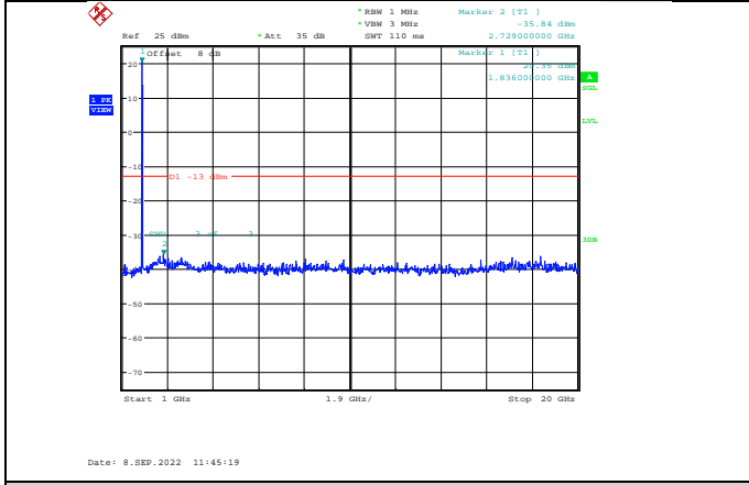
Band2-20MHz-64QAM-18700-1RB#0-Range2:1000~20000MHz
