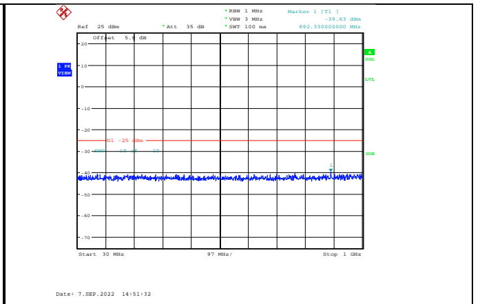
Band7-10MHz-QPSK-20800-1RB#0-Range1:30~1000MHz
