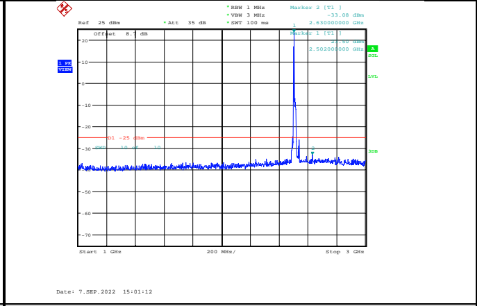
Band7-20MHz-QPSK-20850-1RB#0-Range2:1000~3000MHz
