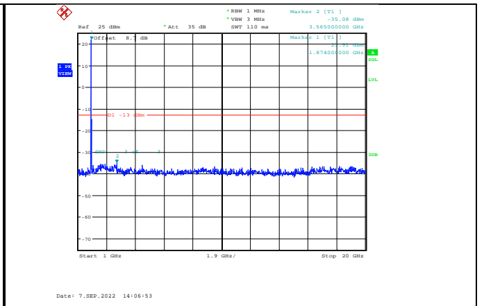
Band2-20MHz-QPSK-18900-1RB#0-Range2:1000~20000MHz
