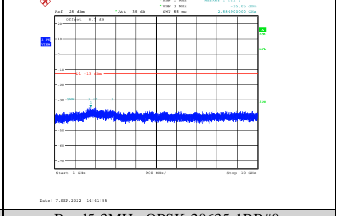
Band5-3MHz-QPSK-20635-1RB#0-Range2:1000~10000MHz
