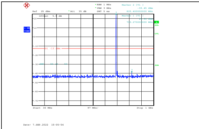
Band12-1.4MHz-QPSK-23017-1RB#0-Range1:30~1000MHz
