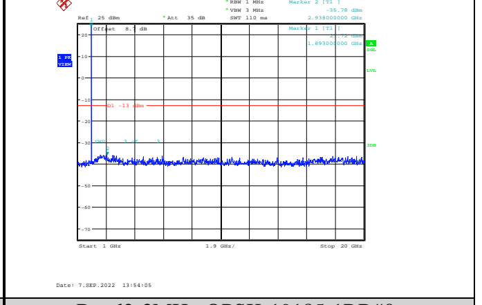
Band2-3MHz-QPSK-19185-1RB#0-Range2:1000~20000MHz
