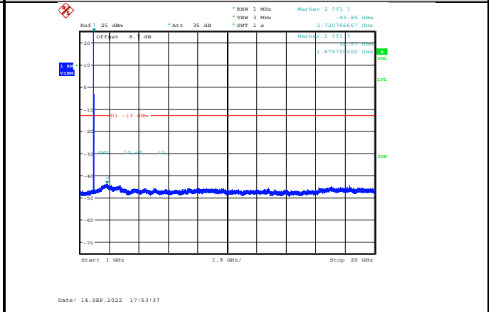
GSM1900-810-0-1000~20000MHz
