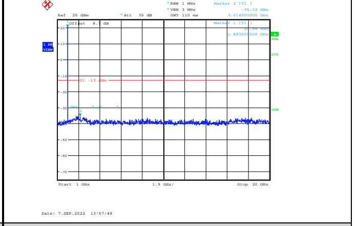
Band2-5MHz-16QAM-19175-1RB#0-Range2:1000~20000MHz
