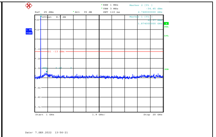
Band2-5MHz-QPSK-18900-1RB#0-Range2:1000~20000MHz
