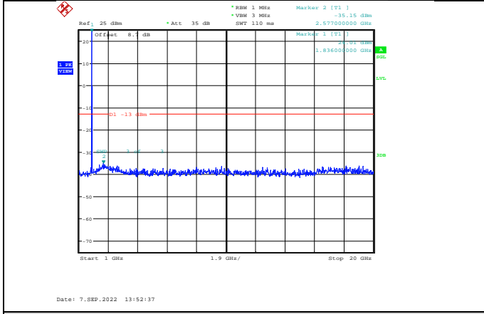
Band2-3MHz-16QAM-18615-1RB#0-Range2:1000~20000MHz
