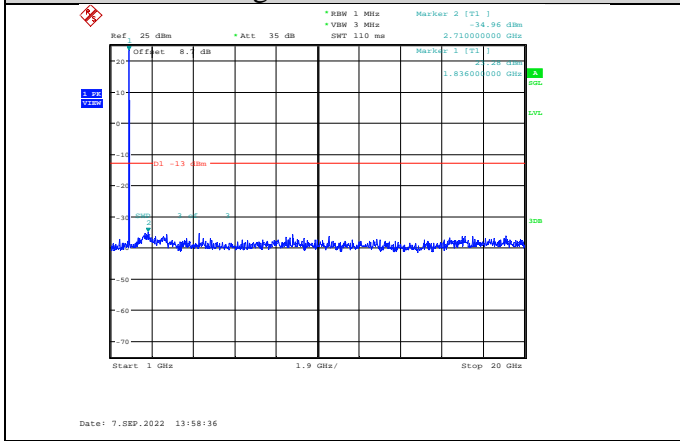
Band2-10MHz-QPSK-18650-1RB#0-Range2:1000~20000MHz
