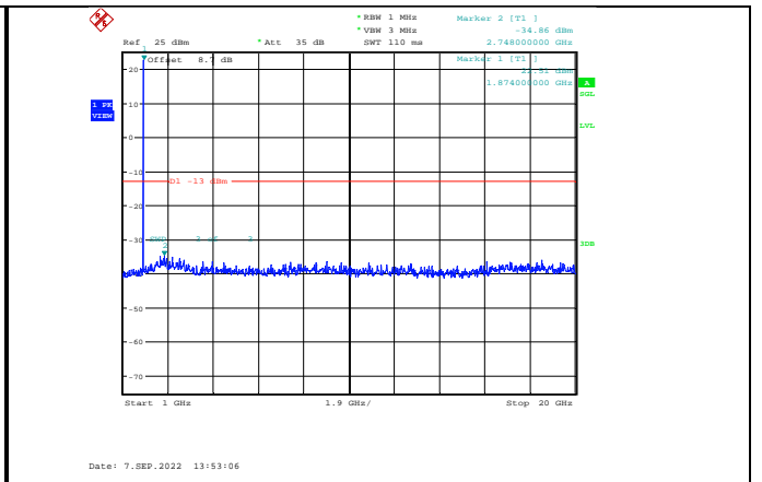
Band2-3MHz-QPSK-18900-1RB#0-Range2:1000~20000MHz
