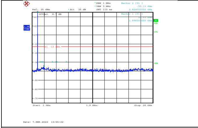
Band2-5MHz-QPSK-18625-1RB#0-Range2:1000~20000MHz
