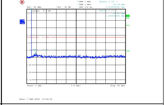
Band2-3MHz-16QAM-19185-1RB#0-Range2:1000~20000MHz
