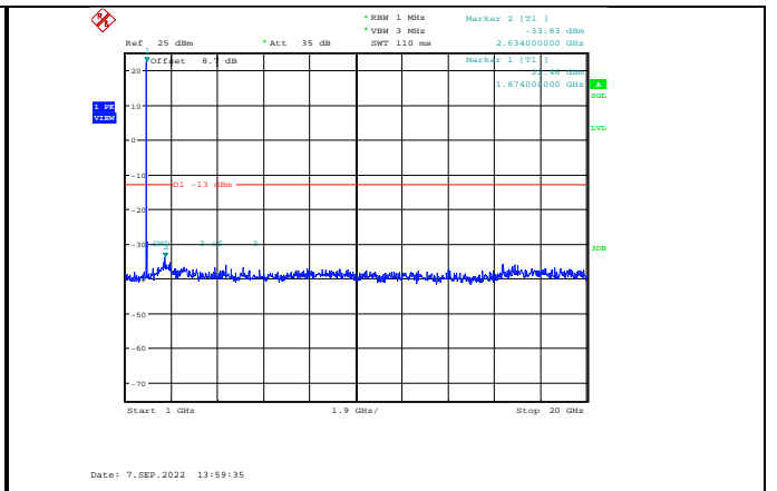
Band2-10MHz-QPSK-18900-1RB#0-Range2:1000~20000MHz
