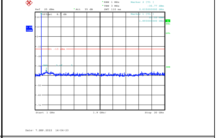
Band2-15MHz-QPSK-19125-1RB#0-Range2:1000~20000MHz
