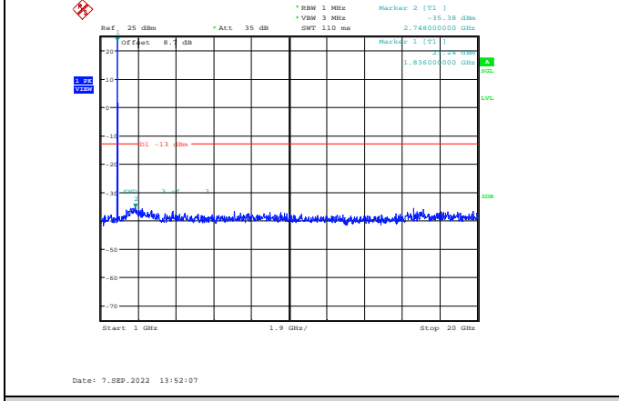
Band2-3MHz-QPSK-18615-1RB#0-Range2:1000~20000MHz
