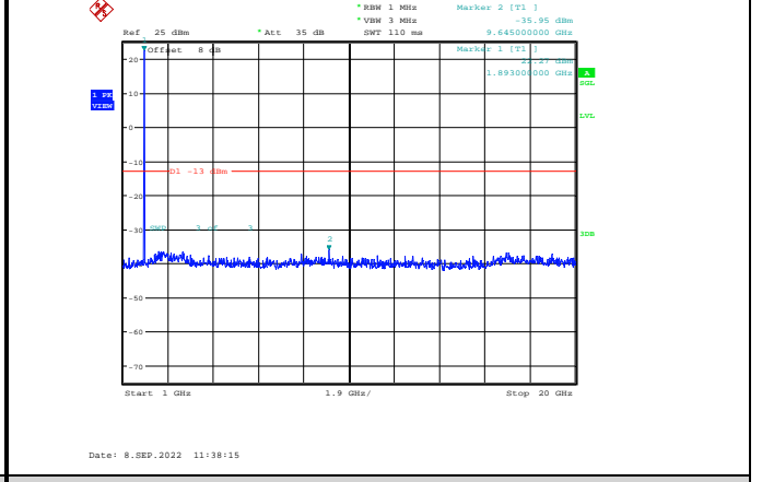
Band2-3MHz-64QAM-19185-1RB#0-Range2:1000~20000MHz
