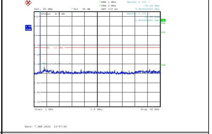
Band2-5MHz-QPSK-19175-1RB#0-Range2:1000~20000MHz
