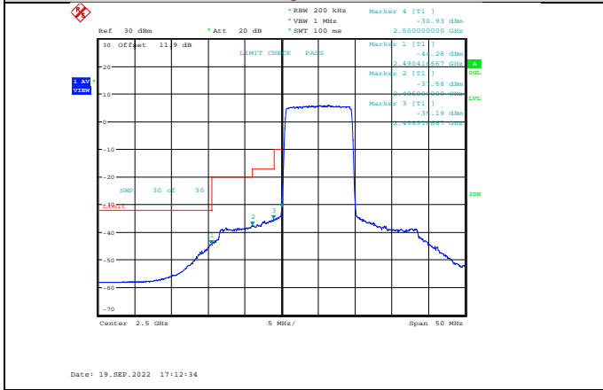
Band7-10MHz-QPSK-20800-50RB#0
