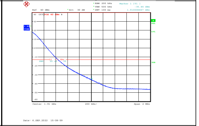
Band2-20MHz-64QAM-19100-1RB#99
