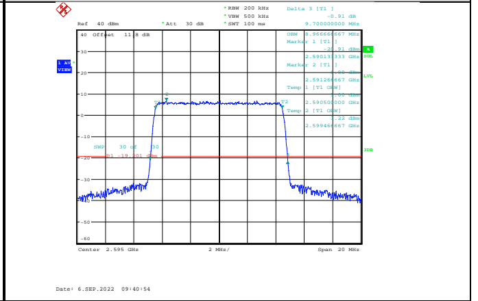
Band41-10MHz-QPSK-40640-50RB#0
