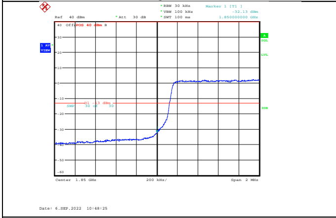
Band2-3MHz-QPSK-18615-15RB#0
