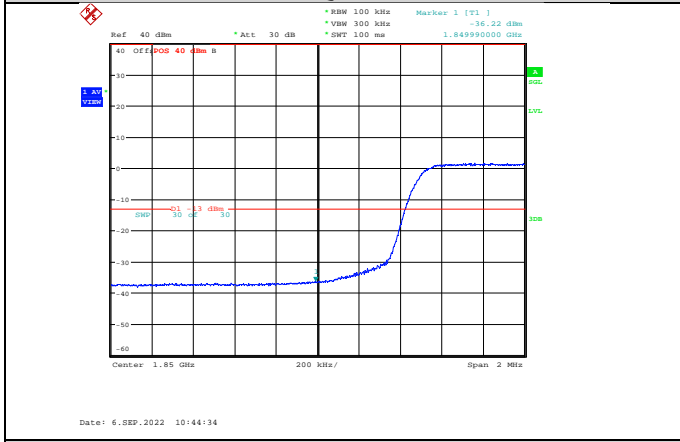
Band2-10MHz-QPSK-18650-50RB#0
