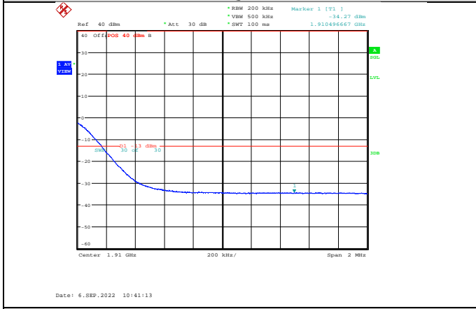
Band2-20MHz-16QAM-19100-100RB#0
