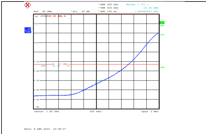
Band2-20MHz-QPSK-18700-1RB#0
