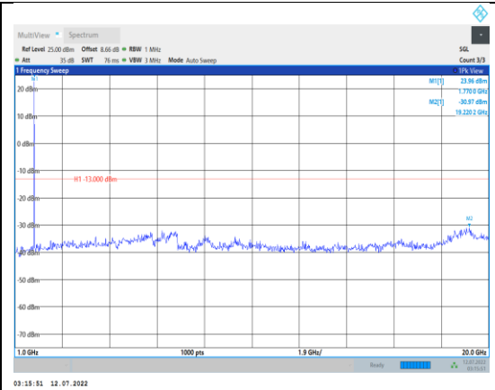
Band66-5MHz-QPSK-132647-1RB#0- Range2:1000~20000MHz
