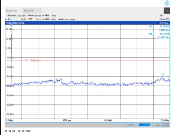
Band66-20MHz-QPSK-132072-1RB#0- Range2:1000~20000MHz
