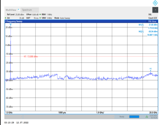
Band66-3MHz-QPSK-131987-1RB#0- Range2:1000~20000MHz
