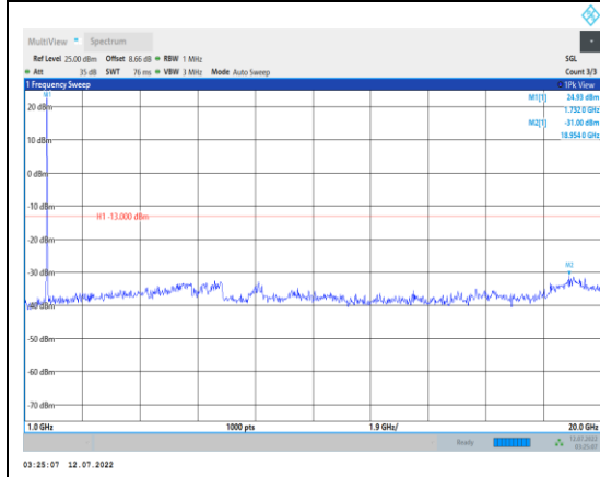
Band66-20MHz-QPSK-132322-1RB#0- Range2:1000~20000MHz
