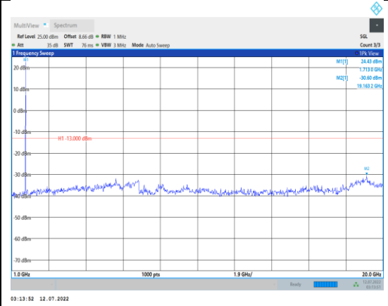
Band66-5MHz-QPSK-131997-1RB#0- Range2:1000~20000MHz
