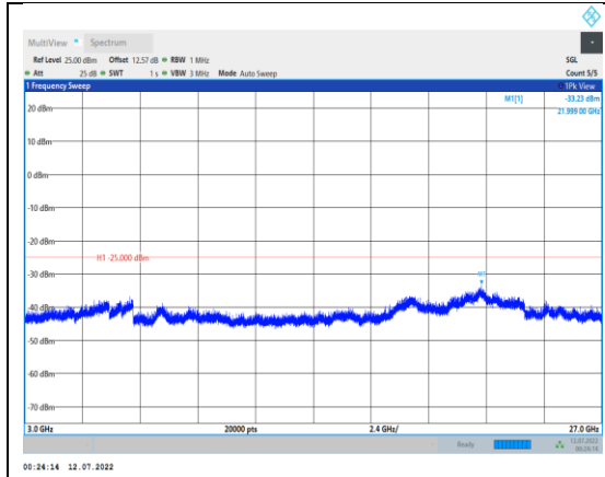
Band41-20MHz-QPSK-41490-1RB#0-Range3:3000~27000MHz
