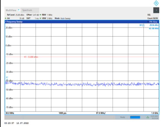
Band66-20MHz-QPSK-132072-1RB#0- Range1:30~1000MHz
