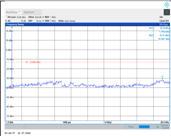
Band66-20MHz-QPSK-132572-1RB#0- Range2:1000~20000MHz
