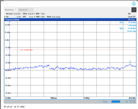
Band66-10MHz-QPSK-132622-1RB#0- Range2:1000~20000MHz
