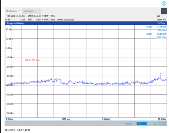
Band66-10MHz-QPSK-132022-1RB#0- Range2:1000~20000MHz
