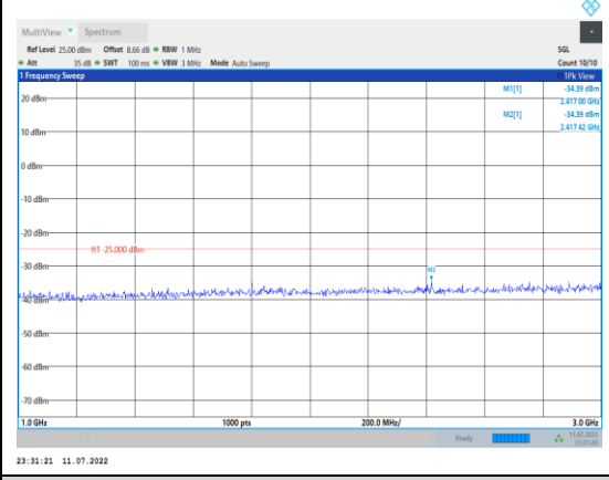
Band41-15MHz-QPSK-41515-1RB#0- Range2:1000~3000MHz
