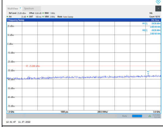
Band38-20MHz-16QAM-37850-1RB#0- Range2:1000~3000MHz
