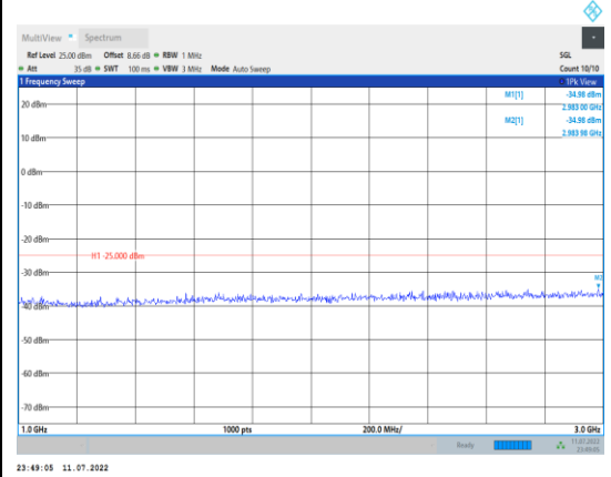
Band41-20MHz-QPSK-39750-1RB#0- Range2:1000~3000MHz
