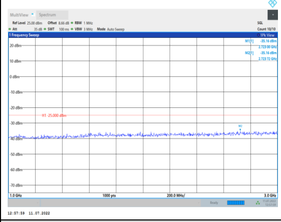
Band38-20MHz-QPSK-38150-1RB#0- Range2:1000~3000MHz
