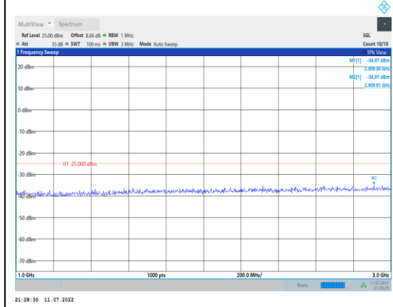
Band41-5MHz-QPSK-40620-1RB#0- Range2:1000~3000MHz
