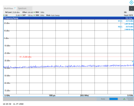
Band38-20MHz-QPSK-37850-1RB#0- Range2:1000~3000MHz
