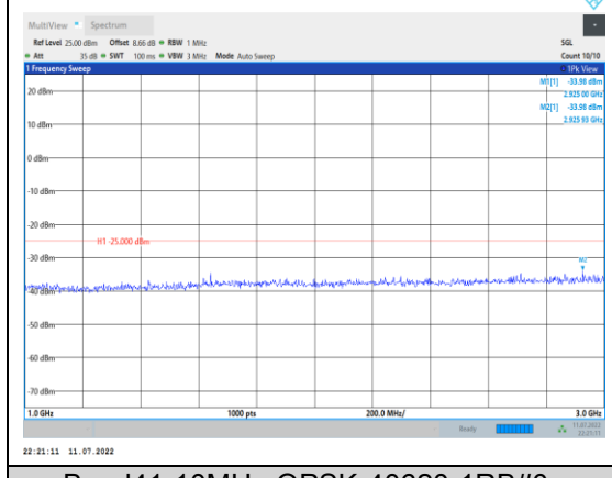
Band41-10MHz-QPSK-40620-1RB#0- Range2:1000~3000MHz
