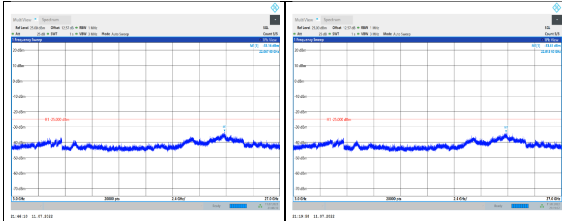
Band41-5MHz-QPSK-41565-1RB#0- Range3:3000~27000MHz
