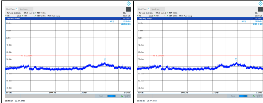
Band41-20MHz-QPSK-39750-1RB#0- Range3:3000~27000MHz
