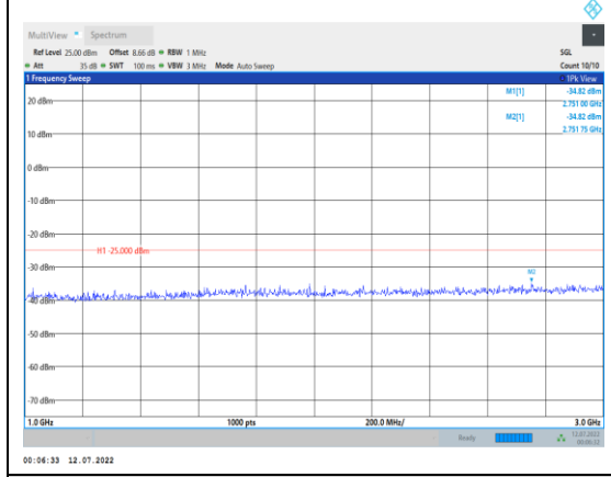
Band41-20MHz-QPSK-40620-1RB#0- Range2:1000~3000MHz
