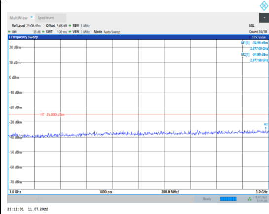
Band41-5MHz-QPSK-39675-1RB#0- Range2:1000~3000MHz
