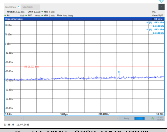
Band41-10MHz-QPSK-41540-1RB#0- Range2:1000~3000MHz
