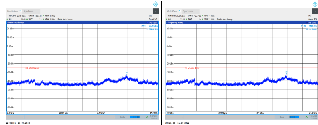
Band41-10MHz-QPSK-39700-1RB#0- Range3:3000~27000MHz
