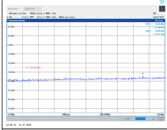
Band38-20MHz-QPSK-38000-1RB#0- Range2:1000~3000MHz
