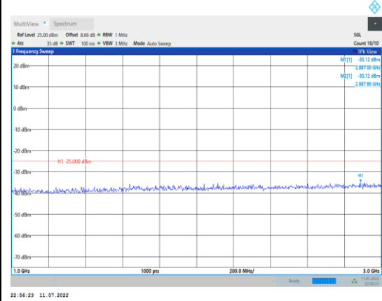
Band41-15MHz-QPSK-39725-1RB#0- Range2:1000~3000MHz
