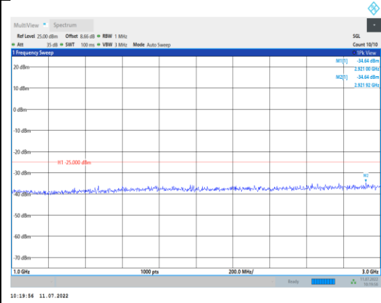
Band38-5MHz-QPSK-38225-1RB#0- Range2:1000~3000MHz
