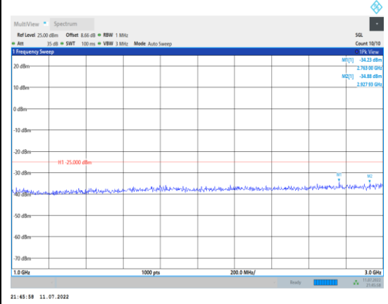
Band41-5MHz-QPSK-41565-1RB#0- Range2:1000~3000MHz
