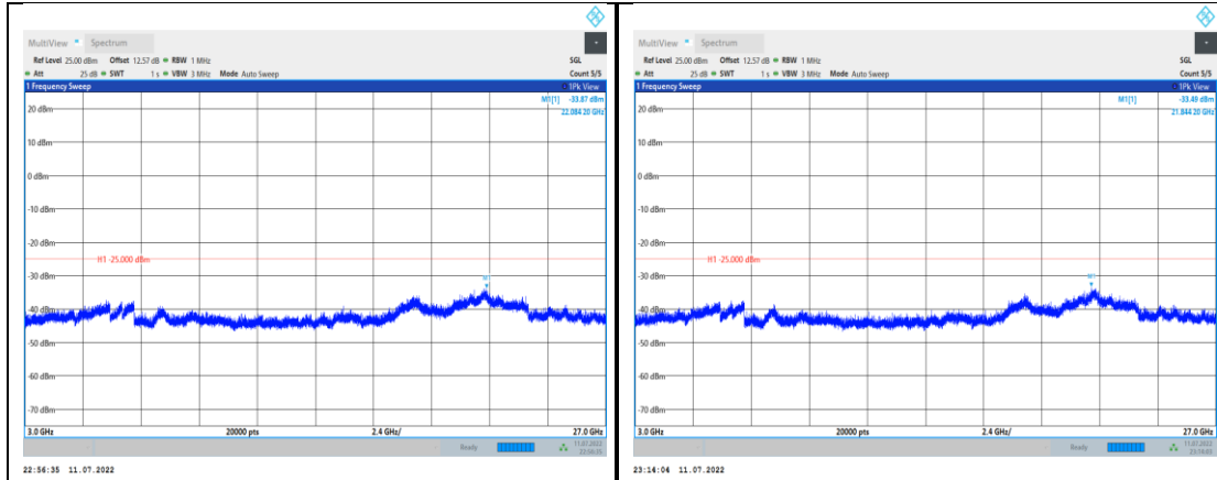
Band41-15MHz-QPSK-39725-1RB#0- Range3:3000~27000MHz
