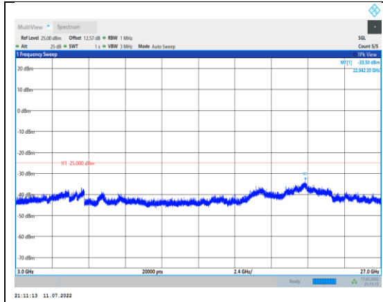
Band41-5MHz-QPSK-39675-1RB#0- Range3:3000~27000MHz
