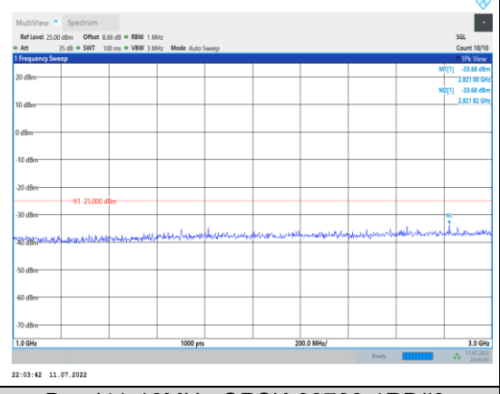
Band41-10MHz-QPSK-39700-1RB#0- Range2:1000~3000MHz
