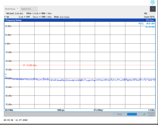
Band41-10MHz-QPSK-39700-1RB#0- Range1:30~1000MHz
