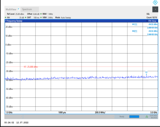
Band41-20MHz-QPSK-41490-1RB#0- Range2:1000~3000MHz
