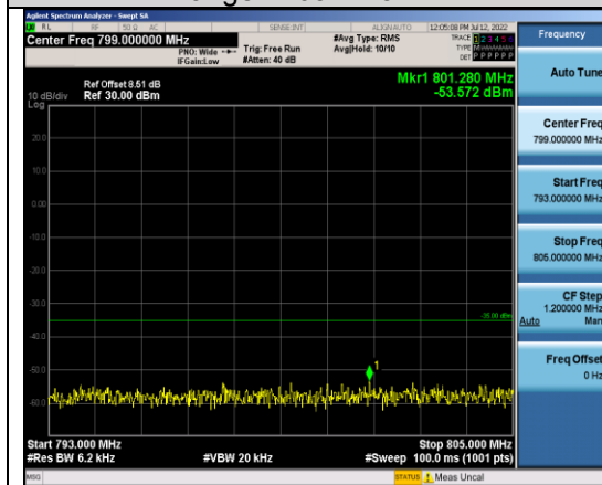
Band13-10MHz-QPSK-23230-1RB#0- Range5:793~805MHz
