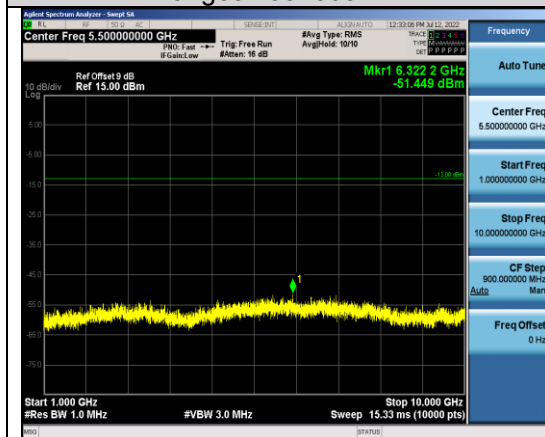
Band13-5MHz-QPSK-23230-1RB#0- Range2:1000~10000MHz
