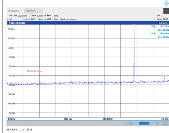
Band7-5MHz-QPSK-21425-1RB#0- Range2:1000~3000MHz
