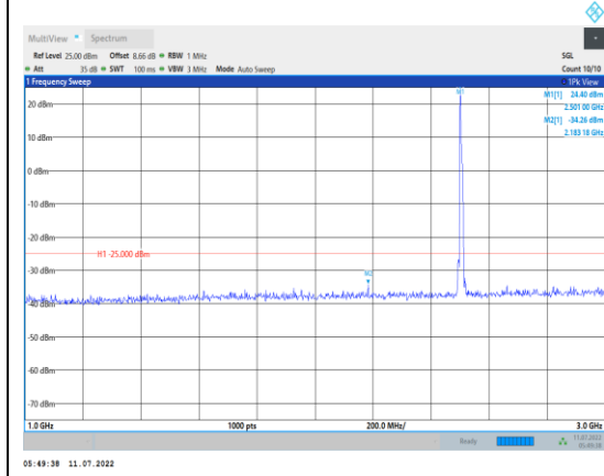
Band7-10MHz-QPSK-20800-1RB#0- Range2:1000~3000MHz
