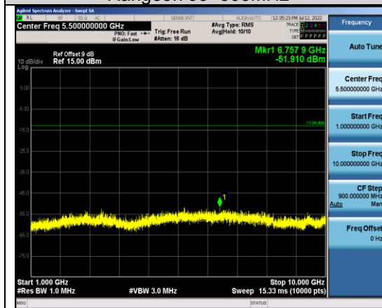
Band13-5MHz-QPSK-23255-1RB#0- Range2:1000~10000MHz
