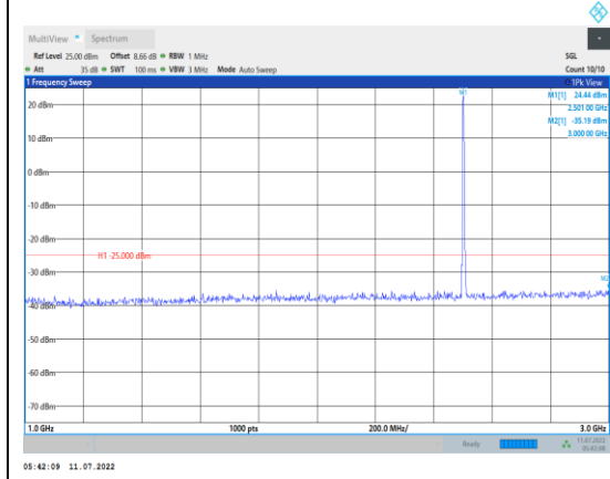
Band7-5MHz-QPSK-20775-1RB#0- Range2:1000~3000MHz
