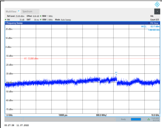
Band5-10MHz-QPSK-20525-1RB#0- Range2:1000~10000MHz
