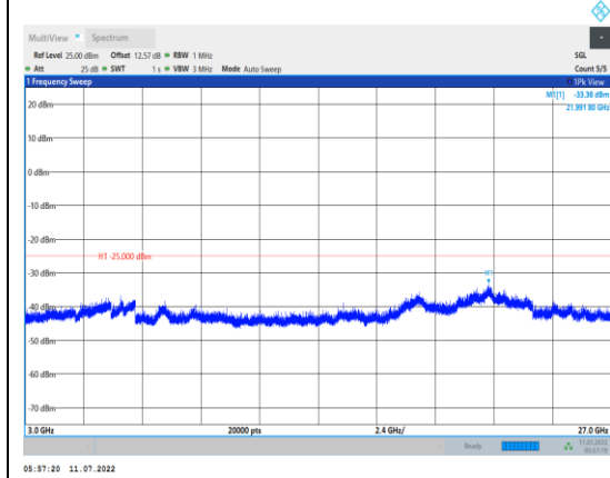
Band7-15MHz-QPSK-20825-1RB#0- Range3:3000~27000MHz
