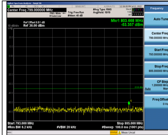
Band13-5MHz-QPSK-23255-1RB#0- Range5:793~805MHz
