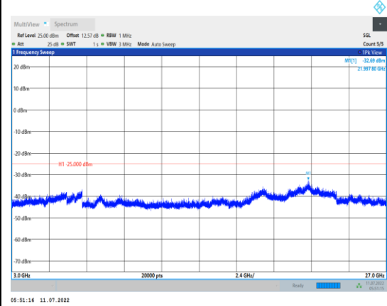
Band7-10MHz-QPSK-21100-1RB#0- Range3:3000~27000MHz
