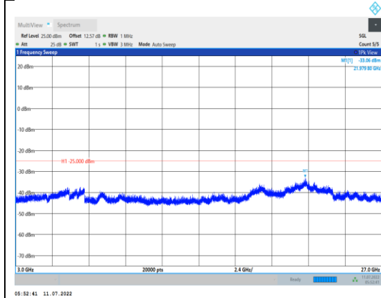
Band7-10MHz-QPSK-21400-1RB#0- Range3:3000~27000MHz
