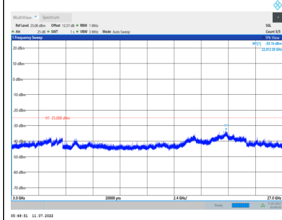
Band7-10MHz-QPSK-20800-1RB#0- Range3:3000~27000MHz
