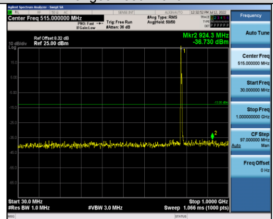
Band13-5MHz-QPSK-23230-1RB#0- Range1:30~1000MHz
