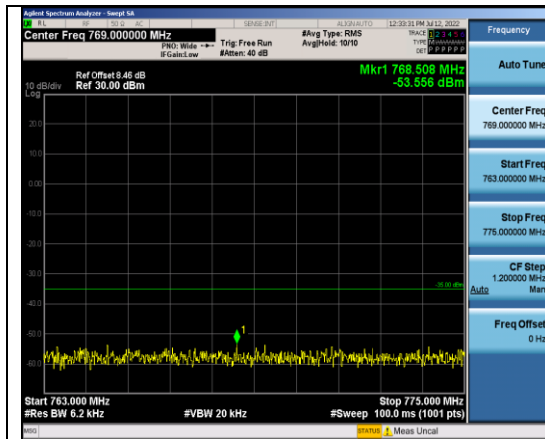
Band13-5MHz-QPSK-23230-1RB#0- Range4:763~775MHz
