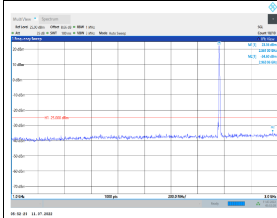
Band7-10MHz-QPSK-21400-1RB#0- Range2:1000~3000MHz
