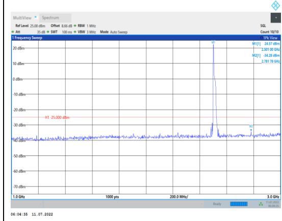
Band7-20MHz-QPSK-20850-1RB#0-Range2:1000~3000MHz
