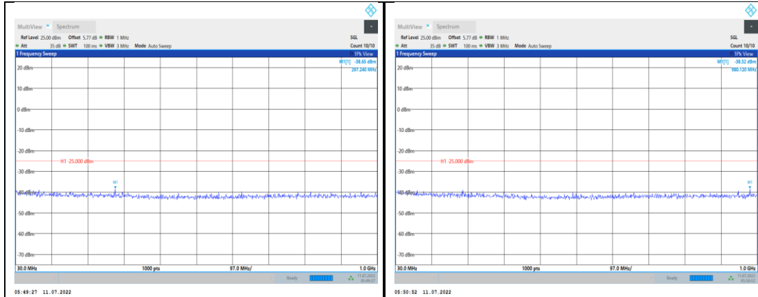
Band7-10MHz-QPSK-20800-1RB#0- Range1:30~1000MHz
