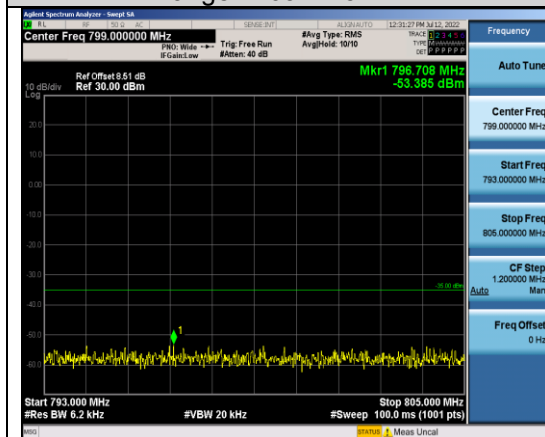
Band13-5MHz-QPSK-23205-1RB#0- Range5:793~805MHz
