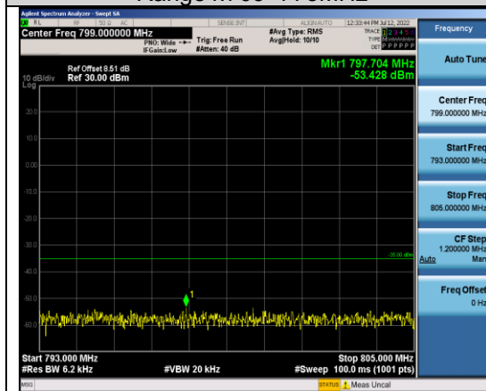
Band13-5MHz-QPSK-23230-1RB#0- Range5:793~805MHz
