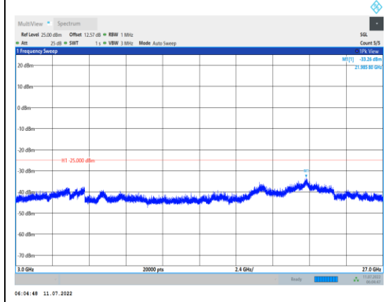
Band7-20MHz-QPSK-20850-1RB#0-Range3:3000~27000MHz
