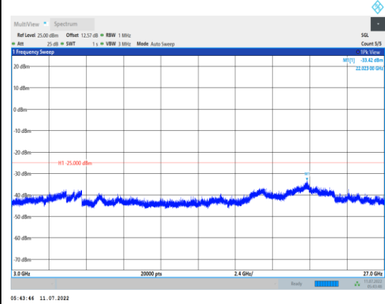
Band7-5MHz-QPSK-21100-1RB#0- Range3:3000~27000MHz
