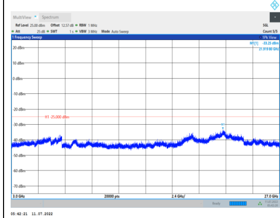
Band7-5MHz-QPSK-20775-1RB#0- Range3:3000~27000MHz
