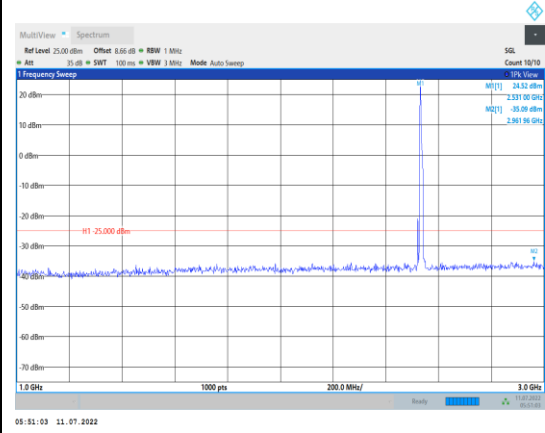
Band7-10MHz-QPSK-21100-1RB#0- Range2:1000~3000MHz
