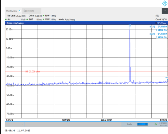
Band7-5MHz-QPSK-21100-1RB#0- Range2:1000~3000MHz
