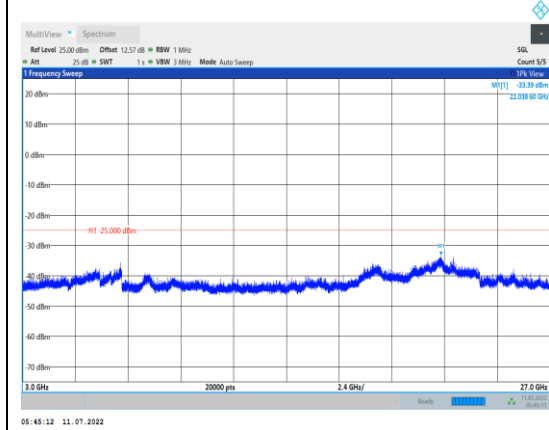
Band7-5MHz-QPSK-21425-1RB#0- Range3:3000~27000MHz
