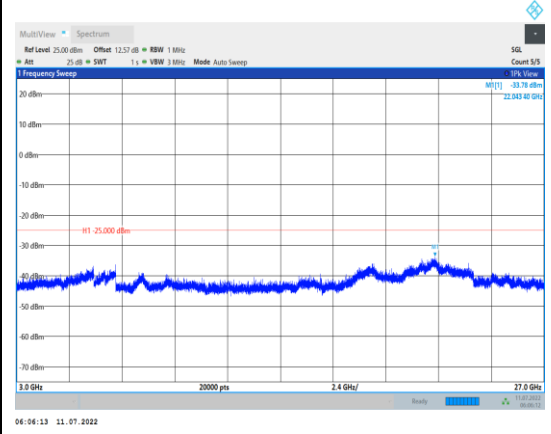
Band7-20MHz-QPSK-21100-1RB#0-Range3:3000~27000MHz
