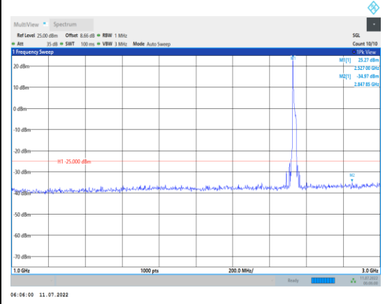
Band7-20MHz-QPSK-21100-1RB#0-Range2:1000~3000MHz
