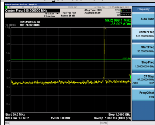
Band13-5MHz-QPSK-23255-1RB#0- Range1:30~1000MHz
