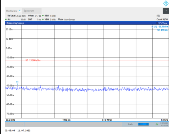
Band2-5MHz-QPSK-19175-1RB#0- Range1:30~1000MHz
