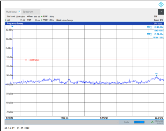
Band2-20MHz-16QAM-18900-1RB#0- Range2:1000~20000MHz
