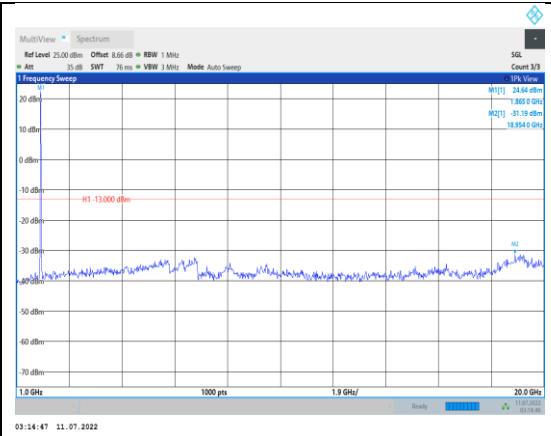
Band2-20MHz-QPSK-18900-1RB#0- Range2:1000~20000MHz
