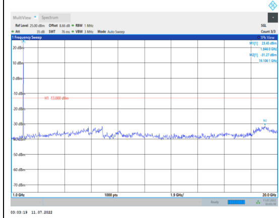
Band2-5MHz-QPSK-18625-1RB#0- Range2:1000~20000MHz
