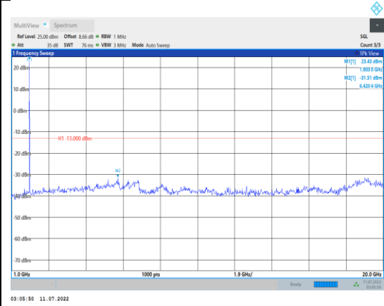
Band2-5MHz-16QAM-19175-1RB#0- Range2:1000~20000MHz
