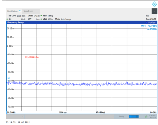
Band2-20MHz-QPSK-18700-1RB#0- Range1:30~1000MHz
