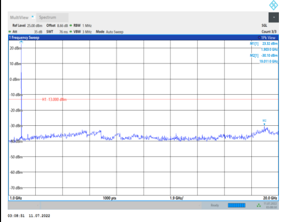
Band2-10MHz-QPSK-19150-1RB#0- Range2:1000~20000MHz
