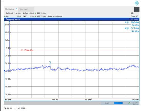
Band4-15MHz-QPSK-20325-1RB#0- Range2:1000~20000MHz
