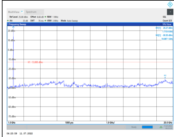
Band4-15MHz-QPSK-20025-1RB#0- Range2:1000~20000MHz
