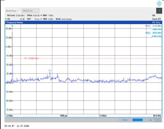
Band2-20MHz-QPSK-19100-1RB#0- Range2:1000~20000MHz
