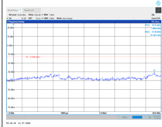
Band2-20MHz-16QAM-18700-1RB#0- Range2:1000~20000MHz
