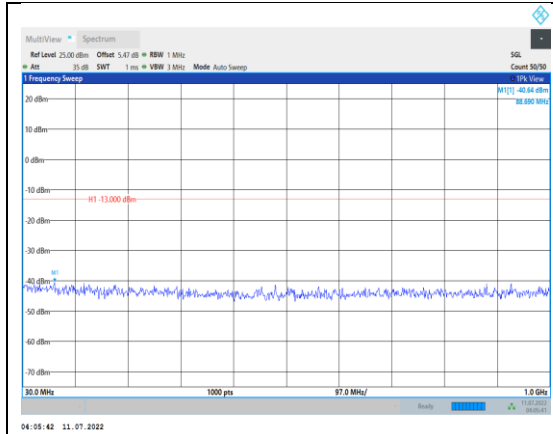
Band4-3MHz-QPSK-19965-1RB#0- Range1:30~1000MHz
