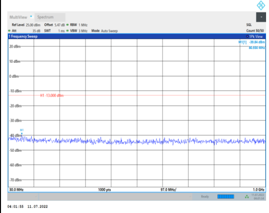
Band4-1.4MHz-QPSK-20393-1RB#0- Range1:30~1000MHz
