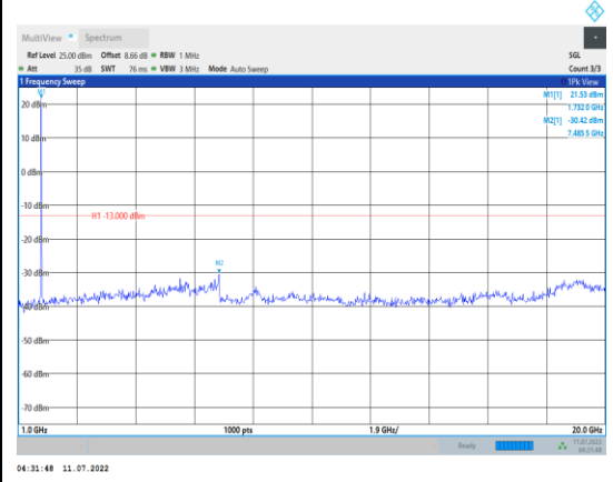
Band4-20MHz-QPSK-20300-1RB#0- Range2:1000~20000MHz
