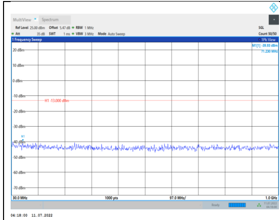
Band4-10MHz-QPSK-20000-1RB#0- Range1:30~1000MHz
