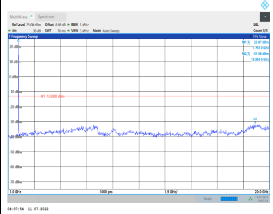
Band4-3MHz-QPSK-20385-1RB#0- Range2:1000~20000MHz
