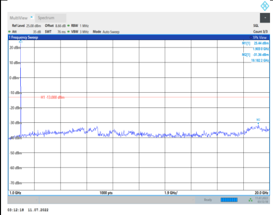
Band2-15MHz-QPSK-19125-1RB#0- Range2:1000~20000MHz
