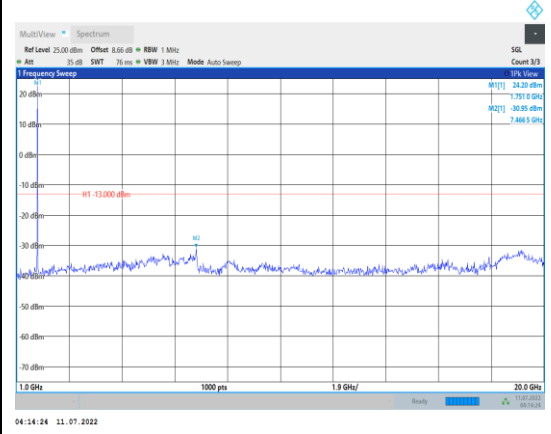
Band4-5MHz-QPSK-20375-1RB#0- Range2:1000~20000MHz
