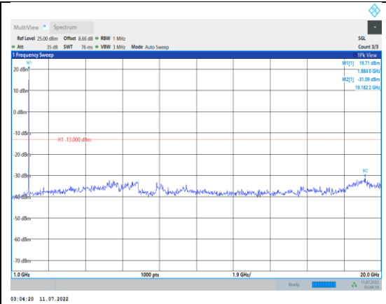
Band2-5MHz-QPSK-18900-1RB#0- Range2:1000~20000MHz
