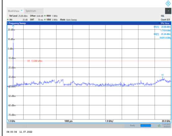
Band4-1.4MHz-QPSK-19957-1RB#0- Range2:1000~20000MHz
