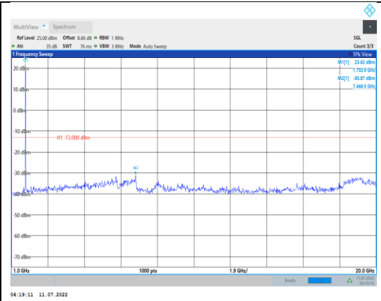
Band4-10MHz-QPSK-20175-1RB#0- Range2:1000~20000MHz
