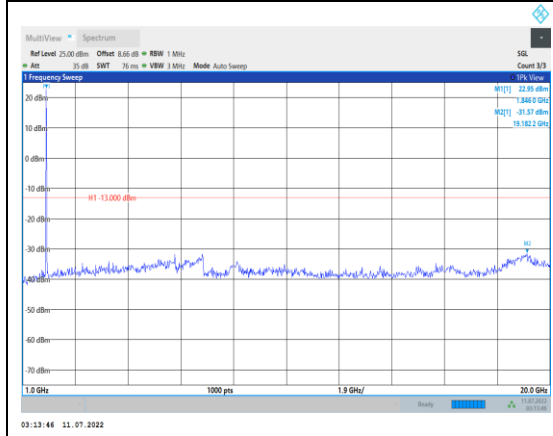
Band2-20MHz-QPSK-18700-1RB#0- Range2:1000~20000MHz
