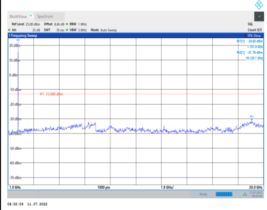
Band4-1.4MHz-QPSK-20393-1RB#0- Range2:1000~20000MHz
