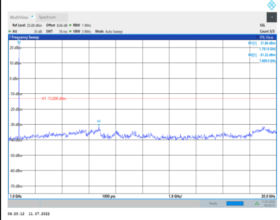
Band4-10MHz-QPSK-20350-1RB#0- Range2:1000~20000MHz
