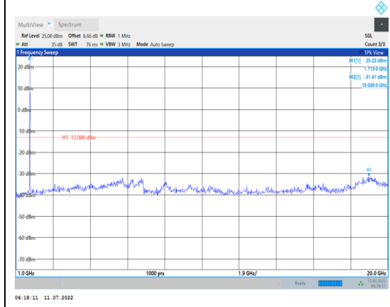
Band4-10MHz-QPSK-20000-1RB#0- Range2:1000~20000MHz
