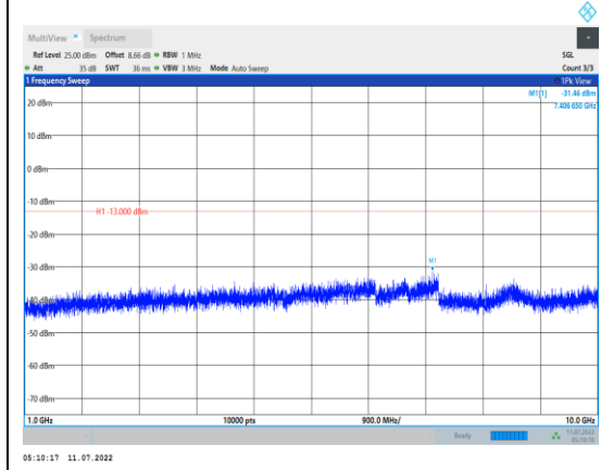
Band5-5MHz-QPSK-20425-1RB#0- Range2:1000~10000MHz
