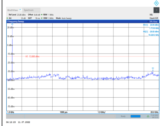
Band4-5MHz-QPSK-19975-1RB#0- Range2:1000~20000MHz
