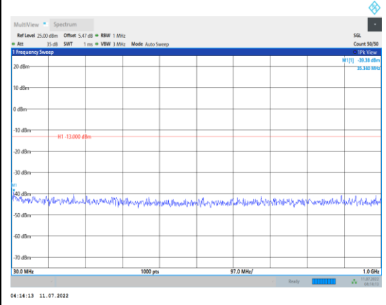
Band4-5MHz-QPSK-20375-1RB#0- Range1:30~1000MHz
