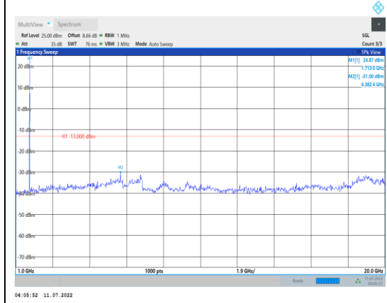
Band4-3MHz-QPSK-19965-1RB#0- Range2:1000~20000MHz
