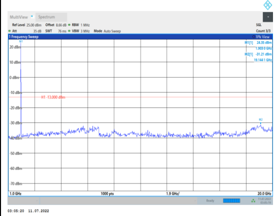
Band2-5MHz-QPSK-19175-1RB#0- Range2:1000~20000MHz
