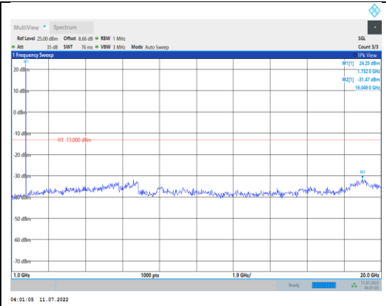
Band4-1.4MHz-QPSK-20175-1RB#0- Range2:1000~20000MHz
