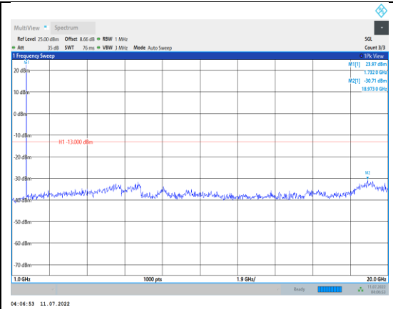
Band4-3MHz-QPSK-20175-1RB#0- Range2:1000~20000MHz
