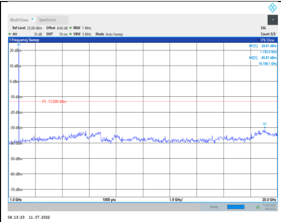
Band4-5MHz-QPSK-20175-1RB#0- Range2:1000~20000MHz
