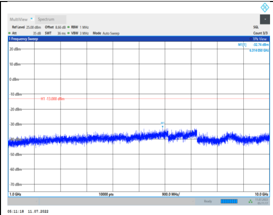
Band5-5MHz-QPSK-20525-1RB#0- Range2:1000~10000MHz
