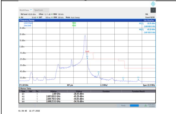
Band41-5MHz-16QAM-41565-1RB#24
