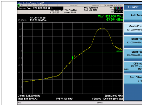
Band5-10MHz-QPSK-20450-1RB#0
