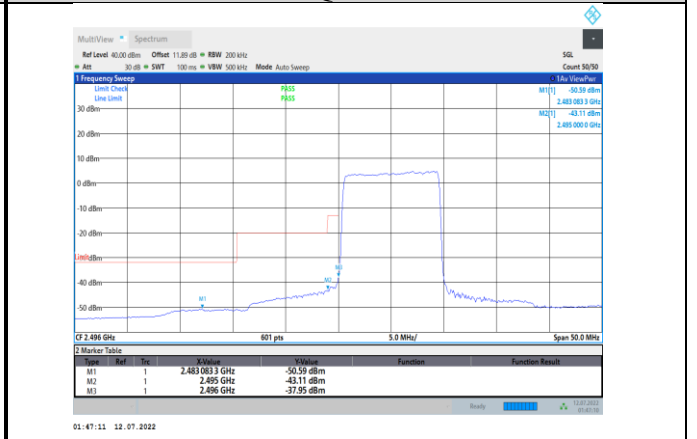
Band41-10MHz-QPSK-39700-50RB#0
