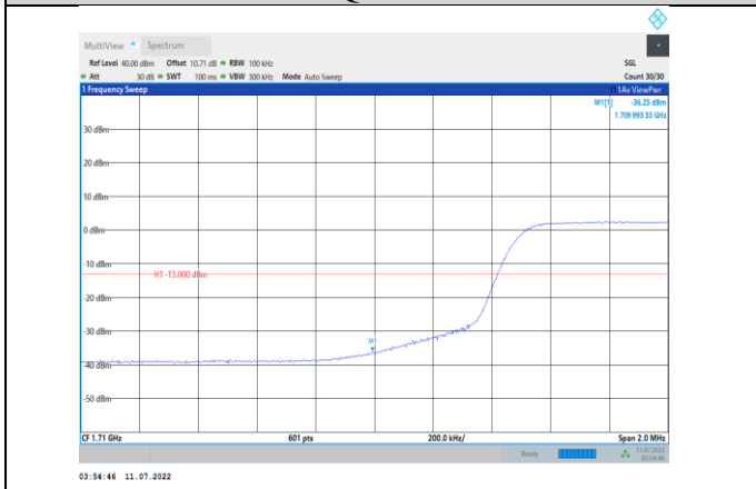
Band4-10MHz-QPSK-20000-50RB#0
