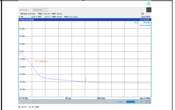
Band2-20MHz-16QAM-19100-100RB#0
