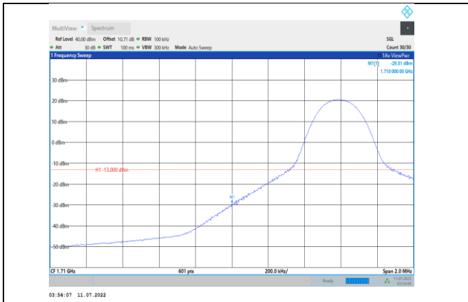
Band4-10MHz-QPSK-20000-1RB#0
