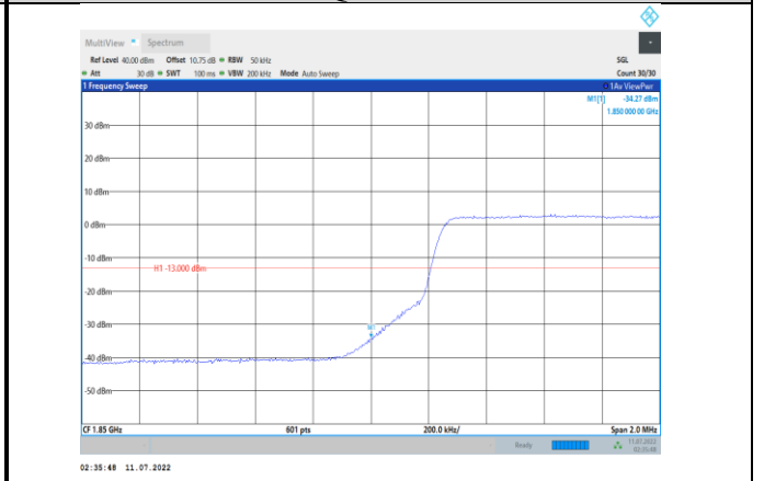
Band2-5MHz-QPSK-18625-25RB#0
