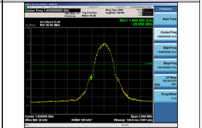
EGPRS1900-512-2
