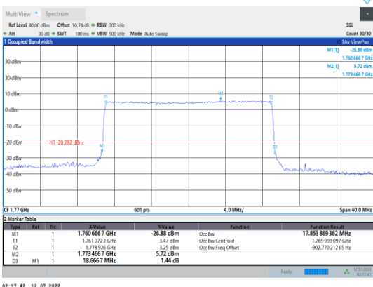
Band66-20MHz-QPSK-132572-100RB#0
