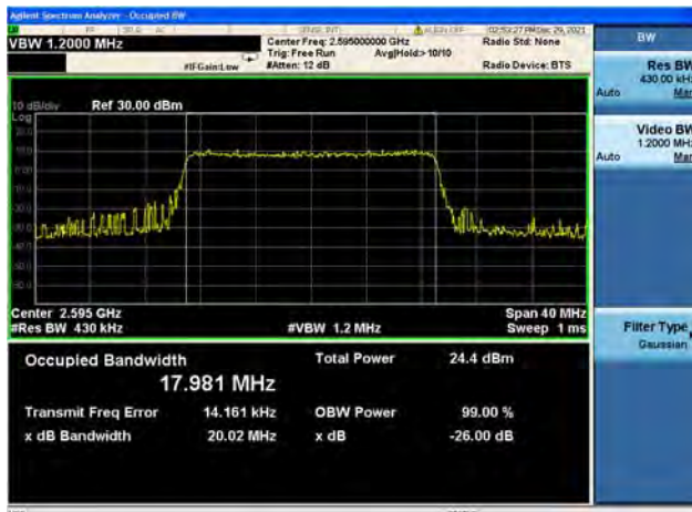
Band41 / 20MHz / Mid CH / 64QAM
