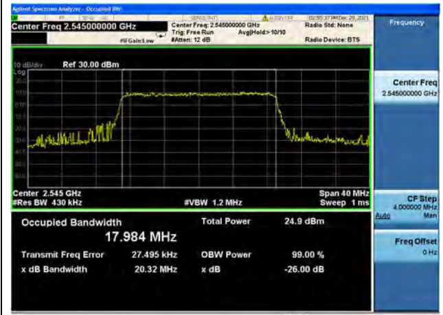
Band41 / 20MHz / Low CH / 64QAM
