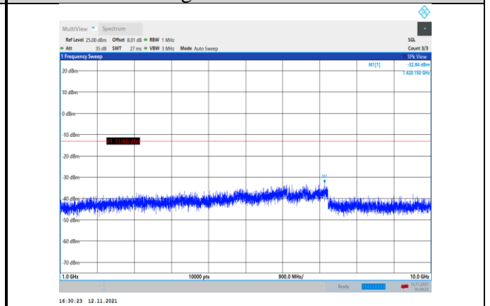
Band12-10MHz-QPSK-23130-1RB#0- Range2:1000~10000MHz
