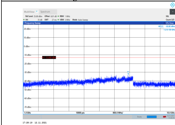
Band26-5MHz-QPSK-26715-1RB#0- Range2:1000~10000MHz
