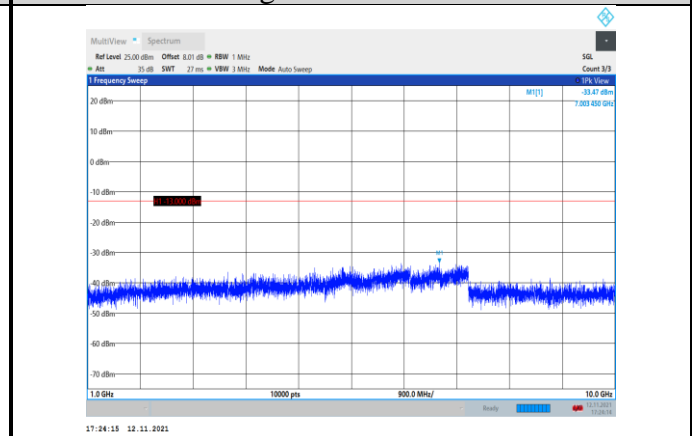
Band26-3MHz-QPSK-26775-1RB#0- Range2:1000~10000MHz
