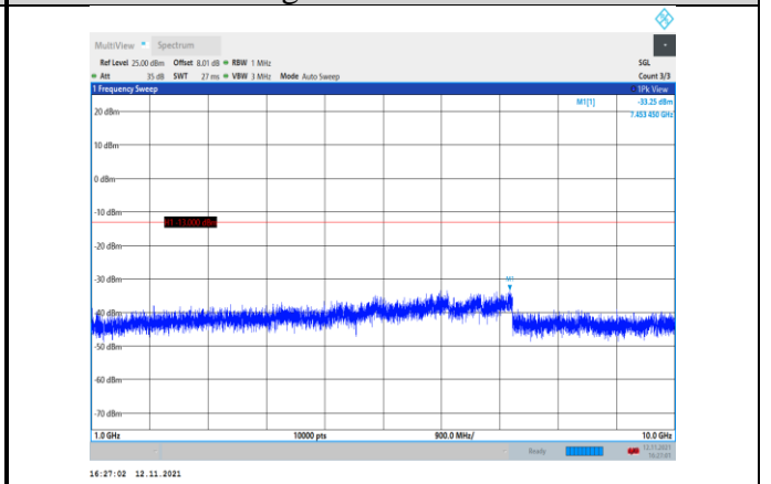
Band12-5MHz-QPSK-23155-1RB#0- Range2:1000~10000MHz
