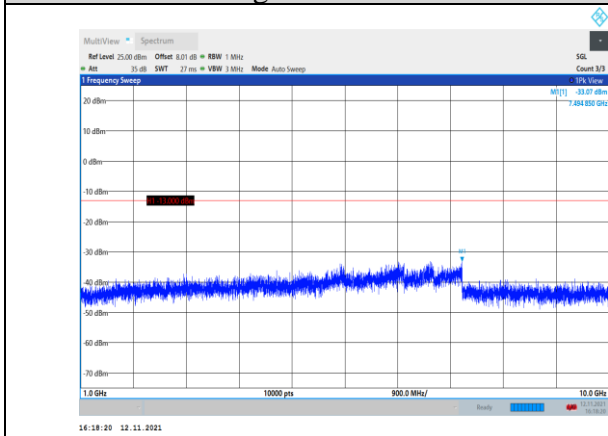
Band12-1.4MHz-QPSK-23017-1RB#0- Range2:1000~10000MHz
