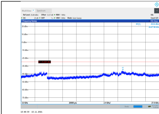
Band38-5MHz-QPSK-38225-1RB#0- Range3:3000~27000MHz
