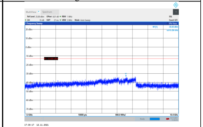
Band26-5MHz-QPSK-26765-1RB#0- Range2:1000~10000MHz
