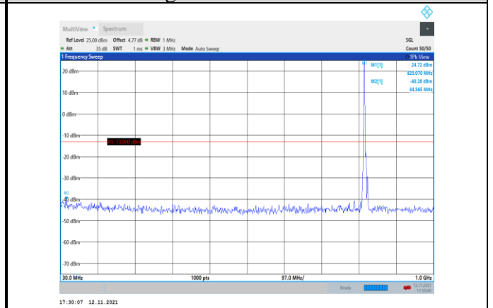
Band26-5MHz-QPSK-26765-1RB#0- Range1:30~1000MHz
