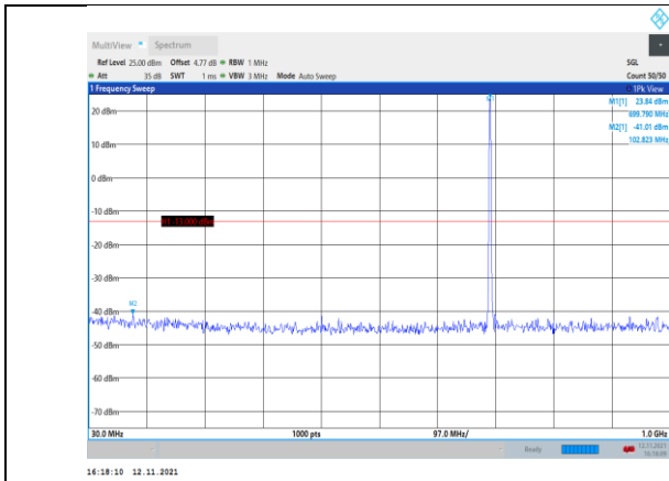
Band12-1.4MHz-QPSK-23017-1RB#0- Range1:30~1000MHz
