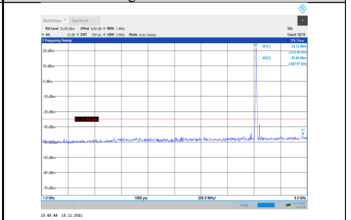
Band38-5MHz-QPSK-38225-1RB#0- Range2:1000~3000MHz
