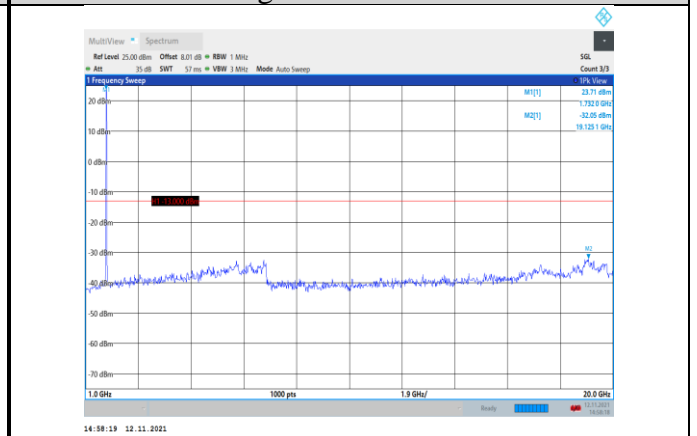
Band4-15MHz-QPSK-20325-1RB#0- Range2:1000~20000MHz
