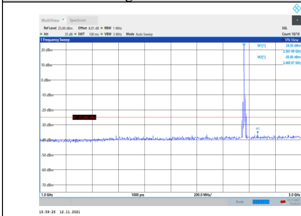
Band7-10MHz-QPSK-21400-1RB#0- Range2:1000~3000MHz
