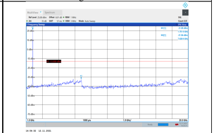
Band4-10MHz-QPSK-20350-1RB#0- Range2:1000~20000MHz
