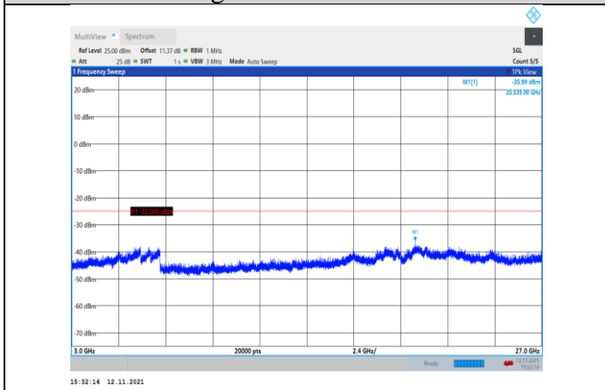
Band7-5MHz-QPSK-21425-1RB#0- Range3:3000~27000MHz
