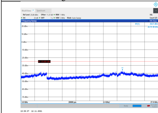
Band7-10MHz-QPSK-21400-1RB#0- Range3:3000~27000MHz
