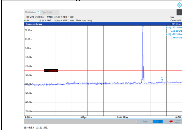
Band7-15MHz-QPSK-20825-1RB#0- Range2:1000~3000MHz
