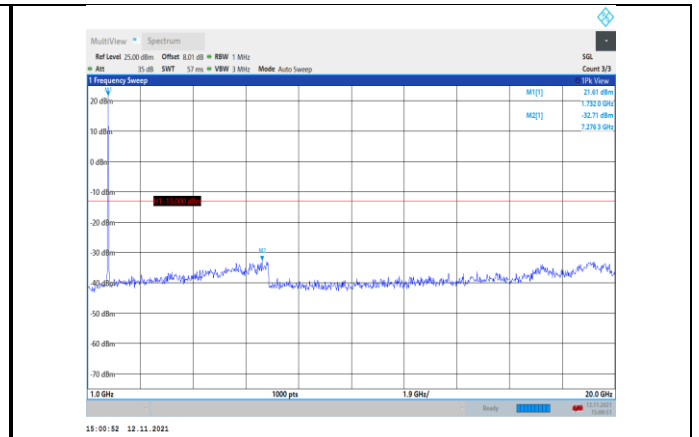
Band4-20MHz-QPSK-20175-1RB#0- Range2:1000~20000MHz
