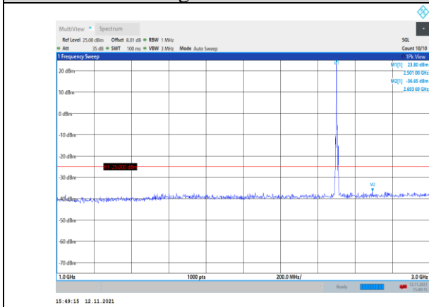
Band7-5MHz-QPSK-20775-1RB#0- Range2:1000~3000MHz
