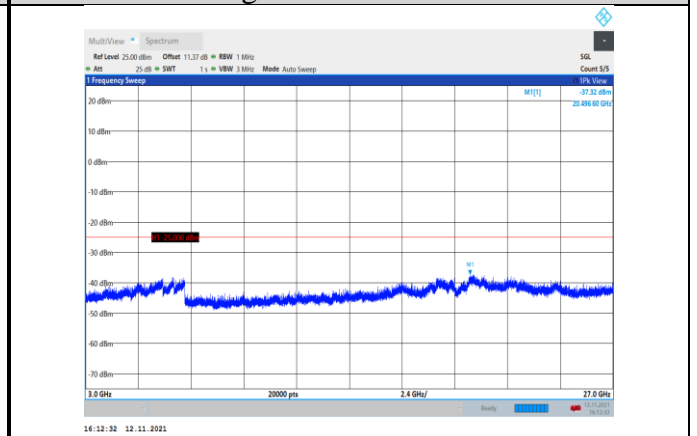
Band7-20MHz-QPSK-21100-1RB#0- Range3:3000~27000MHz
