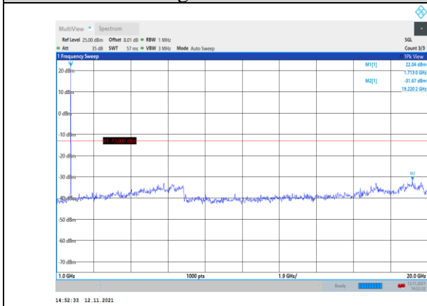
Band4-10MHz-QPSK-20000-1RB#0- Range2:1000~20000MHz
