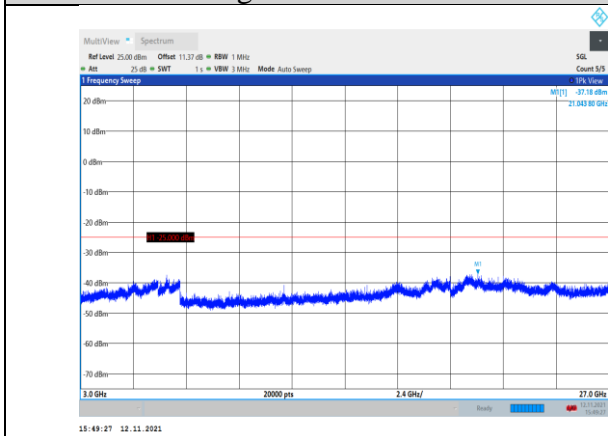
Band7-5MHz-QPSK-20775-1RB#0- Range3:3000~27000MHz
