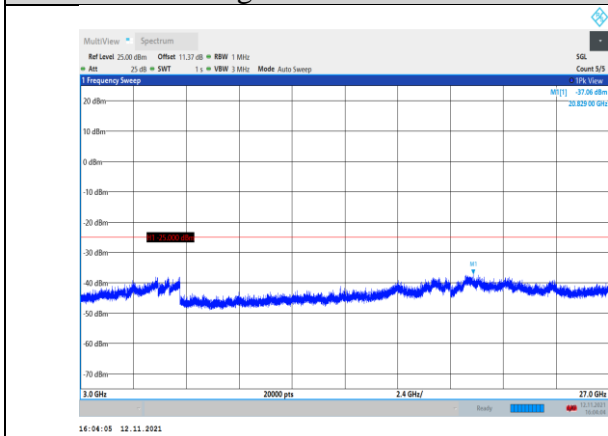
Band7-15MHz-QPSK-20825-1RB#0- Range3:3000~27000MHz
