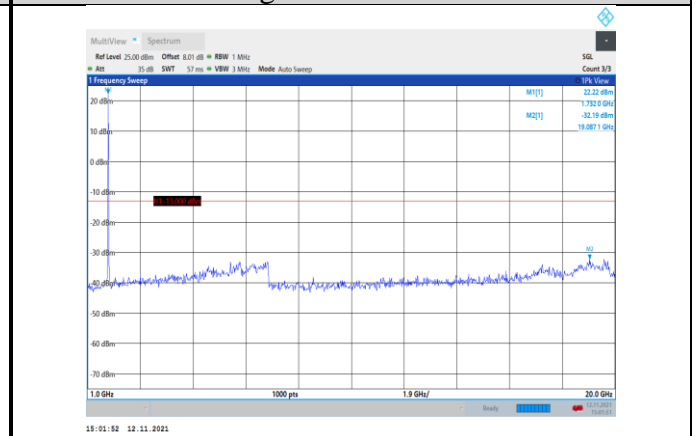
Band4-20MHz-QPSK-20300-1RB#0- Range2:1000~20000MHz
