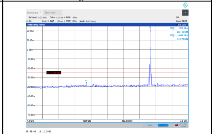
Band7-10MHz-QPSK-21100-1RB#0- Range2:1000~3000MHz
