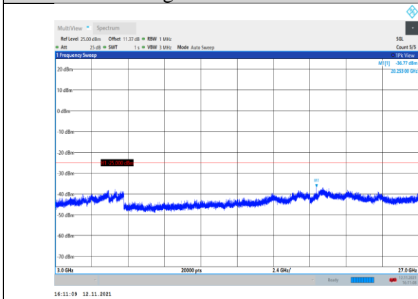
Band7-20MHz-QPSK-20850-1RB#0- Range3:3000~27000MHz
