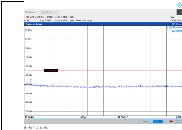
Band7-10MHz-QPSK-20800-1RB#0- Range1:30~1000MHz
