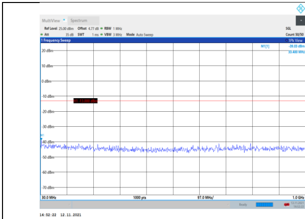
Band4-10MHz-QPSK-20000-1RB#0- Range1:30~1000MHz
