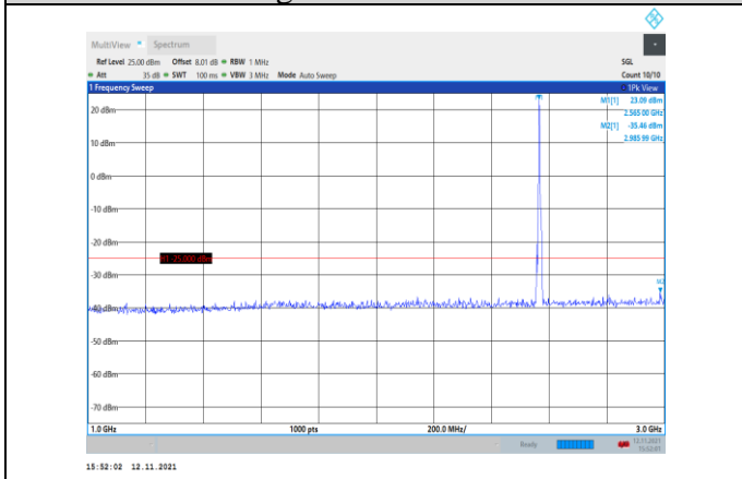
Band7-5MHz-QPSK-21425-1RB#0- Range2:1000~3000MHz
