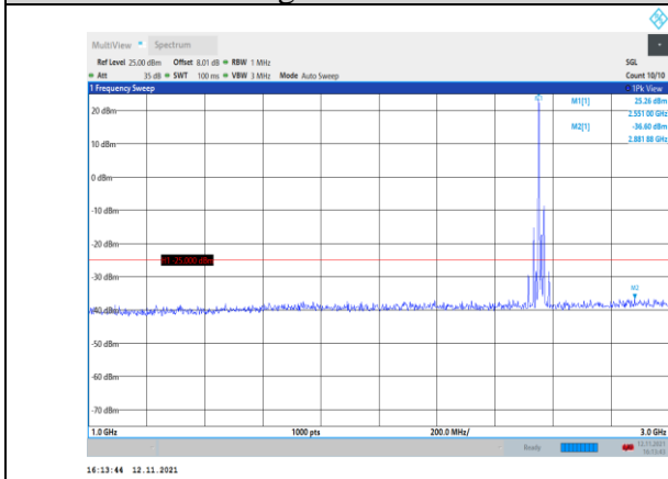
Band7-20MHz-QPSK-21350-1RB#0- Range2:1000~3000MHz
