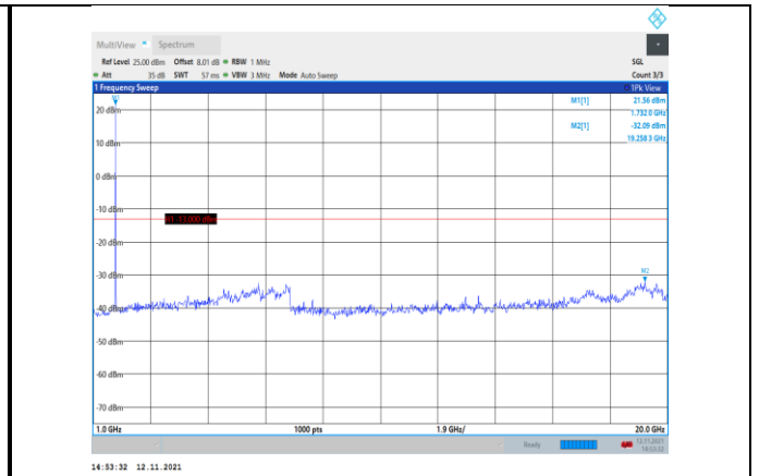
Band4-10MHz-QPSK-20175-1RB#0- Range2:1000~20000MHz
