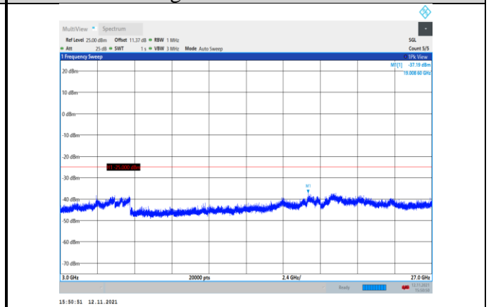
Band7-5MHz-QPSK-21100-1RB#0- Range3:3000~27000MHz
