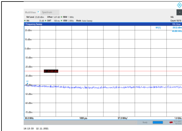
Band7-20MHz-QPSK-21350-1RB#0- Range1:30~1000MHz
