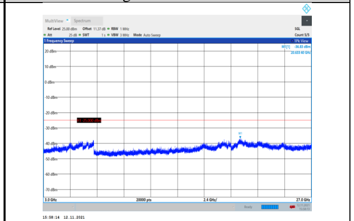
Band7-10MHz-QPSK-21100-1RB#0- Range3:3000~27000MHz
