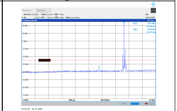
Band7-20MHz-QPSK-21100-1RB#0- Range2:1000~3000MHz
