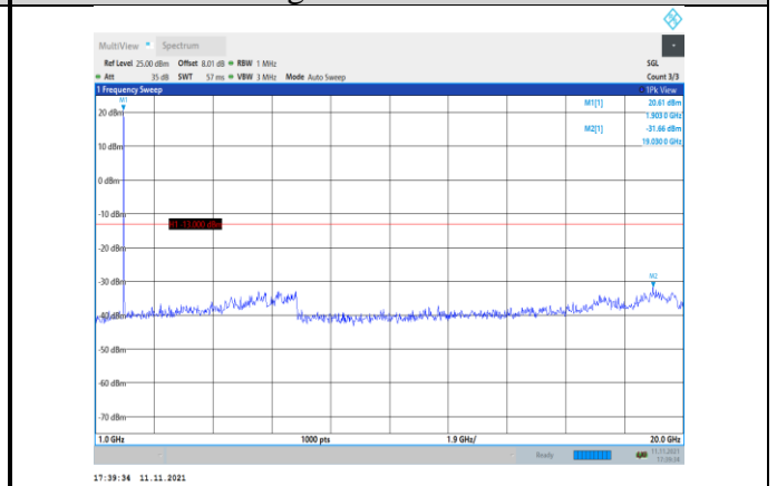
Band2-5MHz-QPSK-19175-1RB#0- Range2:1000~20000MHz
