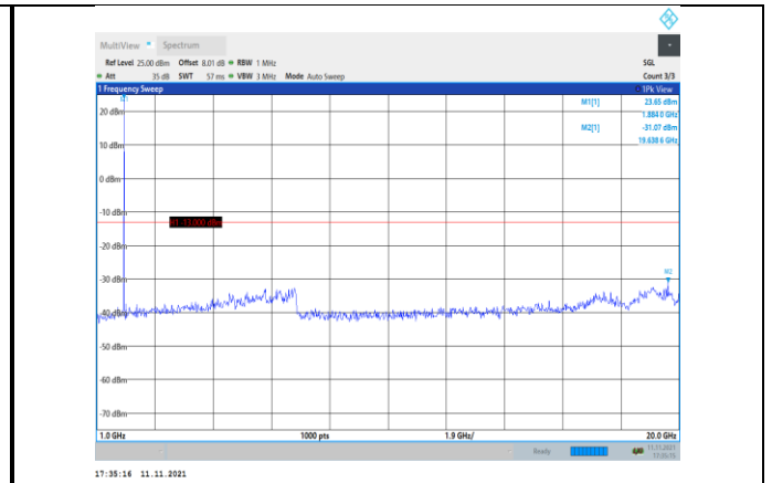
Band2-3MHz-QPSK-18900-1RB#0- Range2:1000~20000MHz
