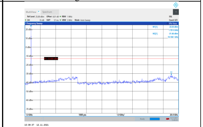
Band4-1.4MHz-QPSK-20393-1RB#0- Range2:1000~20000MHz
