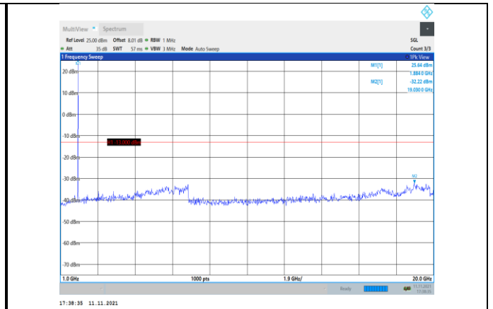
Band2-5MHz-QPSK-18900-1RB#0- Range2:1000~20000MHz
