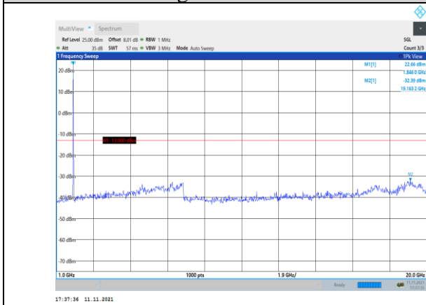
Band2-5MHz-QPSK-18625-1RB#0- Range2:1000~20000MHz
