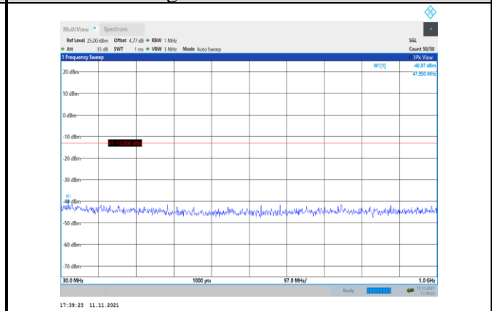
Band2-5MHz-QPSK-19175-1RB#0- Range1:30~1000MHz
