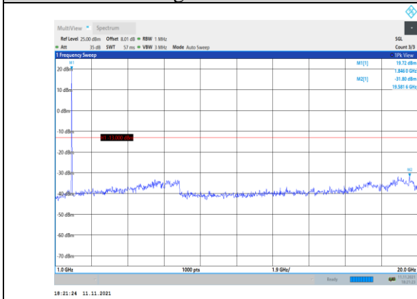
Band2-20MHz-16QAM-18700-1RB#0- Range2:1000~20000MHz
