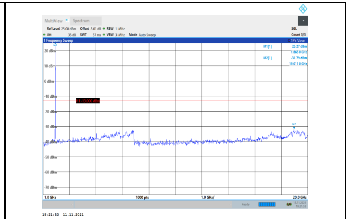
Band2-20MHz-QPSK-18900-1RB#0- Range2:1000~20000MHz
