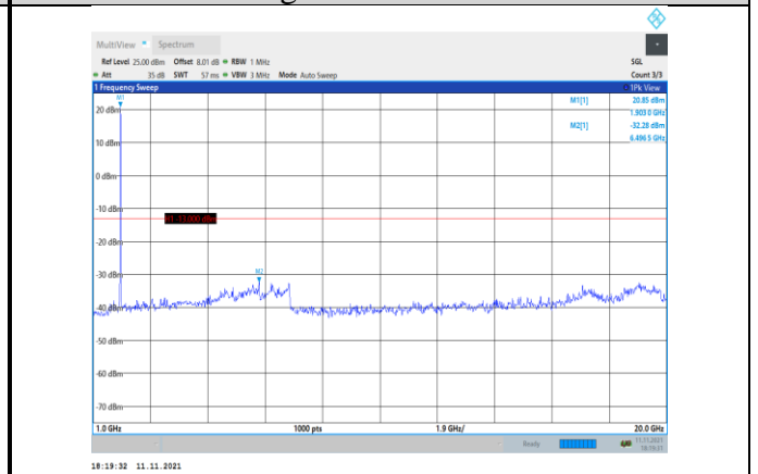
Band2-15MHz-QPSK-19125-1RB#0- Range2:1000~20000MHz
