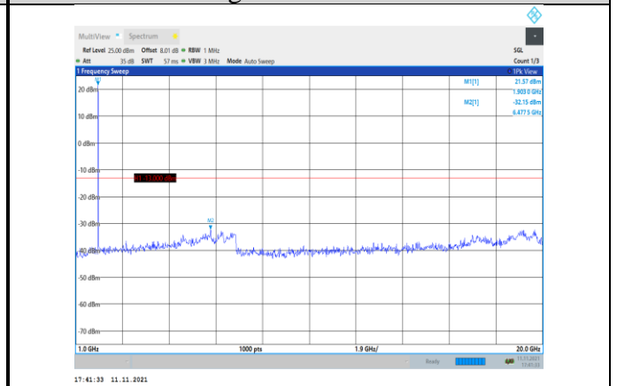
Band2-5MHz-16QAM-19175-1RB#0- Range2:1000~20000MHz
