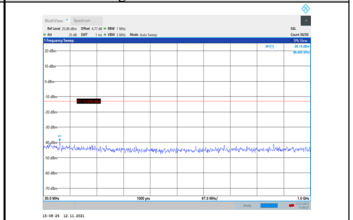
Band4-1.4MHz-QPSK-20393-1RB#0- Range1:30~1000MHz
