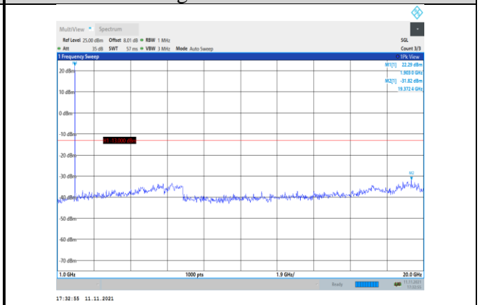
Band2-1.4MHz-QPSK-19193-1RB#0- Range2:1000~20000MHz
