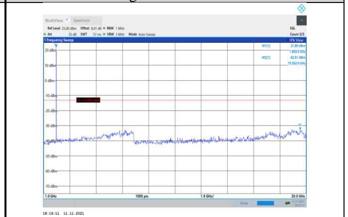
Band2-10MHz-QPSK-19150-1RB#0- Range2:1000~20000MHz
