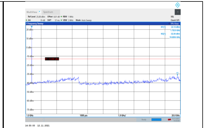
Band4-5MHz-QPSK-20175-1RB#0- Range2:1000~20000MHz
