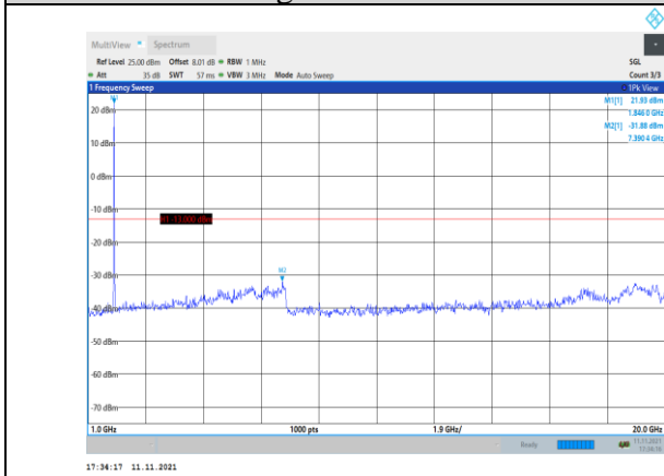
Band2-3MHz-QPSK-18615-1RB#0- Range2:1000~20000MHz
