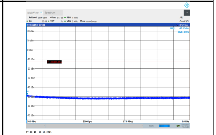
GSM1900-810-0-30~1000MHz
