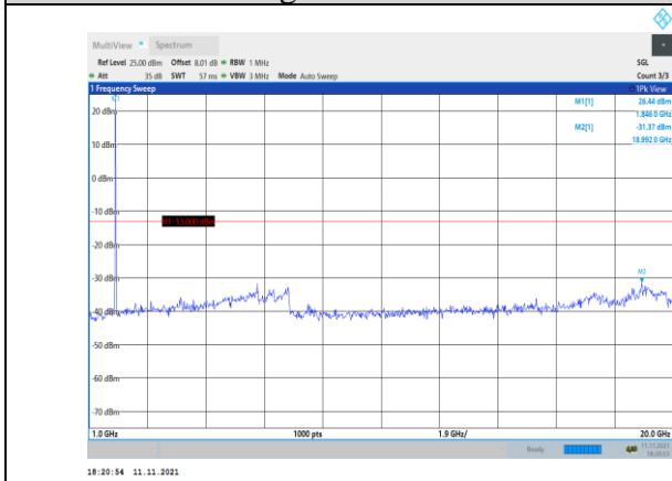
Band2-20MHz-QPSK-18700-1RB#0- Range2:1000~20000MHz
