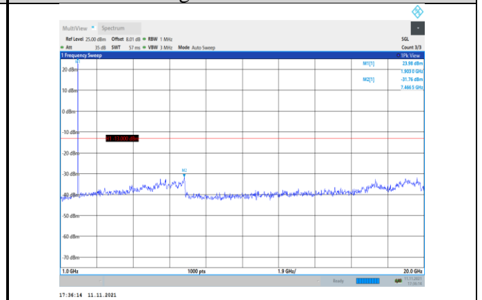
Band2-3MHz-QPSK-19185-1RB#0- Range2:1000~20000MHz
