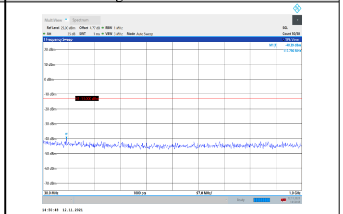
Band4-5MHz-QPSK-20375-1RB#0- Range1:30~1000MHz
