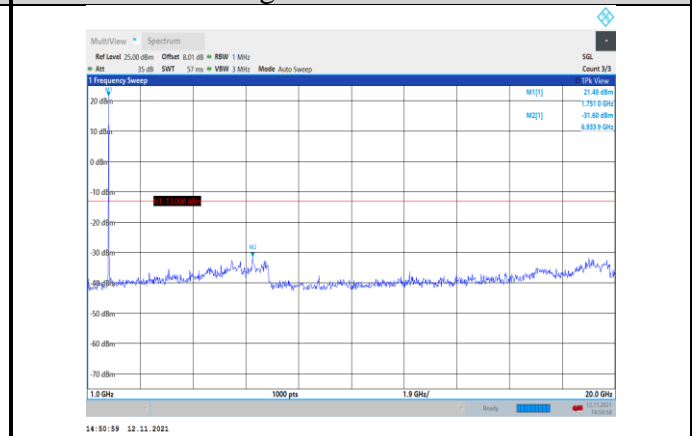
Band4-5MHz-QPSK-20375-1RB#0- Range2:1000~20000MHz
