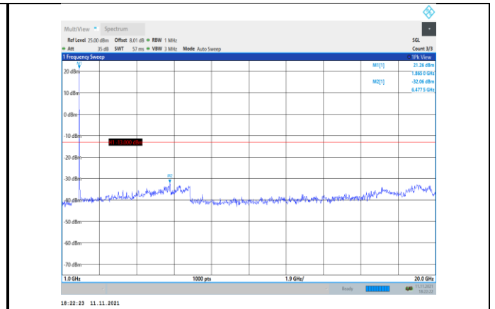
Band2-20MHz-16QAM-18900-1RB#0- Range2:1000~20000MHz
