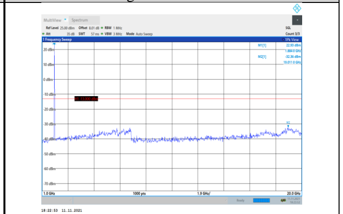
Band2-20MHz-QPSK-19100-1RB#0- Range2:1000~20000MHz
