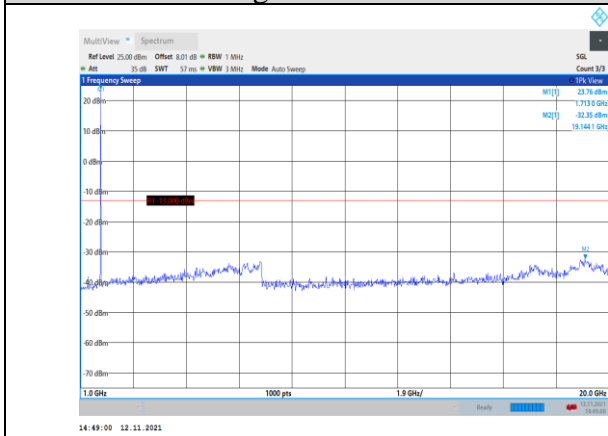
Band4-5MHz-QPSK-19975-1RB#0- Range2:1000~20000MHz
