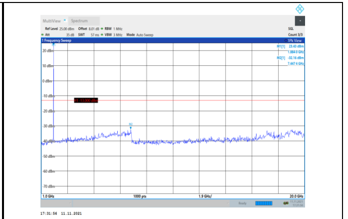
Band2-1.4MHz-QPSK-18900-1RB#0- Range2:1000~20000MHz
