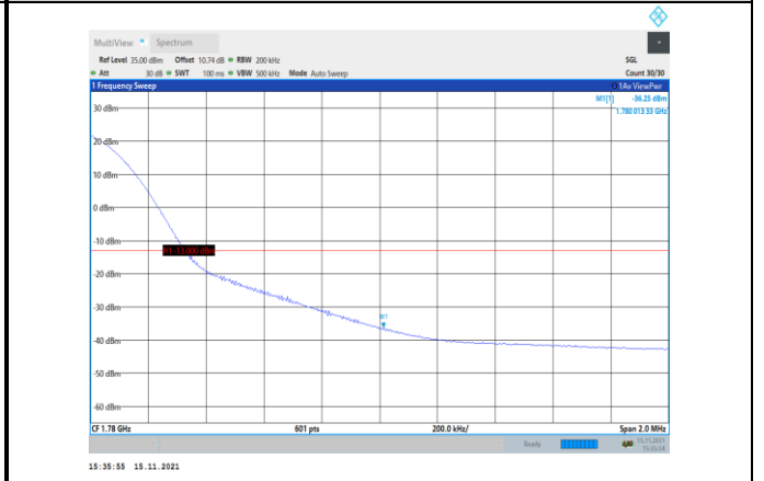
Band66-20MHz-QPSK-132572-1RB#99
