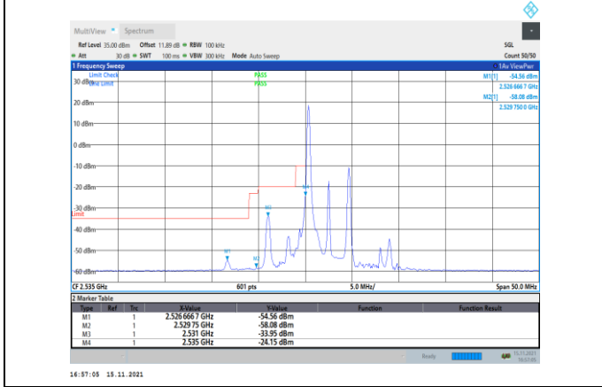
Band41-5MHz-QPSK-40065-1RB#0
