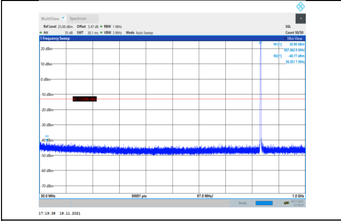
GSM850-190-3-30~1000MHz
