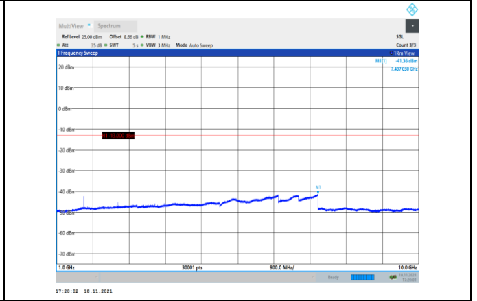
GSM850-190-3-1000~10000MHz
