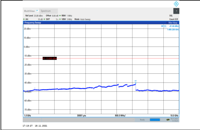
GSM850-128-3-1000~10000MHz
