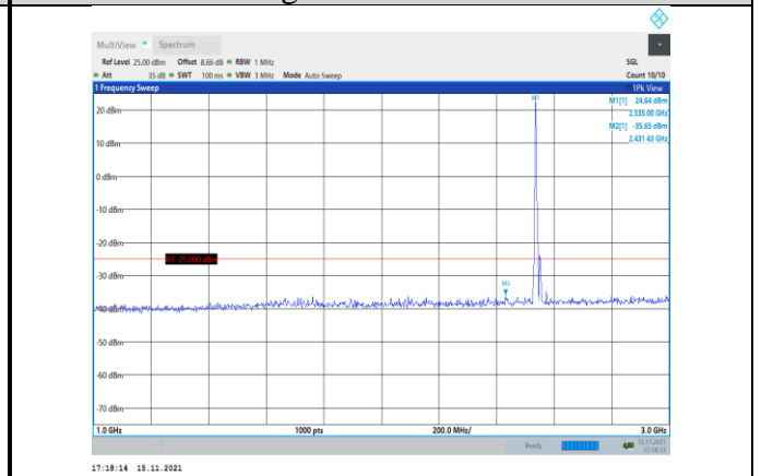
Band41-5MHz-QPSK-40065-1RB#0-Range2:1000~3000MHz
