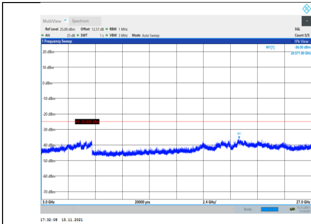
Band41-20MHz-QPSK-40140-1RB#0- Range3:3000~27000MHz
