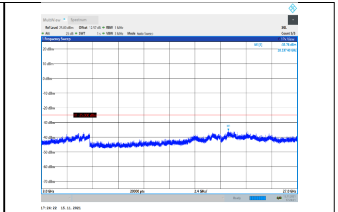
Band41-10MHz-QPSK-40590-1RB#0- Range3:3000~27000MHz
