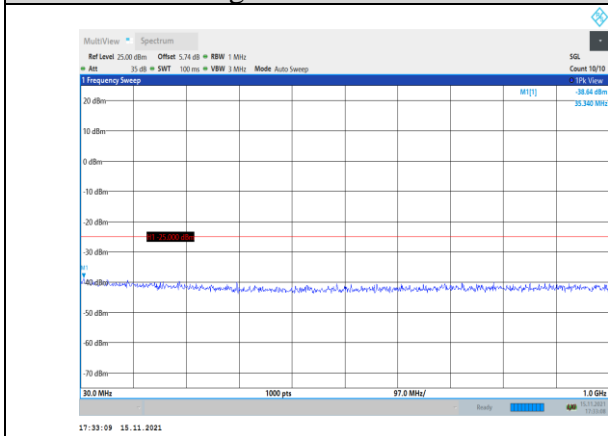
Band41-20MHz-QPSK-40590-1RB#0- Range1:30~1000MHz
