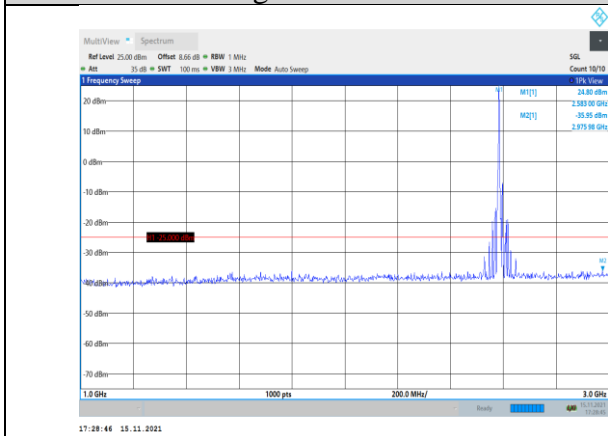
Band41-15MHz-QPSK-40590-1RB#0- Range2:1000~3000MHz
