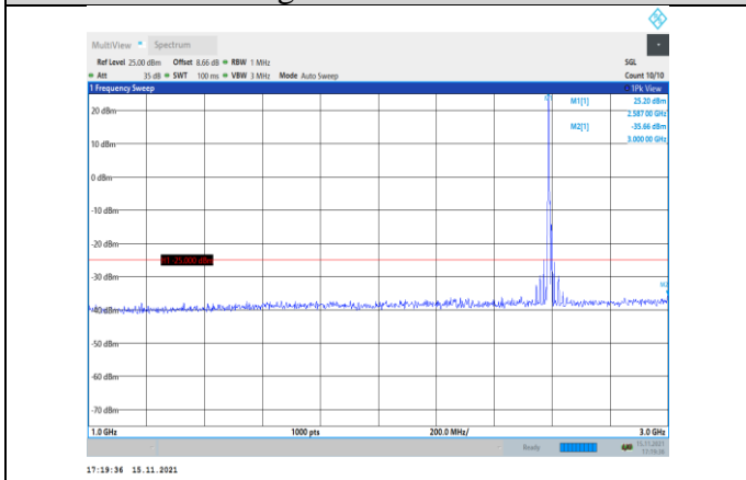
Band41-5MHz-QPSK-40590-1RB#0- Range2:1000~3000MHz
