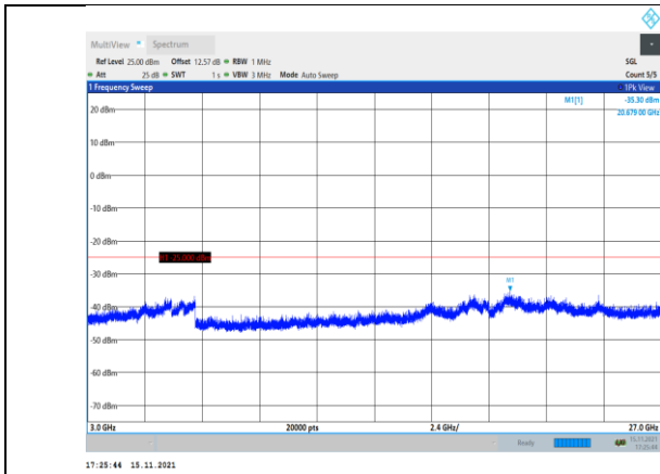
Band41-10MHz-QPSK-41190-1RB#0- Range3:3000~27000MHz
