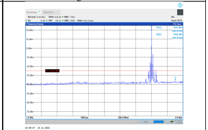
Band38-20MHz-QPSK-38150-1RB#0- Range2:1000~3000MHz
