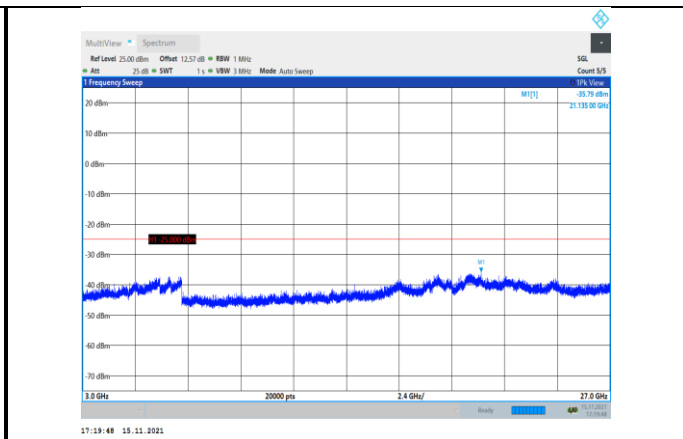
Band41-5MHz-QPSK-40590-1RB#0- Range3:3000~27000MHz
