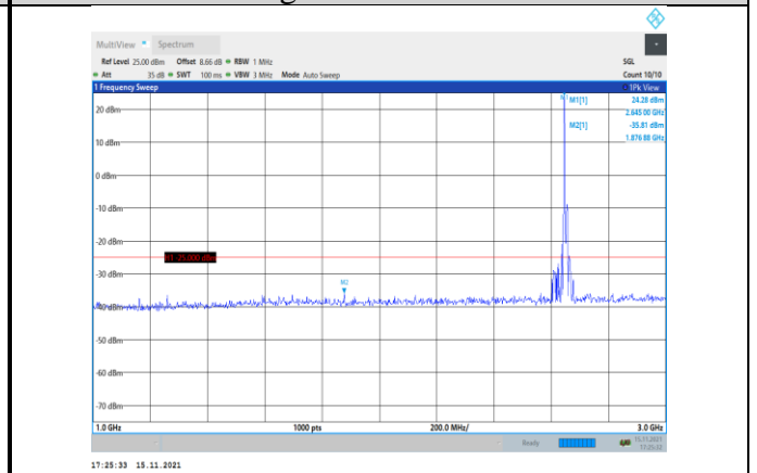
Band41-10MHz-QPSK-41190-1RB#0- Range2:1000~3000MHz
