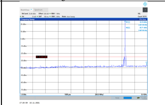
Band41-5MHz-QPSK-41215-1RB#0- Range2:1000~3000MHz
