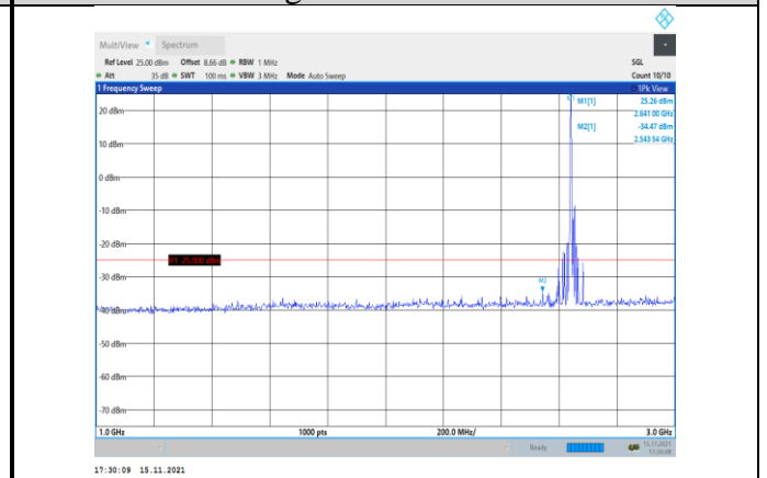
Band41-15MHz-QPSK-41165-1RB#0- Range2:1000~3000MHz
