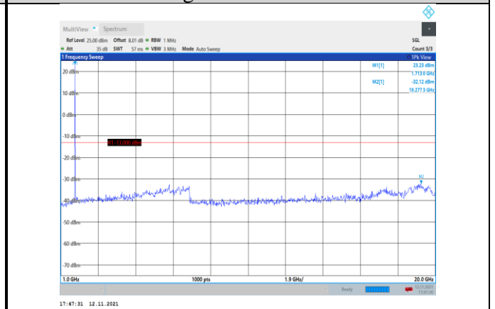
Band66-3MHz-QPSK-131987-1RB#0- Range2:1000~20000MHz
