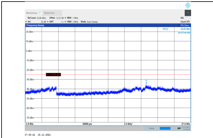
Band41-15MHz-QPSK-41165-1RB#0- Range3:3000~27000MHz
