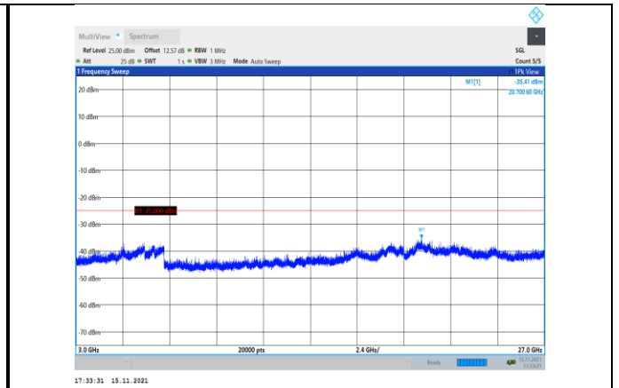
Band41-20MHz-QPSK-40590-1RB#0- Range3:3000~27000MHz
