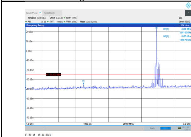
Band41-20MHz-QPSK-40590-1RB#0- Range2:1000~3000MHz
