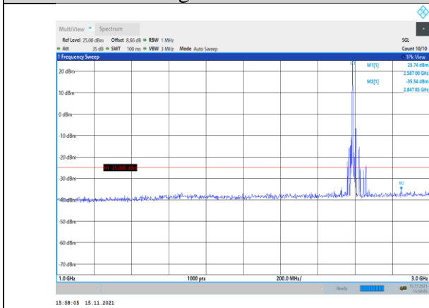
Band38-20MHz-QPSK-38000-1RB#0- Range2:1000~3000MHz
