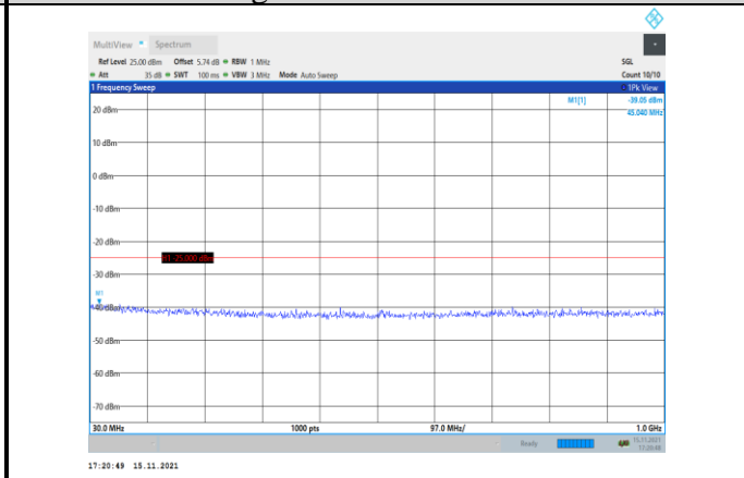
Band41-5MHz-QPSK-41215-1RB#0- Range1:30~1000MHz
