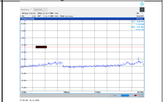
Band66-5MHz-QPSK-131997-1RB#0- Range2:1000~20000MHz
