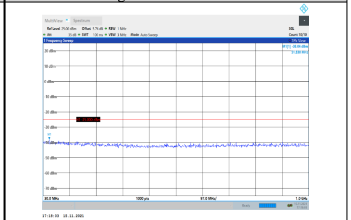
Band41-5MHz-QPSK-40065-1RB#0-Range1:30~1000MHz
