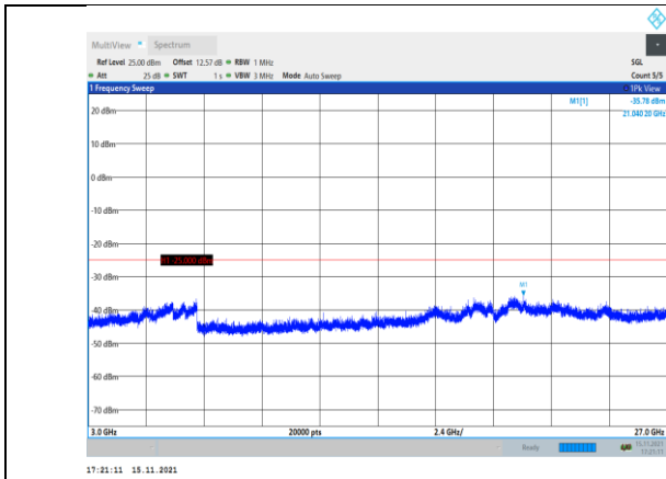
Band41-5MHz-QPSK-41215-1RB#0- Range3:3000~27000MHz
