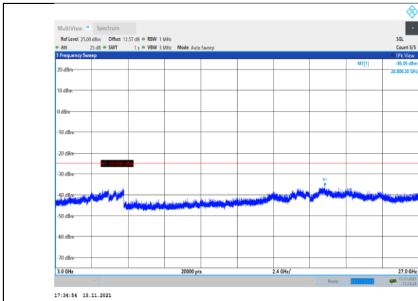
Band41-20MHz-QPSK-41140-1RB#0- Range3:3000~27000MHz
