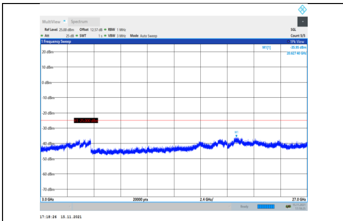
Band41-5MHz-QPSK-40065-1RB#0- Range3:3000~27000MHz
