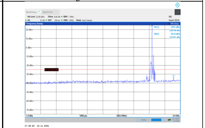
Band41-20MHz-QPSK-41140-1RB#0- Range2:1000~3000MHz
