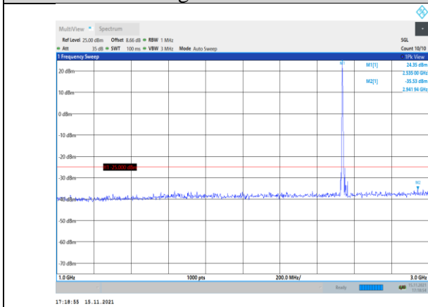
Band41-5MHz-16QAM-40065-1RB#0- Range2:1000~3000MHz
