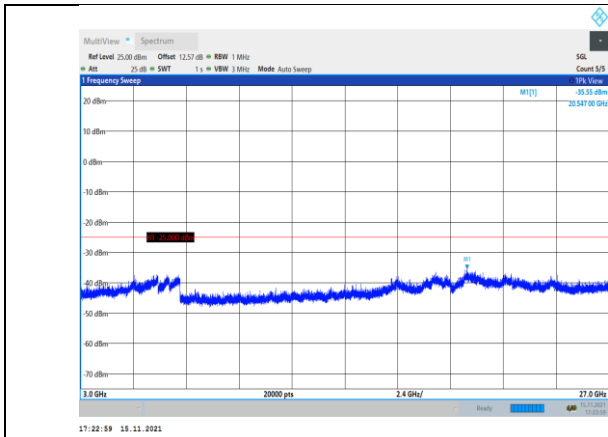
Band41-10MHz-QPSK-40090-1RB#0- Range3:3000~27000MHz
