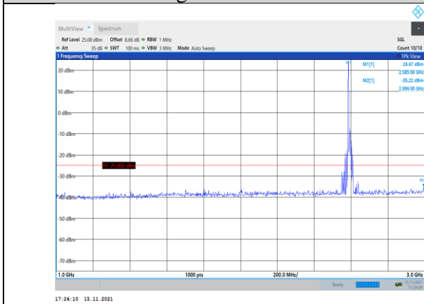
Band41-10MHz-QPSK-40590-1RB#0- Range2:1000~3000MHz
