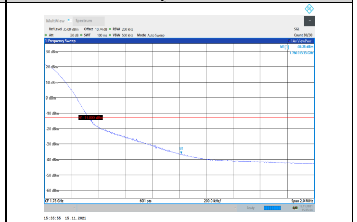
Band66-20MHz-QPSK-132572-1RB#99
