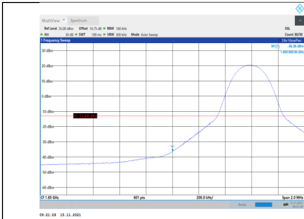
Band2-10MHz-QPSK-18650-1RB#0
