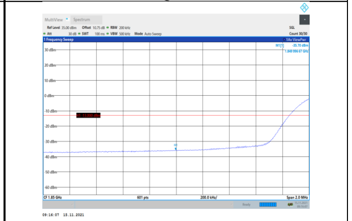
Band2-20MHz-QPSK-18700-100RB#0
