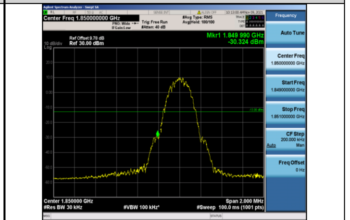
EGPRS1900-512-2
