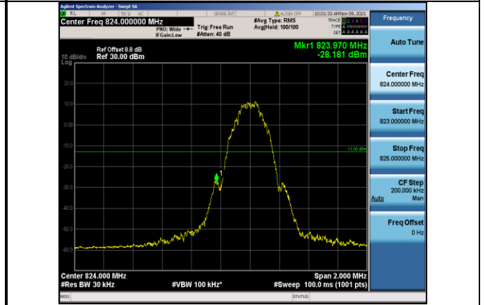
EGPRS850-128-8
