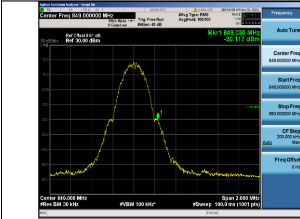
GSM850-251-3
