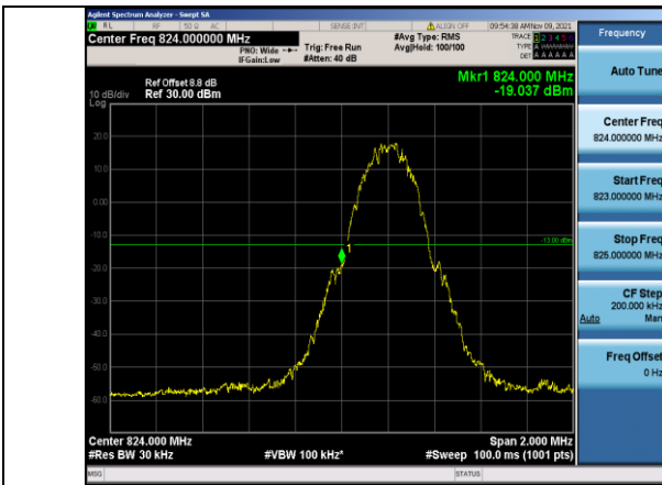
GSM850-128-3
