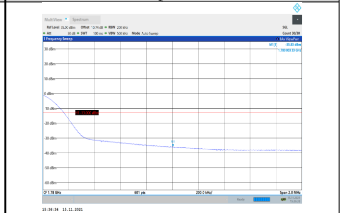
Band66-20MHz-QPSK-132572-100RB#0
