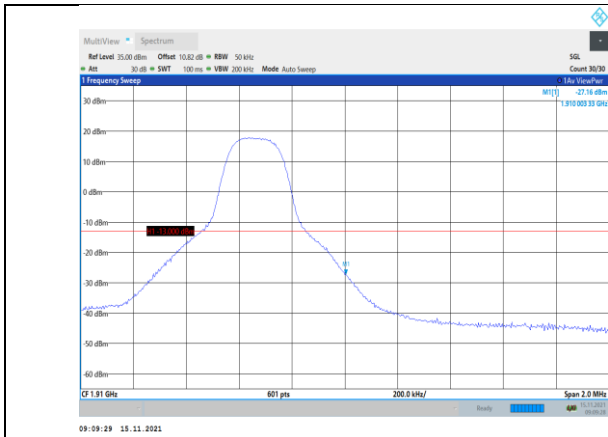
Band2-5MHz-QPSK-19175-1RB#24
