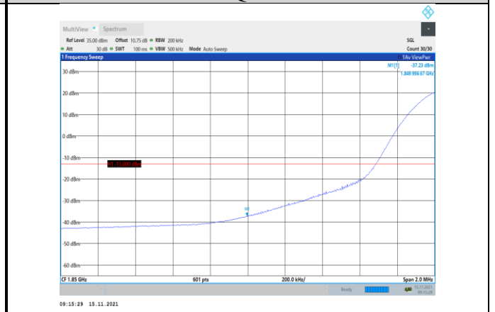
Band2-20MHz-QPSK-18700-1RB#0
