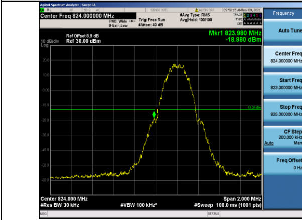
GPRS850-128-3
