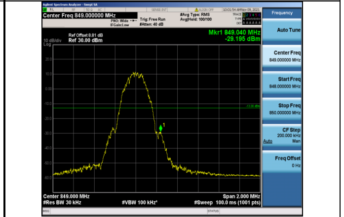
EGPRS850-251-8
