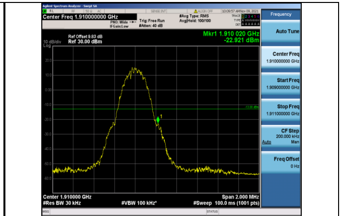
GPRS1900-810-0
