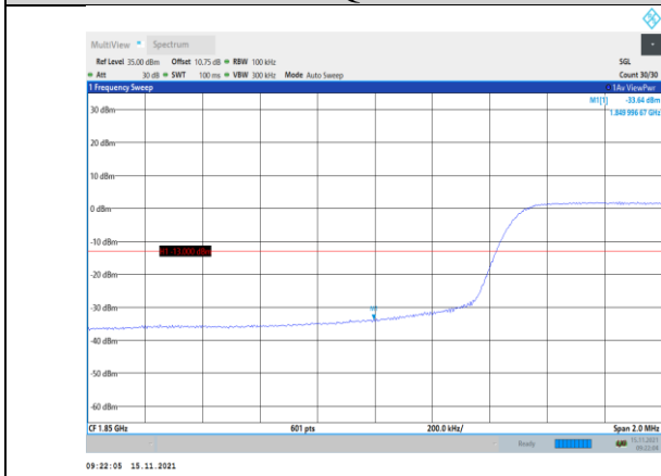
Band2-10MHz-QPSK-18650-50RB#0
