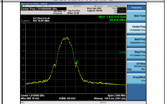
EGPRS1900-810-2
