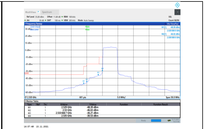
Band41-5MHz-QPSK-40065-25RB#0
