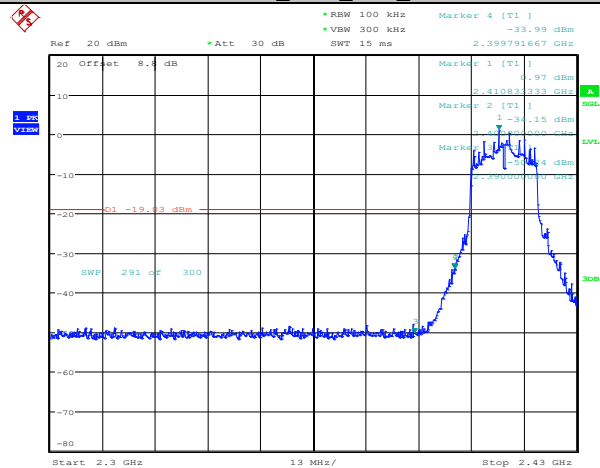
11G_Ant1_Low_2412
