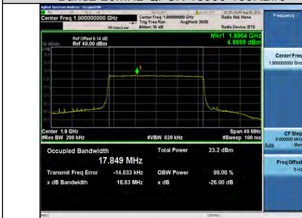
Band2-20MHz-QPSK-19100-100RB#0
