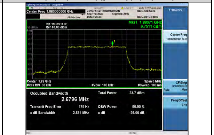
Band2-3MHz-16QAM-18800-15RB#0
