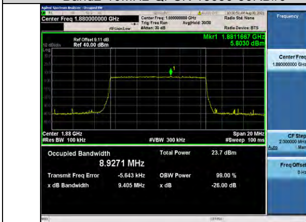
Band2-10MHz-QPSK-18800-50RB#0
