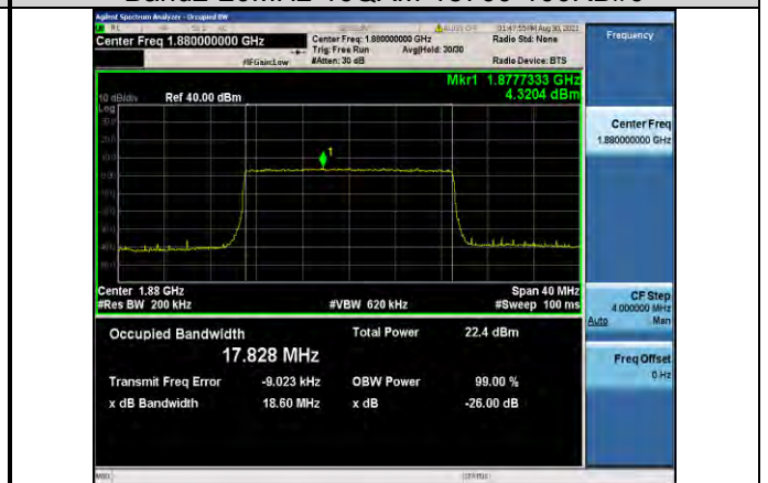
Band2-20MHz-16QAM-18900-100RB#0
