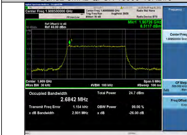
Band2-3MHz-QPSK-19185-15RB#0
