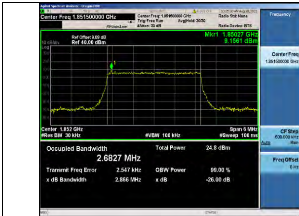
Band2-3MHz-QPSK-18615-15RB#0
