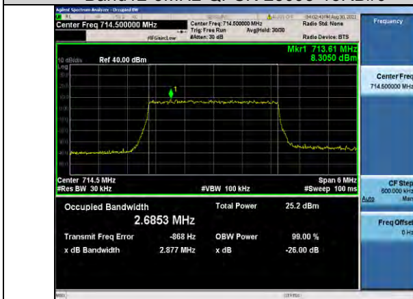
Band12-3MHz-QPSK-23165-15RB#0
