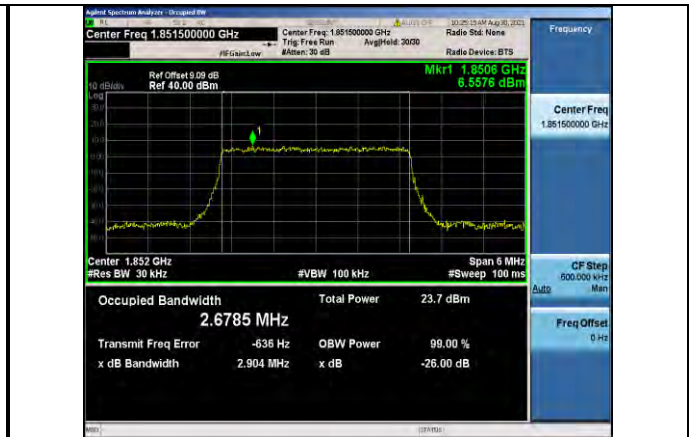
Band2-3MHz-16QAM-18615-15RB#0
