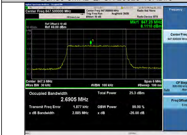
Band5-3MHz-QPSK-20635-15RB#0
