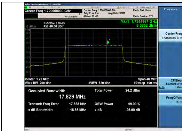
Band4-20MHz-QPSK-20050-100RB#0
