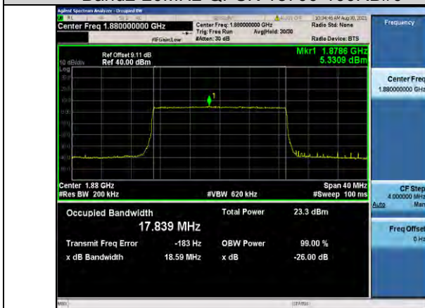
Band2-20MHz-QPSK-18900-100RB#0
