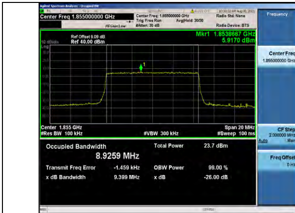
Band2-10MHz-QPSK-18650-50RB#0
