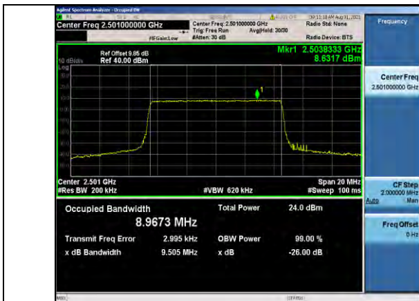
Band41-10MHz-QPSK-39700-50RB#0
