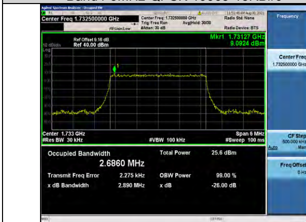
Band4-3MHz-QPSK-17325-15RB#0
