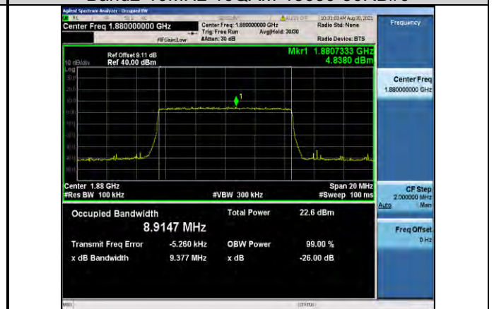
Band2-10MHz-16QAM-18800-50RB#0
