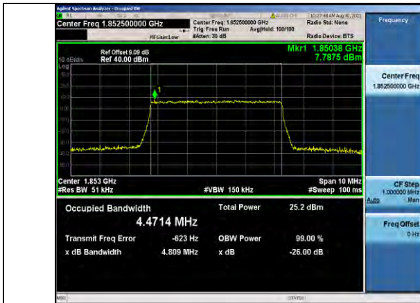
Band2-5MHz-QPSK-18625-25RB#0
