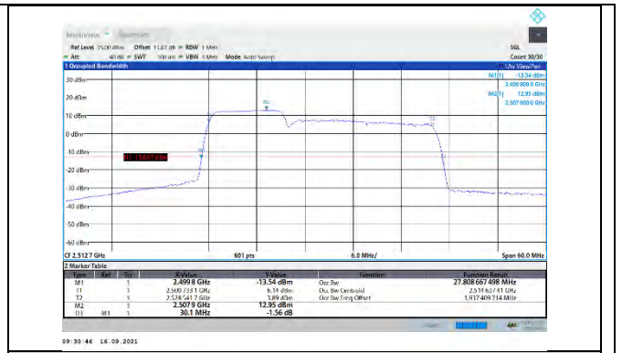
CA_7C-10MHz-20MHz-QPSK-QPSK-20805-20949-50RB#0-100RB#0
