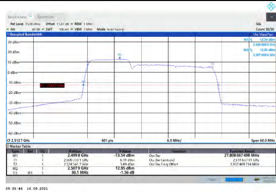
CA_7C-10MHz-20MHz-QPSK-QPSK-20805-20949-50RB#0-100RB#0
