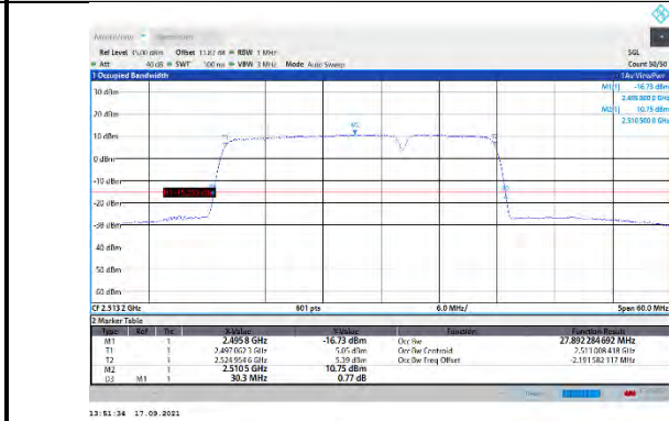
CA_41C-20MHz-10MHz-QPSK-QPSK-39750-39894-100RB#0-50RB#0
