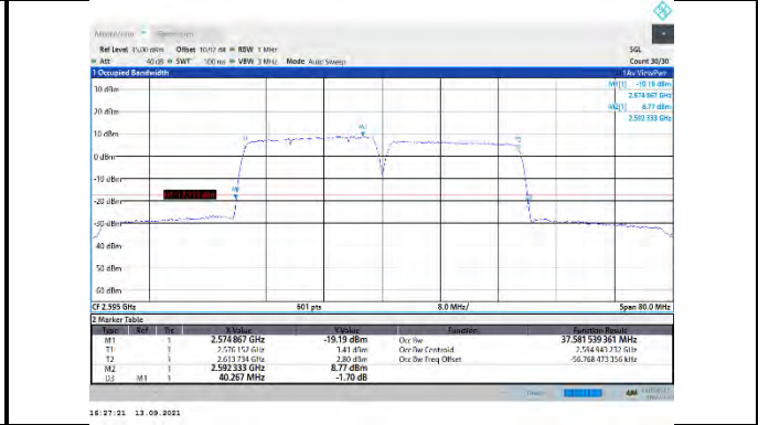
CA_38C-20MHz-20MHz-QPSK-QPSK-37901-38099-100RB#0-100RB#0
