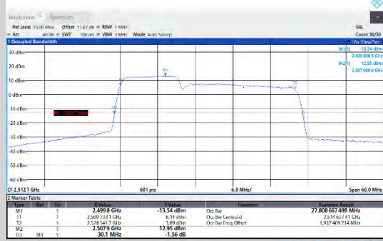
CA_7C-10MHz-20MHz-QPSK-QPSK-20805-20949-50RB#0-100RB#0
