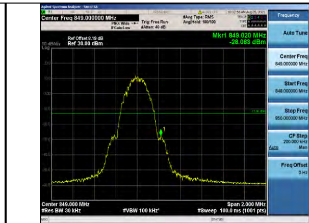
EGPRS850-251
