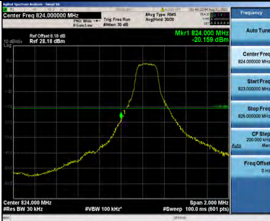
Band5-3MHz-QPSK-20415-1RB#0
