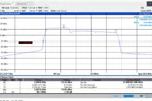
CA_7C-10MHz-20MHz-QPSK-QPSK-20805-20949-50RB#0-100RB#0
