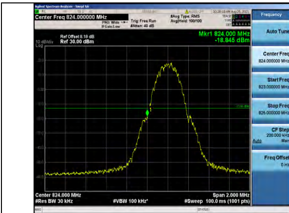
GSM850-128
