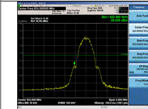
EGPRS850-128
