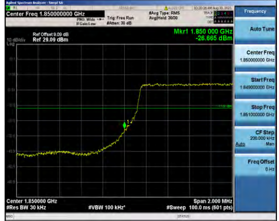
Band2-3MHz-QPSK-19185-1RB#14
