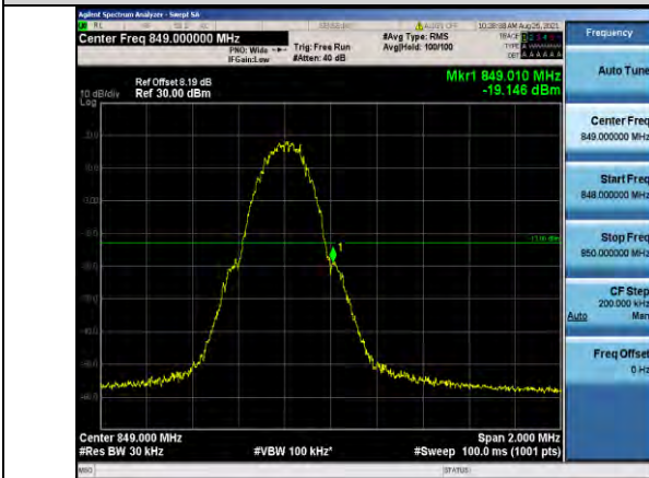
GSM850-251
