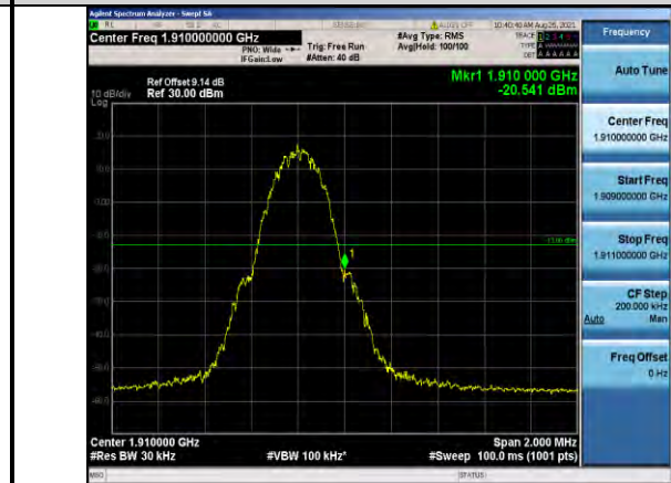
GSM1900-810
