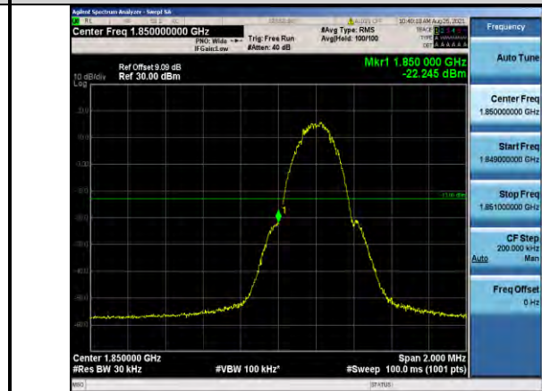
GSM1900-512
