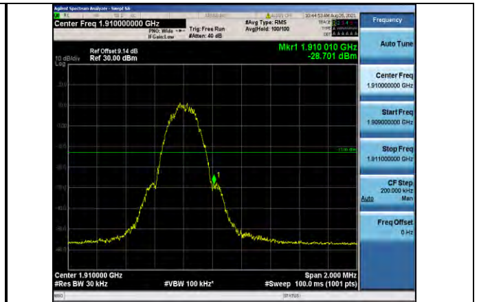
EGPRS1900-810
