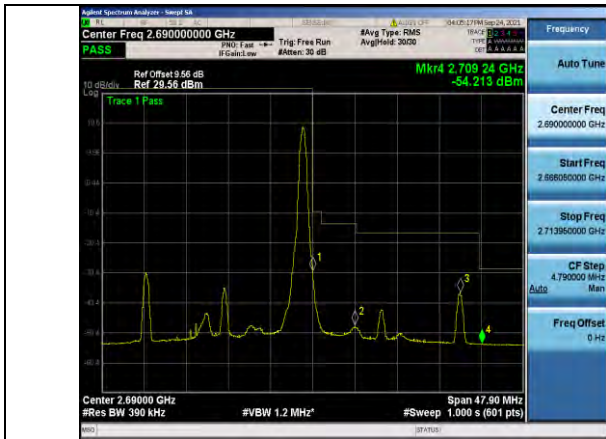
Band41-20MHz-QPSK-41490-1RB#99
