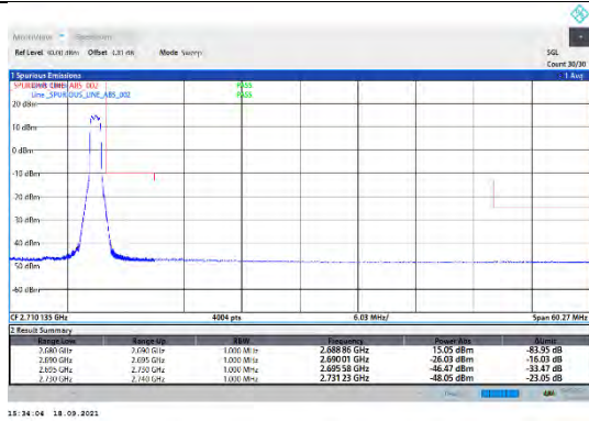
CA_41C-20MHz-20MHz-QPSK-QPSK-41292-41490-0RB#0-1RB#99
