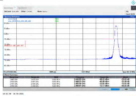
CA_41C-20MHz-20MHz-QPSK-QPSK-39750-39948-1RB#0-0RB#0
