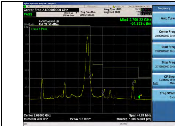
Band41-20MHz-16QAM-41490-1RB#99
