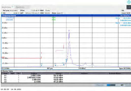
CA_7C-10MHz-20MHz-QPSK-QPSK-20805-20949-1RB#0-0RB#0
