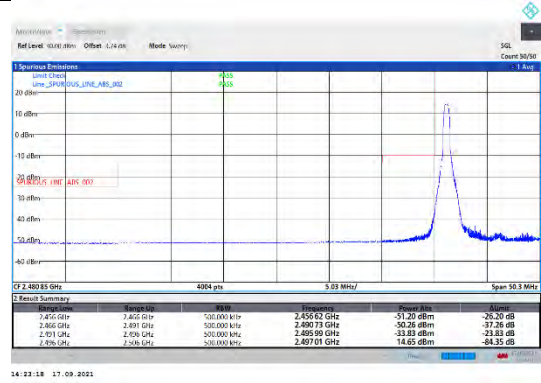
CA_41C-20MHz-10MHz-QPSK-QPSK-39750-39894-1RB#0-0RB#0
