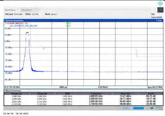
CA_41C-20MHz-20MHz-16QAM-16QAM-41292-41490-0RB#0-1RB#99
