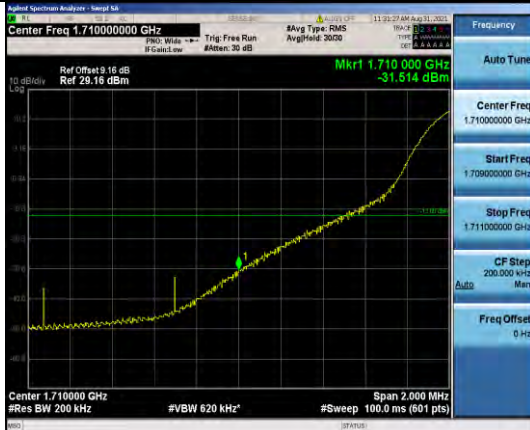
Band66-20MHz-QPSK-132072-1RB#0
