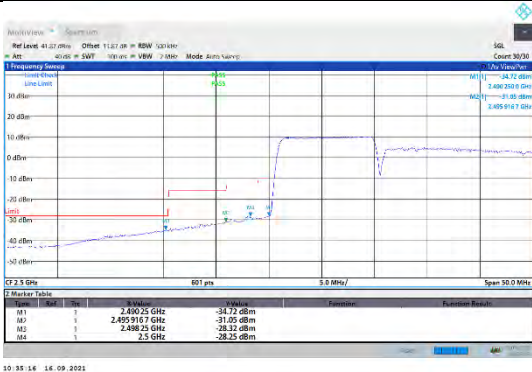
CA_7C-10MHz-20MHz-QPSK-QPSK-20805-20949-50RB#0-100RB#0
