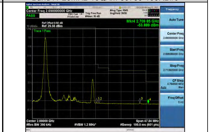
Band41-20MHz-16QAM-41490-1RB#0
