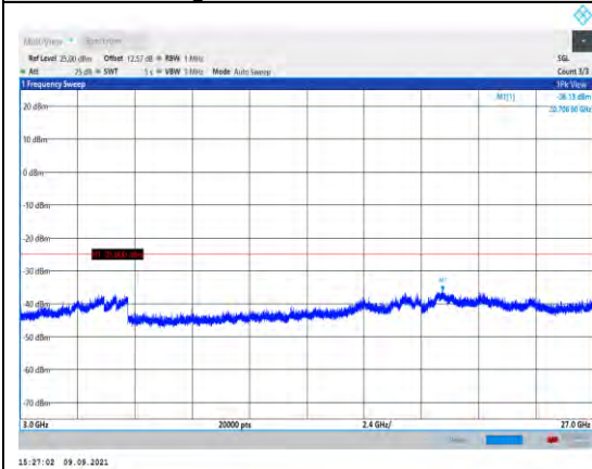
Band7-10MHz-QPSK-21400-1RB#0- Range3:3000~27000MHz
