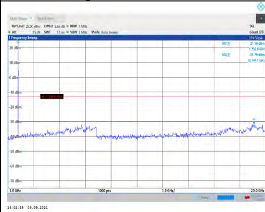
Band4-20MHz-QPSK-20300-1RB#0- Range2:1000~20000MHz
