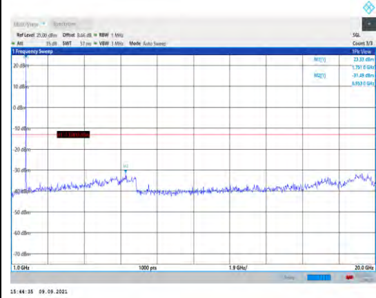
Band4-1.4MHz-QPSK-20393-1RB#0- Range2:1000~20000MHz
