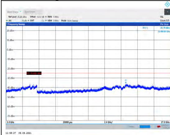
Band41-5MHz-QPSK-41565-1RB#0- Range3:3000~27000MHz
