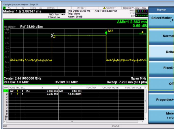
GFSK DH5
