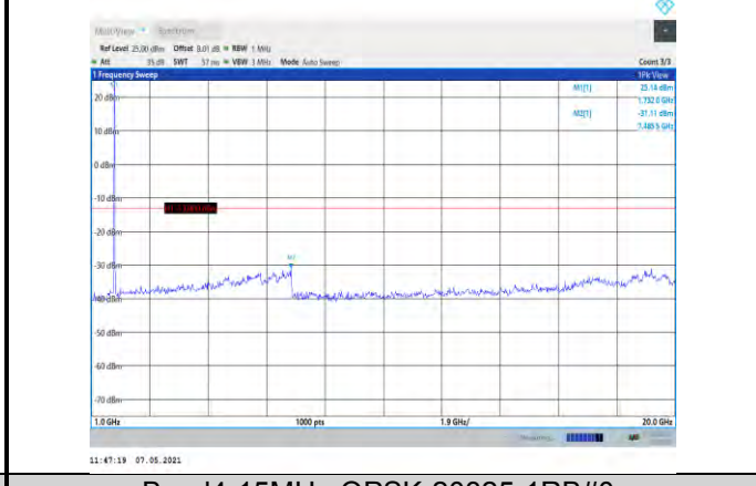
Band4-15MHz-QPSK-20325-1RB#0- Range2:1000~20000MHz
