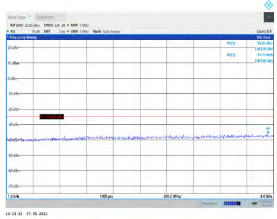
Band7-10MHz-QPSK-21100-1RB#0- Range2:1000~3000MHz
