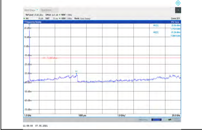
Band4-20MHz-QPSK-20050-1RB#0- Range2:1000~20000MHz
