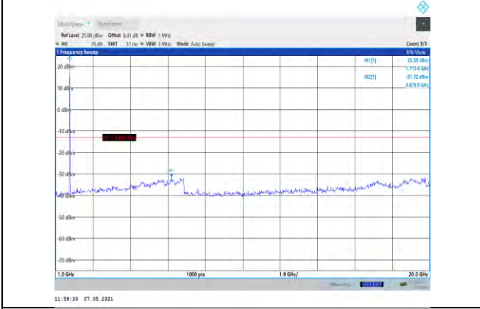
Band4-10MHz-QPSK-20000-1RB#0- Range2:1000~20000MHz
