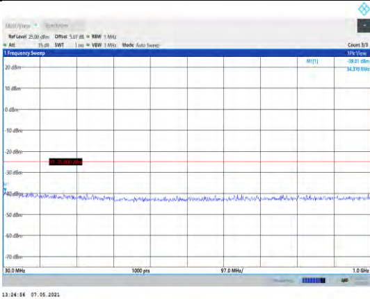
Band7-20MHz-QPSK-20850-1RB#0- Range1:30~1000MHz
