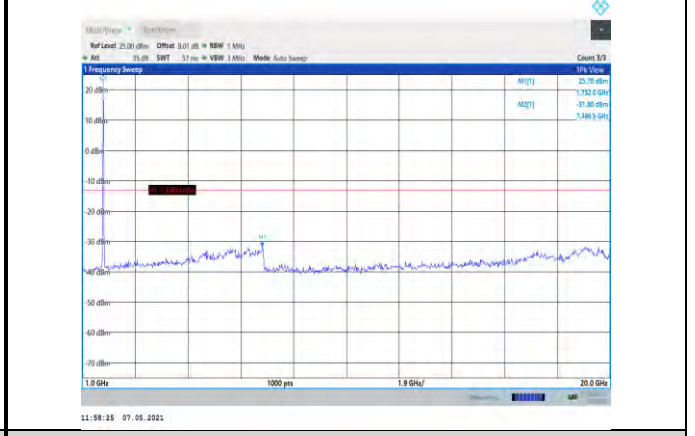
Band4-20MHz-QPSK-20300-1RB#0- Range2:1000~20000MHz
