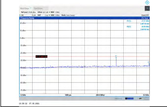
Band7-15MHz-QPSK-20825-1RB#0- Range2:1000~3000MHz
