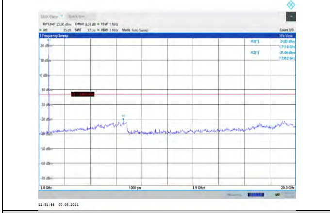
Band4-5MHz-QPSK-19975-1RB#0-Range2:1000~20000MHz
