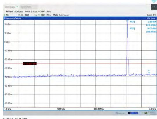
Band38-5MHz-QPSK-38225-1RB#0- Range2:1000~3000MHz
