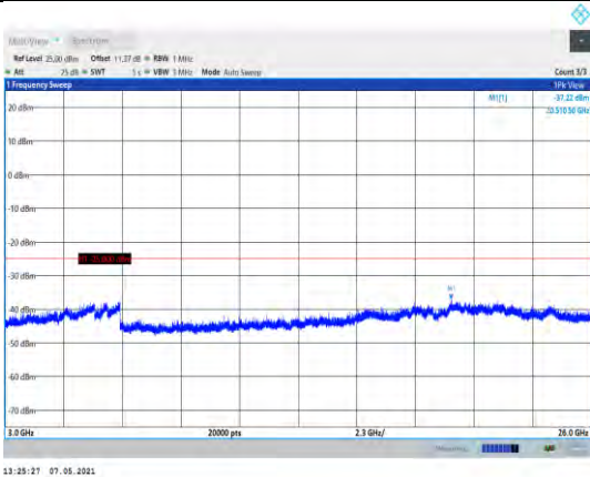
Band7-20MHz-QPSK-20850-1RB#0- Range3:3000~26000MHz
