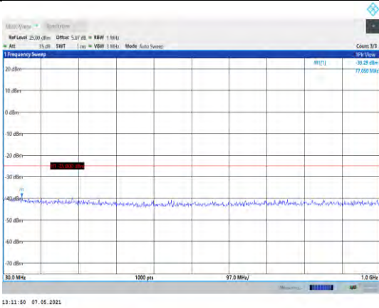
Band7-10MHz-QPSK-20800-1RB#0- Range1:30~1000MHz
