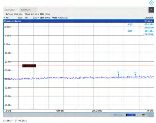
Band7-20MHz-QPSK-21100-1RB#0- Range2:1000~3000MHz
