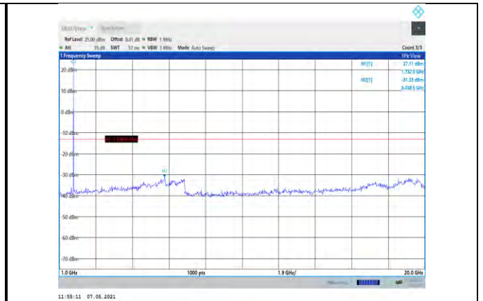
Band4-3MHz-QPSK-20175-1RB#0- Range2:1000~20000MHz
