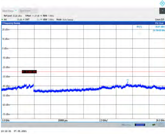
Band7-10MHz-QPSK-20800-1RB#0- Range3:3000~26000MHz
