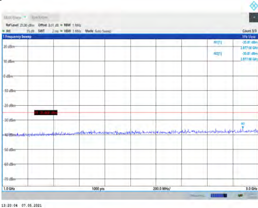
Band7-5MHz-QPSK-20775-1RB#0-Range2:1000~3000MHz
