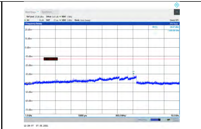
Band5-10MHz-QPSK-20525-1RB#0- Range2:1000~10000MHz
