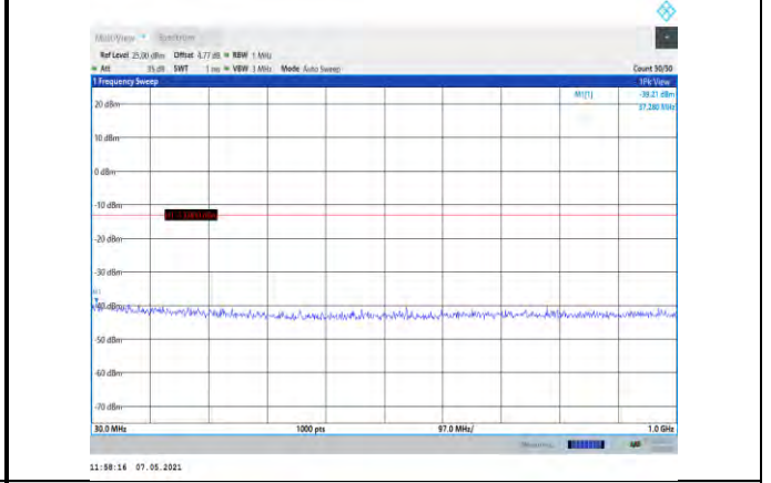
Band4-20MHz-QPSK-20300-1RB#0- Range1:30~1000MHz
