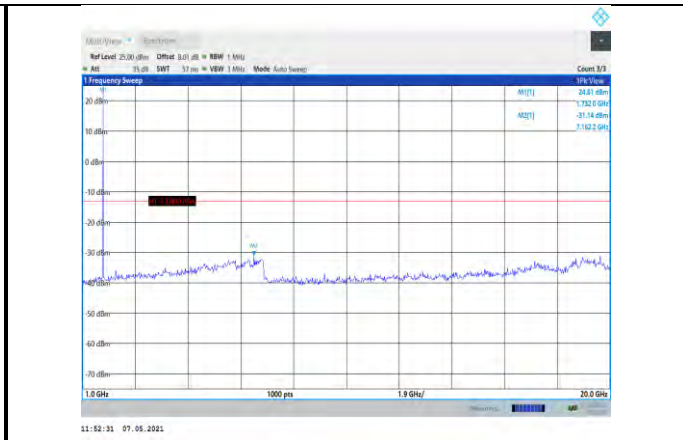
Band4-5MHz-QPSK-20175-1RB#0-Range2:1000~20000MHz
