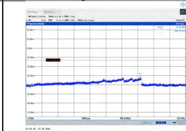
Band12-5MHz-QPSK-23155-1RB#0- Range2:1000~10000MHz
