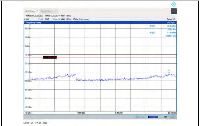
Band4-10MHz-QPSK-20175-1RB#0- Range2:1000~20000MHz
