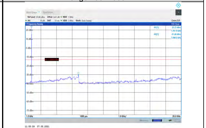
Band4-3MHz-QPSK-20385-1RB#0- Range2:1000~20000MHz
