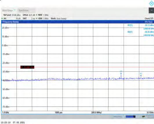
Band7-5MHz-QPSK-21425-1RB#0-Range2:1000~3000MHz
