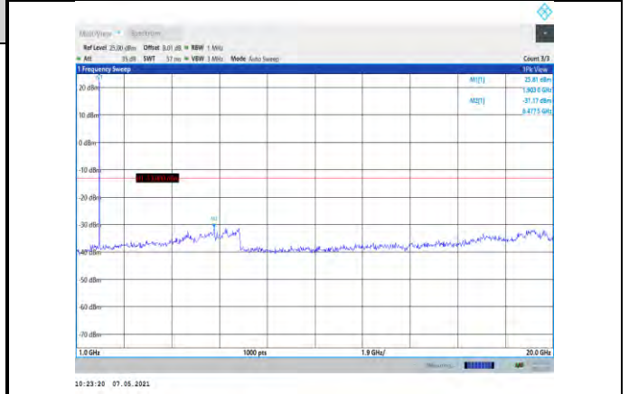
Band2-1.4MHz-QPSK-19193-1RB#0- Range2:1000~20000MHz
