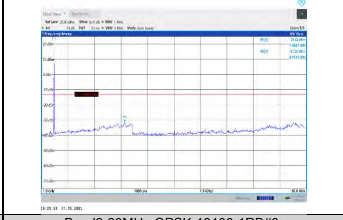
Band2-20MHz-QPSK-19100-1RB#0- Range2:1000~20000MHz
