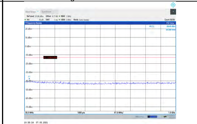
Band2-5MHz-QPSK-19175-1RB#0- Range1:30~1000MHz
