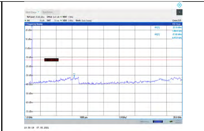
Band2-10MHz-QPSK-18900-1RB#0-Range2:1000~20000MHz
