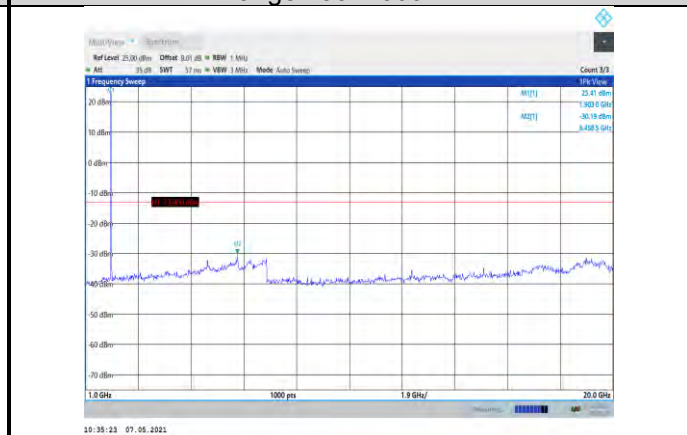
Band2-5MHz-QPSK-19175-1RB#0- Range2:1000~20000MHz
