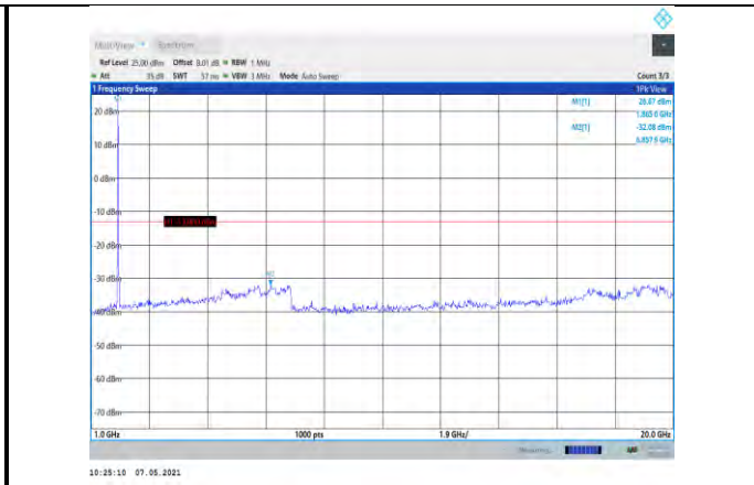
Band2-20MHz-16QAM-18900-1RB#0- Range2:1000~20000MHz
