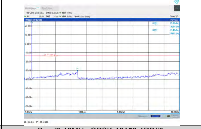
Band2-10MHz-QPSK-19150-1RB#0-Range2:1000~20000MHz
