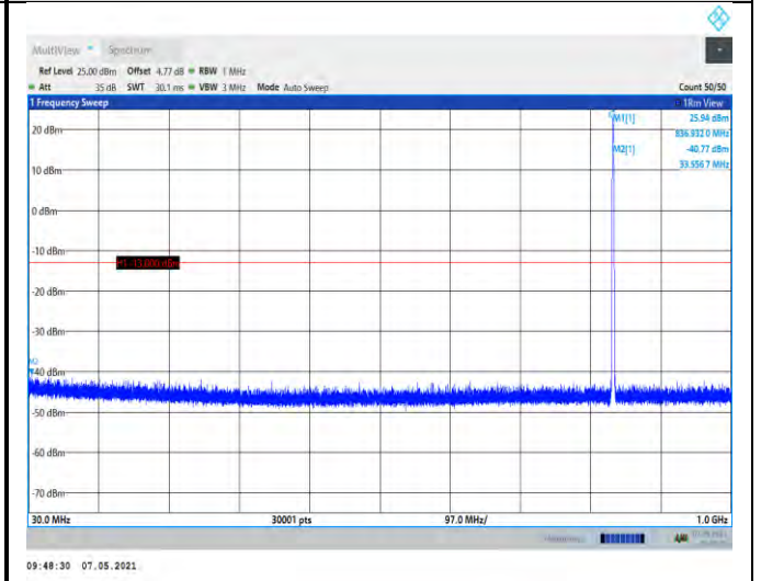
EGPRS850-190-30~1000MHz
