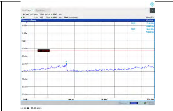
Band2-3MHz-QPSK-18900-1RB#0-Range2:1000~20000MHz
