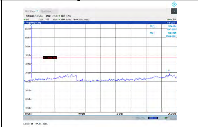
Band2-3MHz-QPSK-19185-1RB#0-Range2:1000~20000MHz
