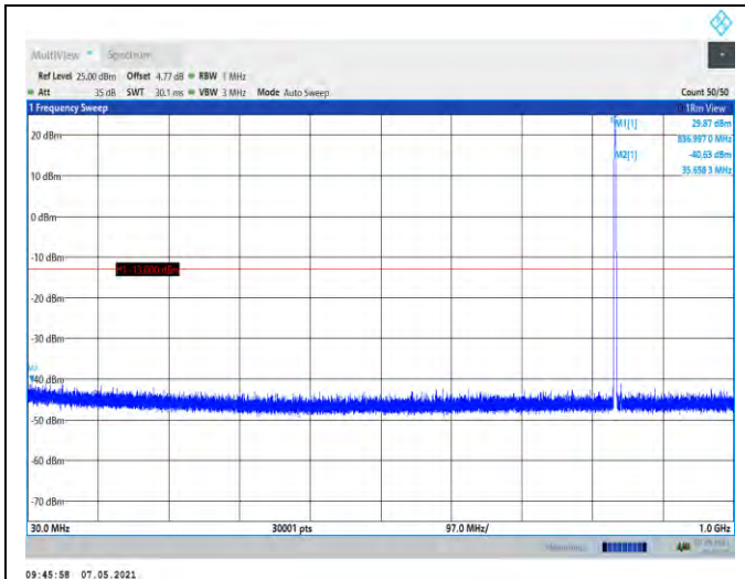
GSM850-128-30~1000MHz
