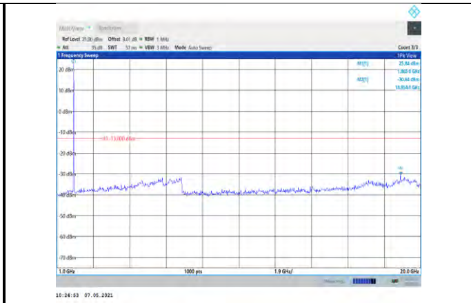
Band2-20MHz-QPSK-18900-1RB#0- Range2:1000~20000MHz
