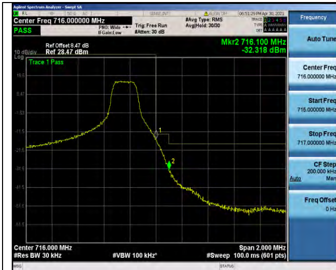
Band12-3MHz-QPSK-23165-1RB#14
