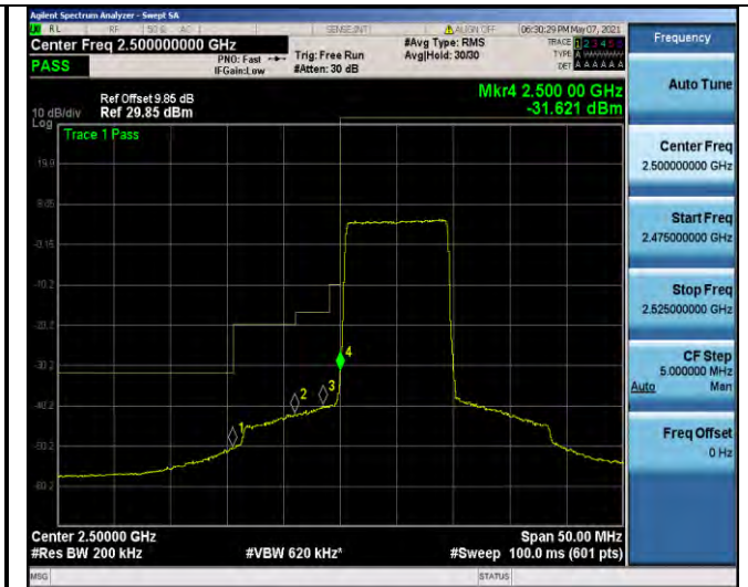
Band7-10MHz-QPSK-20800-50RB#0
