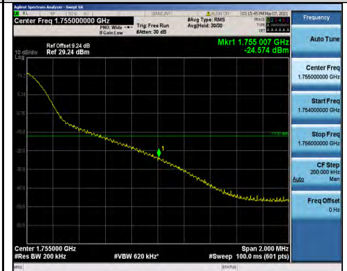
Band4-20MHz-QPSK-20300-1RB#99
