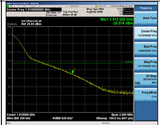
Band2-20MHz-QPSK-19100-1RB#99
