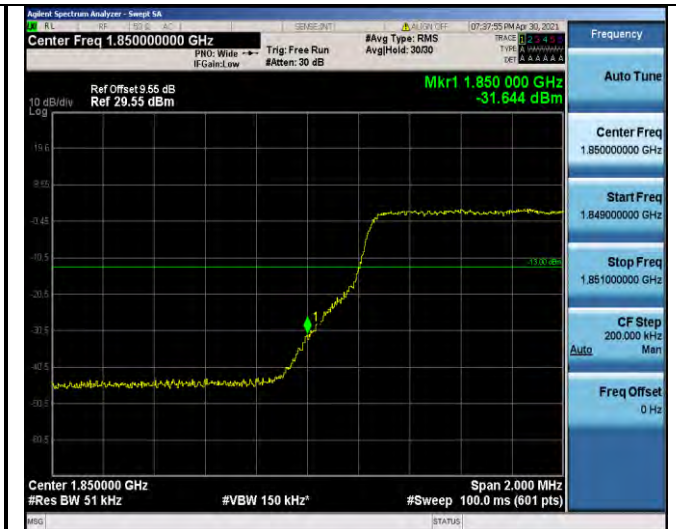
Band2-5MHz-QPSK-18625-25RB#0
