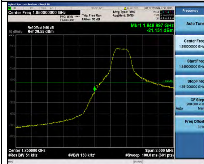
Band2-5MHz-QPSK-18625-1RB#0
