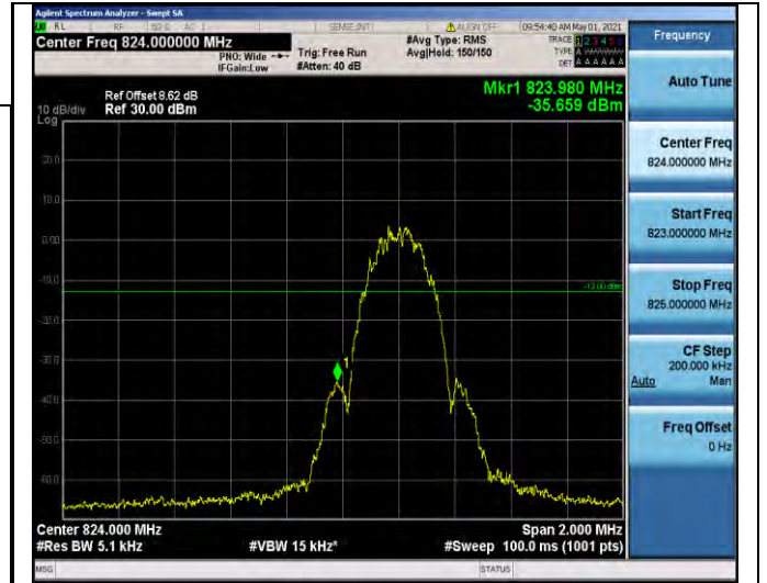
EGPRS850-128
