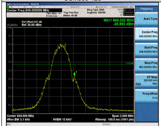
GSM850-251
