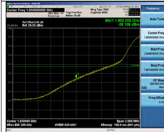
Band2-20MHz-QPSK-18700-1RB#0
