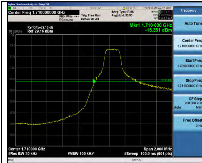
Band4-3MHz-QPSK-19965-1RB#0
