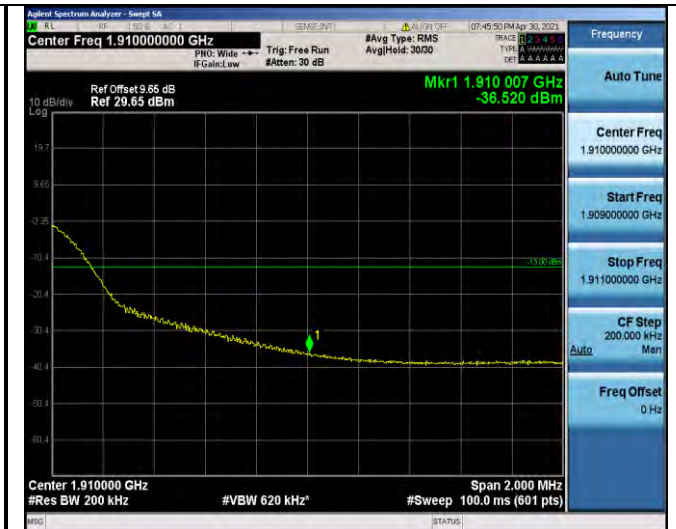
Band2-20MHz-16QAM-19100-100RB#0
