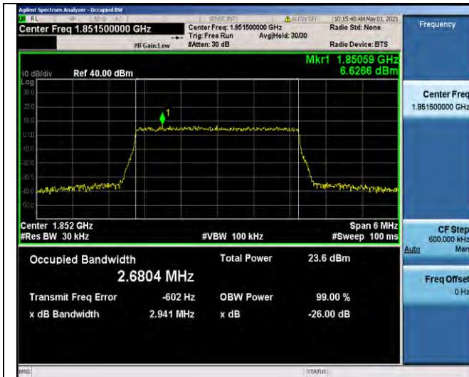
Band2-3MHz-16QAM-18615-15RB#0-2.6804
