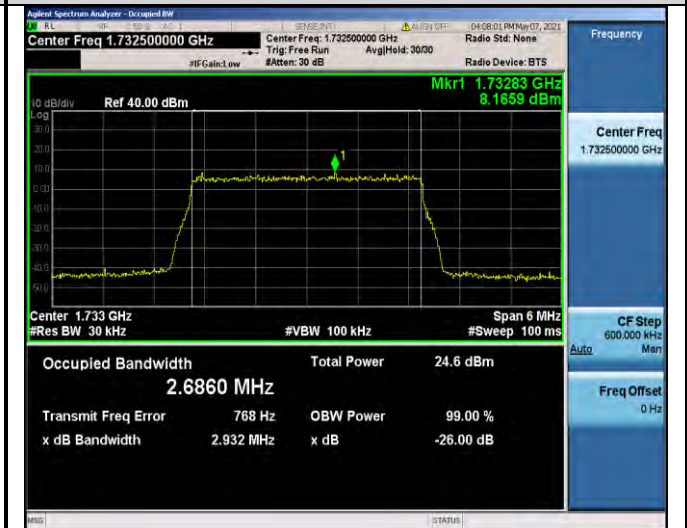
Band4-3MHz-QPSK-20175-15RB#0-2.6860
