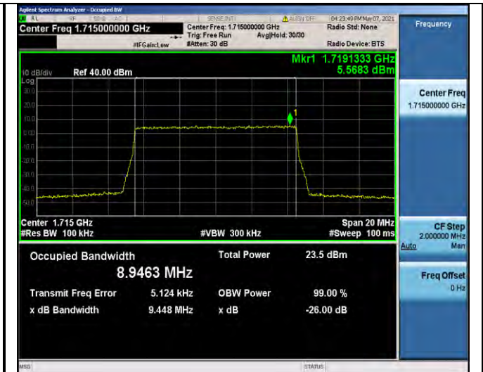
Band4-10MHz-QPSK-20000-50RB#0-8.9463
