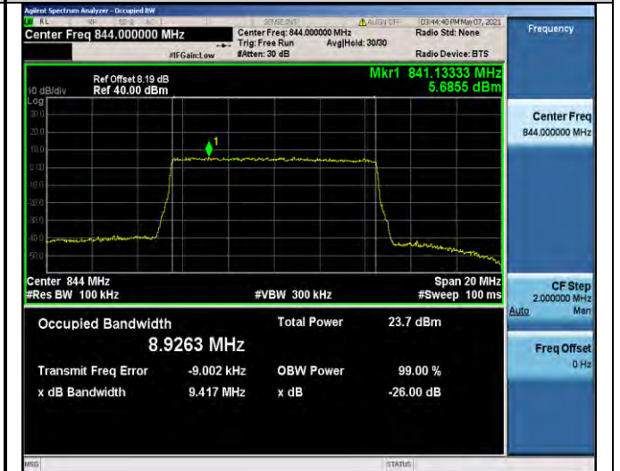
Band5-10MHz-QPSK-20600-50RB#0-8.9263
