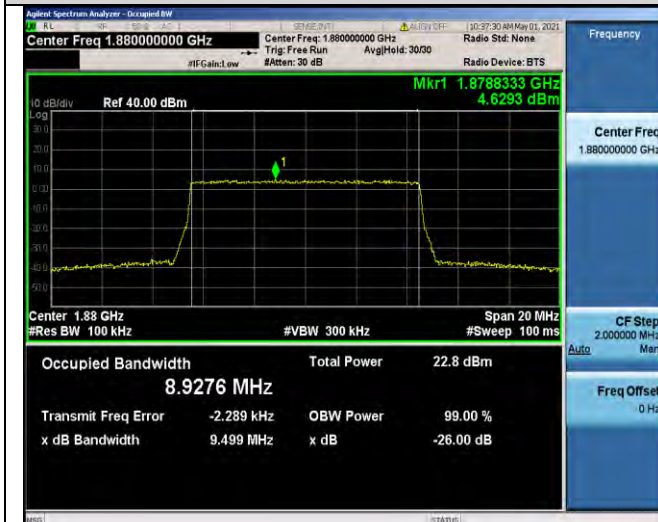
Band2-10MHz-16QAM-18900-50RB#0-8.9276
