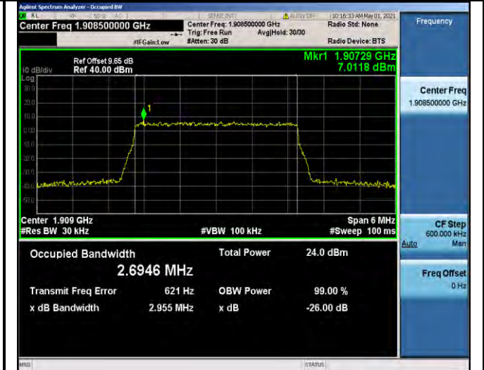
Band2-3MHz-QPSK-19185-15RB#0-2.6946
