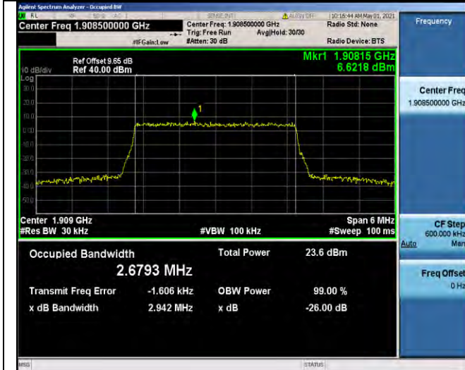
Band2-3MHz-16QAM-19185-15RB#0-2.6793
