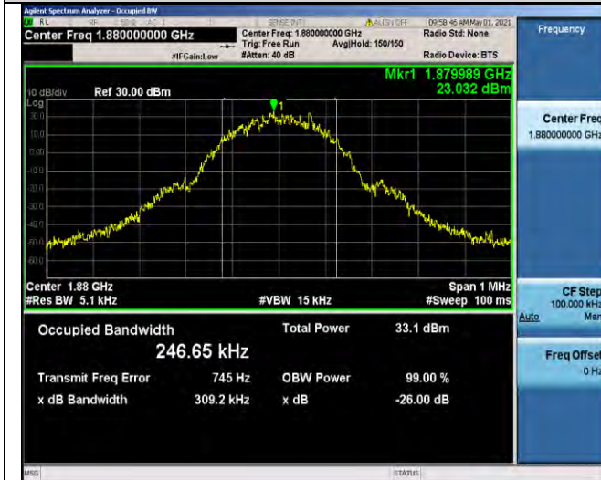
GSM1900-661
