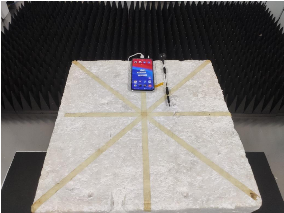
Close-up-BT/WIFI
