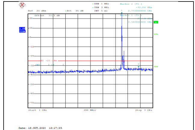
Band7-20MHz-QPSK-20850-1RB#0-Range2:1000~3000MHz--32.06-PASS
