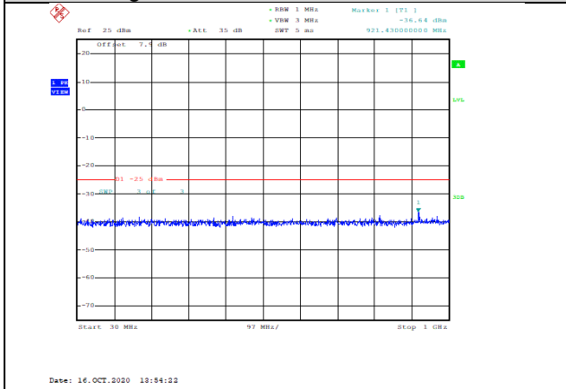
Band41-5MHz-QPSK-40065-1RB#0-Range1:30~1000MHz--36.64-PASS
