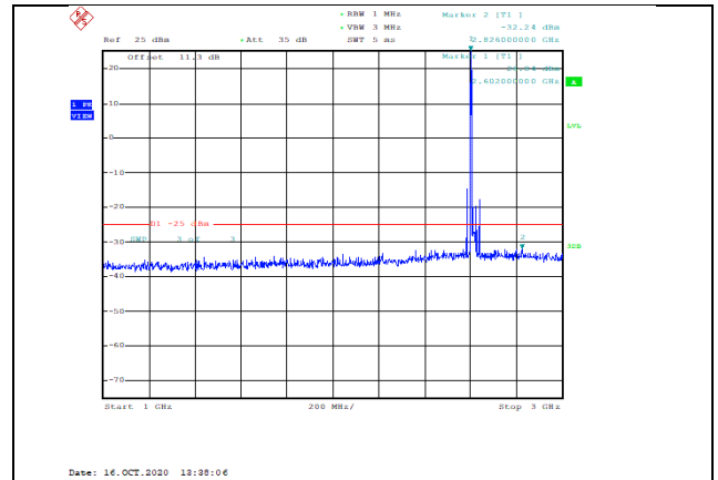
Band38-20MHz-QPSK-38150-1RB#0-Range2:1000~3000MHz--32.24-PASS
