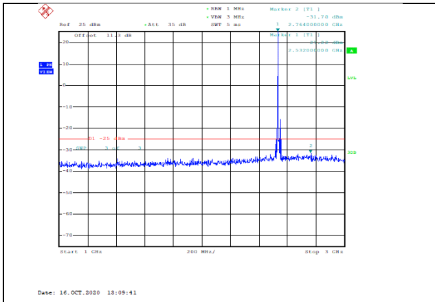
Band7-10MHz-QPSK-21100-1RB#0-Range2:1000~3000MHz--31.7-PASS
