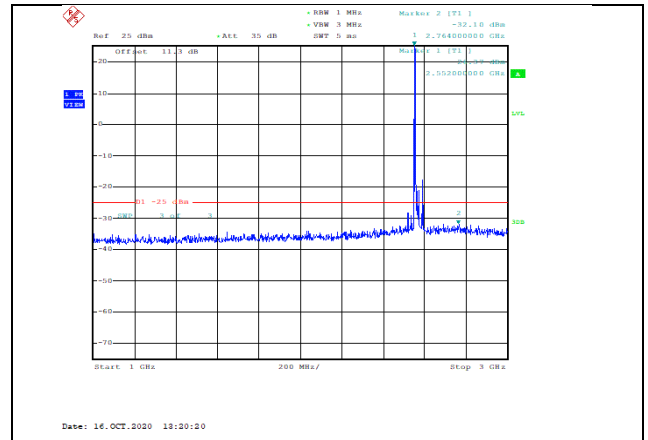
Band7-20MHz-QPSK-21350-1RB#0-Range2:1000~3000MHz--32.1-PASS
