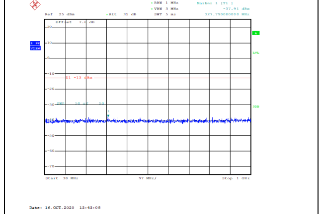
Band66-3MHz-QPSK-132322-1RB#0-Range1:30~1000MHz--37.91-PASS
