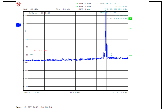
Band38-20MHz-QPSK-37850-1RB#0-Range2:1000~3000MHz--32.32-PASS
