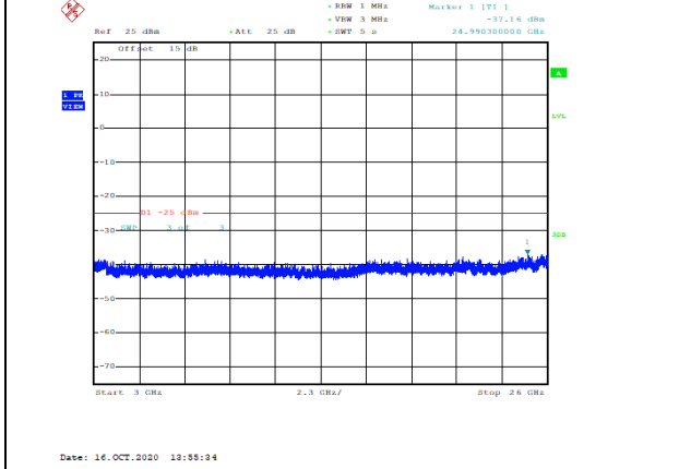
Band41-5MHz-16QAM-40065-1RB#0-Range3:3000~26000MHz--37.16-PASS
