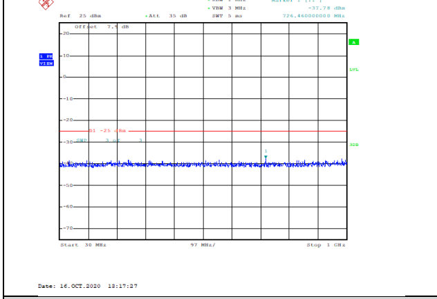
Band7-20MHz-QPSK-20850-1RB#0-Range1:30~1000MHz--37.78-PASS
