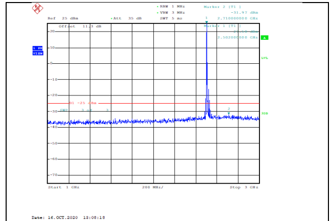
Band7-10MHz-QPSK-20800-1RB#0-Range2:1000~3000MHz--31.97-PASS
