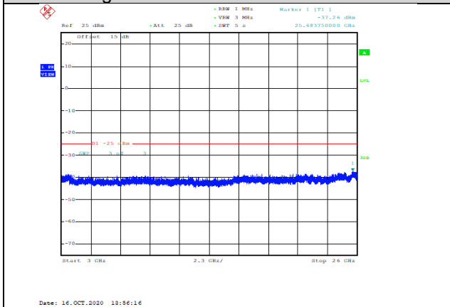
Band41-5MHz-QPSK-40590-1RB#0-Range3:3000~26000MHz--37.26-PASS
