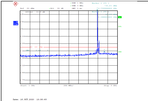
Band38-20MHz-QPSK-38000-1RB#0-Range2:1000~3000MHz--32.01-PASS
