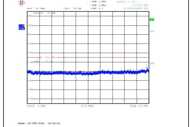
Band7-10MHz-QPSK-20800-1RB#0-Range3:3000~26000MHz--37-PASS
