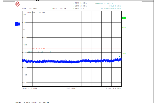
Band38-20MHz-QPSK-37850-1RB#0-Range3:3000~26000MHz--36.24-PASS
