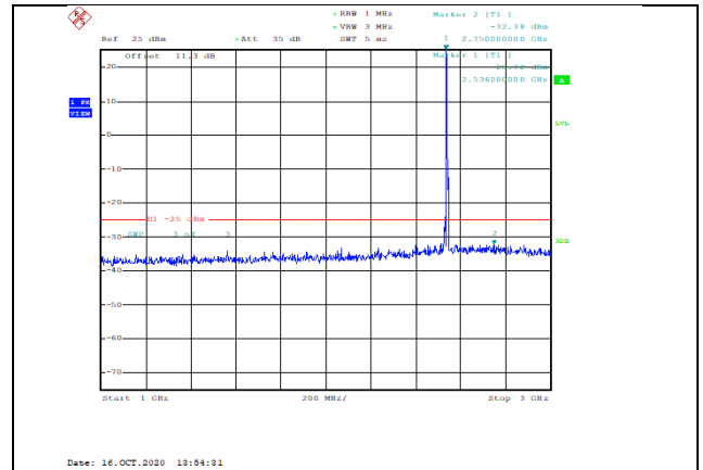
Band41-5MHz-QPSK-40065-1RB#0-Range2:1000~3000MHz--32.38-PASS
