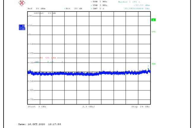
Band7-20MHz-QPSK-20850-1RB#0-Range3:3000~26000MHz--37.37-PASS
