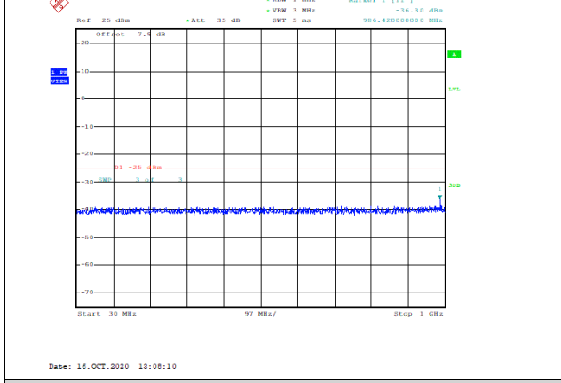
Band7-10MHz-QPSK-20800-1RB#0-Range1:30~1000MHz--36.3-PASS
