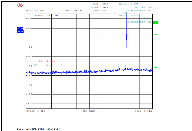
Band41-5MHz-QPSK-40590-1RB#0-Range2:1000~3000MHz--31.89-PASS
