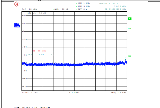
Band41-10MHz-QPSK-40590-1RB#0-Range3:3000~26000MHz--36.76-PASS
