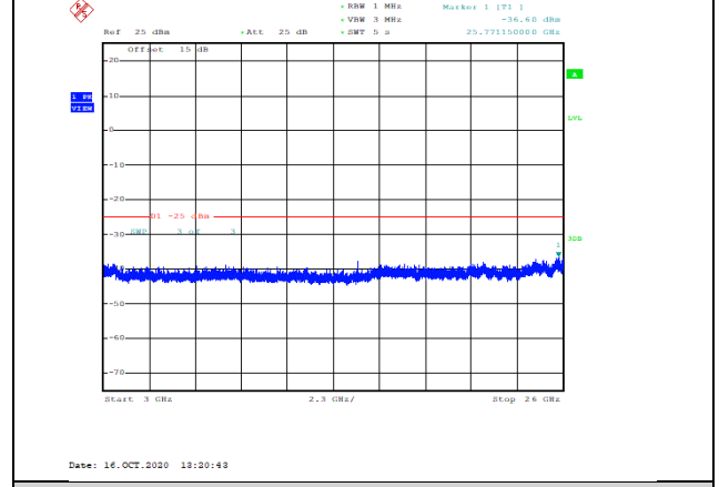
Band7-20MHz-QPSK-21350-1RB#0-Range3:3000~26000MHz--36.6-PASS
