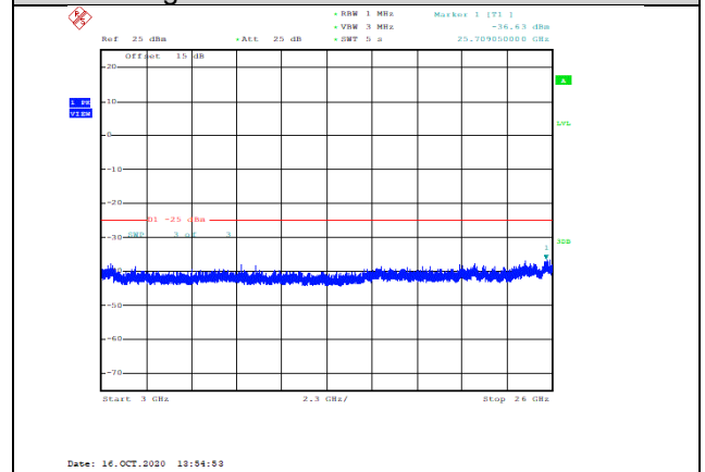
Band41-5MHz-QPSK-40065-1RB#0-Range3:3000~26000MHz--36.63-PASS
