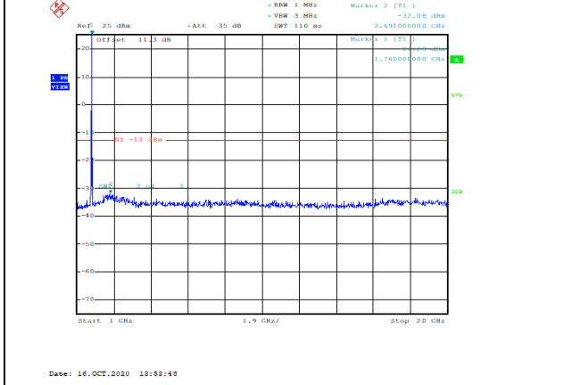
Band66-20MHz-QPSK-132572-1RB#0-Range2:1000~20000MHz--32.08-PASS
