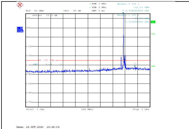
Band38-20MHz-16QAM-37850-1RB#0-Range2:1000~3000MHz--32.25-PASS
