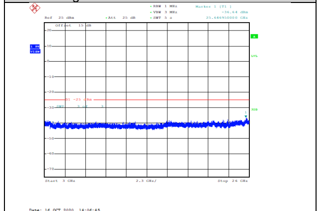
Band41-15MHz-QPSK-41165-1RB#0-Range3:3000~26000MHz--36.64-PASS
