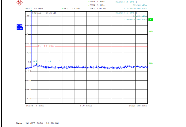
Band2-5MHz-QPSK-19175-1RB#0-Range2:1000~20000MHz--32.56-PASS
