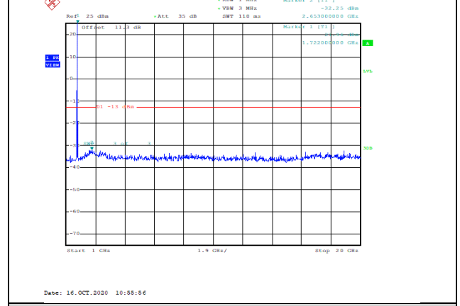
Band4-20MHz-QPSK-20175-1RB#0-Range2:1000~20000MHz--32.25-PASS
