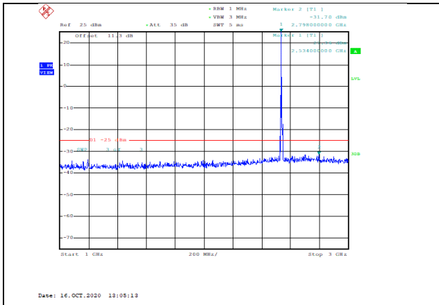
Band7-5MHz-QPSK-21100-1RB#0-Range2:1000~3000MHz--31.7-PASS
