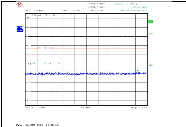
Band4-1.4MHz-QPSK-20393-1RB#0-Range1:30~1000MHz--38.36-PASS
