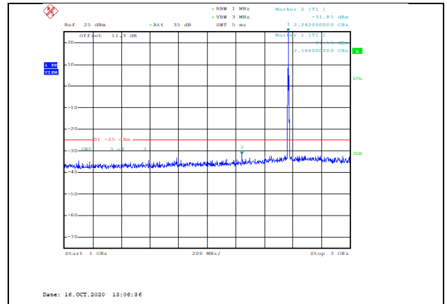
Band7-5MHz-QPSK-21425-1RB#0-Range2:1000~3000MHz--31.85-PASS
