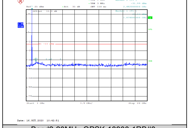
Band2-20MHz-QPSK-18900-1RB#0-Range2:1000~20000MHz--31.99-PASS
