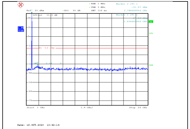
Band2-20MHz-QPSK-18700-1RB#0-Range2:1000~20000MHz--31.97-PASS
