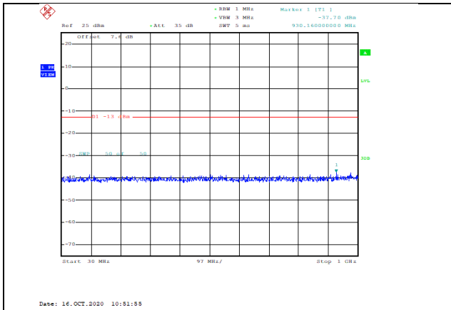
Band4-10MHz-QPSK-20350-1RB#0-Range1:30~1000MHz--37.7-PASS
