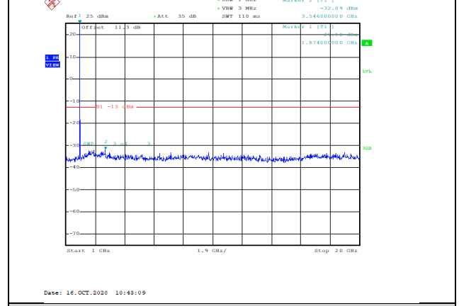
Band2-20MHz-16QAM-18900-1RB#0-Range2:1000~20000MHz--32.09-PASS
