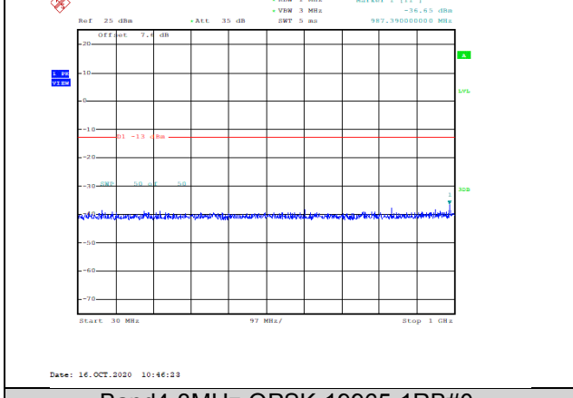
Band4-3MHz-QPSK-19965-1RB#0-Range1:30~1000MHz--36.65-PASS
