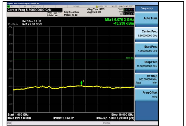
Band26-5MHz-QPSK-26765-1RB#0-Range2:1000~10000MHz
