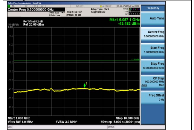
Band12-3MHz-QPSK-23165-1RB#0-Range2:1000~10000MHz
