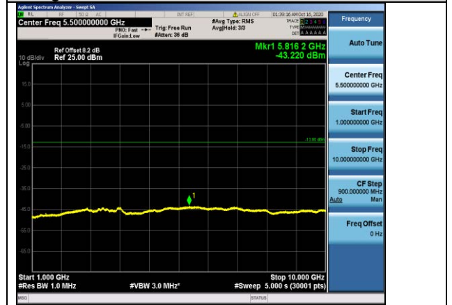
Band12-5MHz-QPSK-23155-1RB#0-Range2:1000~10000MHz
