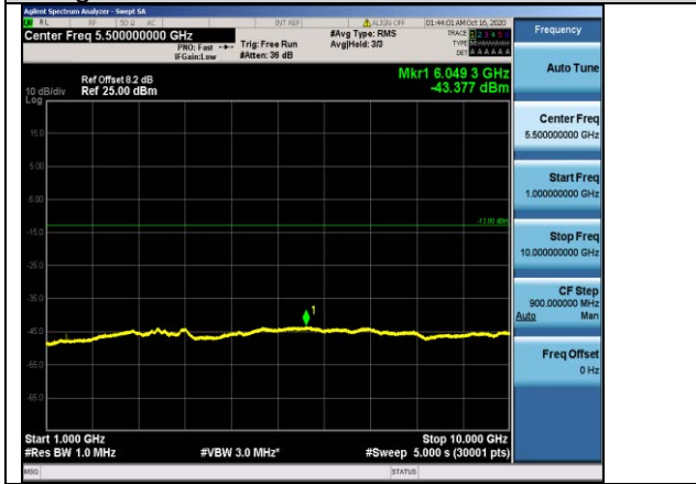
Band12-1.4MHz-QPSK-23017-1RB#0-Range2:1000~10000MHz
