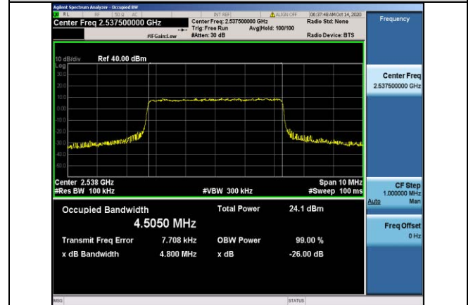
Band41-5MHz-QPSK-40065-25RB#0-4.5050
