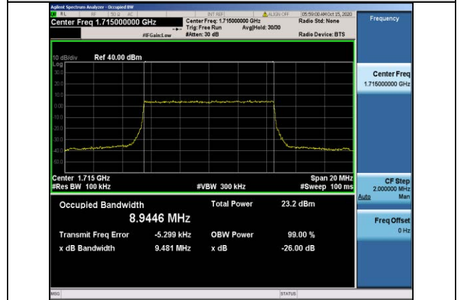
Band66-10MHz-QPSK-132022-50RB#0-8.9446
