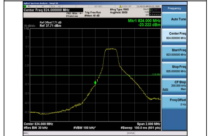
Band5-3MHz-QPSK-20415-1RB#0
