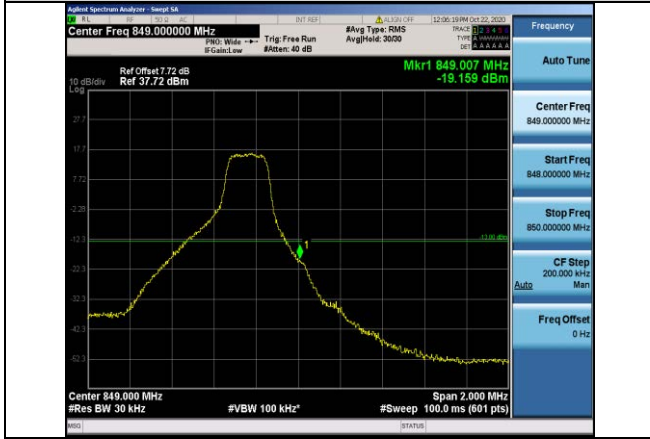
Band5-3MHz-QPSK-20635-1RB#14
