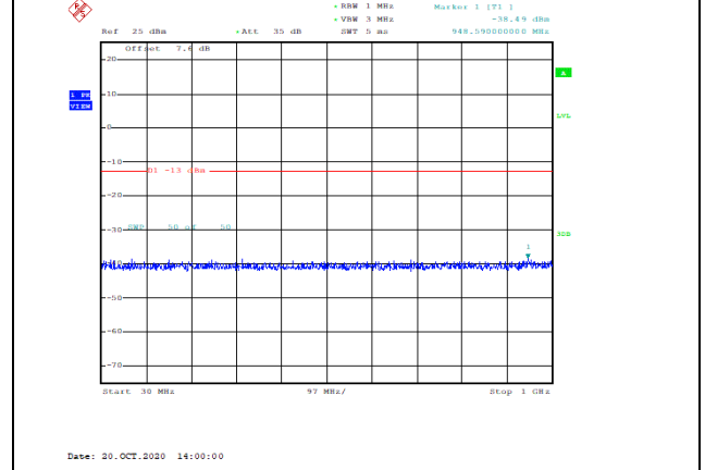
Band66-20MHz-QPSK-132072-1RB#0-Range1:30~1000MHz--38.49-PASS
