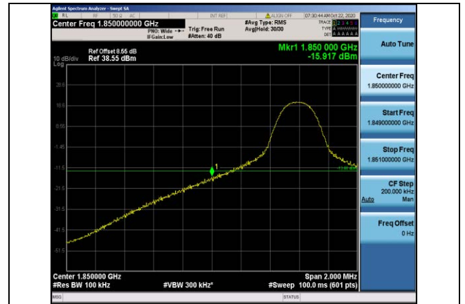
Band2-10MHz-QPSK-18650-1RB#0
