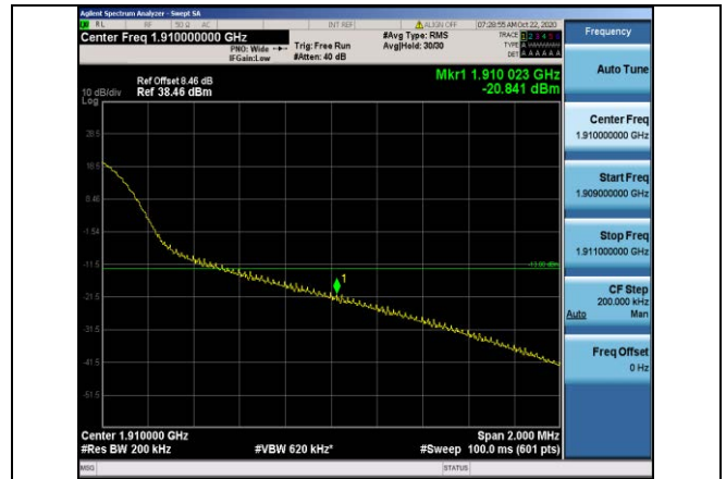
Band2-20MHz-QPSK-19100-1RB#99
