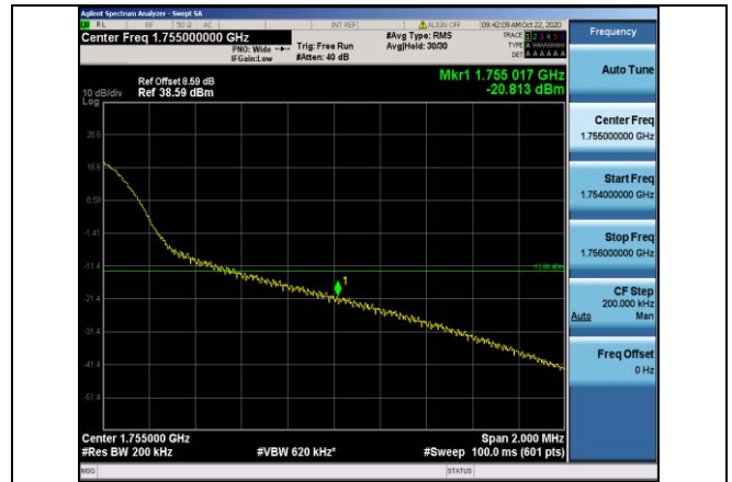
Band4-20MHz-QPSK-20300-1RB#99
