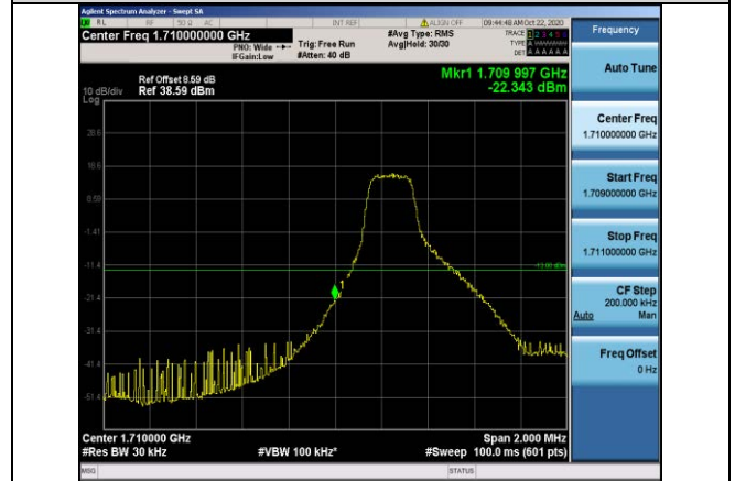
Band4-3MHz-QPSK-19965-1RB#0
