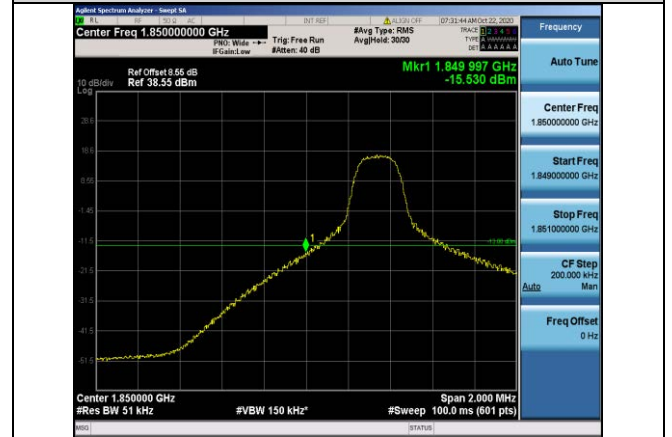
Band2-5MHz-16QAM-18625-1RB#0
