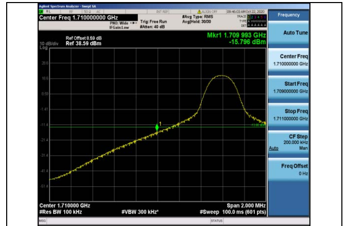
Band4-10MHz-QPSK-20000-1RB#0
