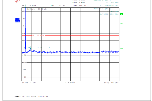
Band66-20MHz-QPSK-132072-1RB#0-Range2:1000~20000MHz--31.89-PASS
