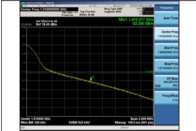
Band2-20MHz-16QAM-19100-1RB#99
